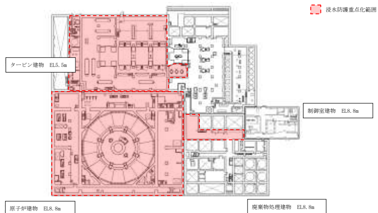
第 2.4-2 図(1) 浸水防護重点化範囲 (平面図)
