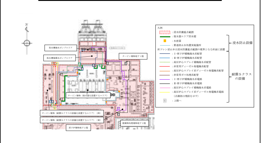
第2.4-3 図 タービン建物地下1階の復水器エリア防水壁等の浸水防止設備と耐震Sクラスの設備の位置
