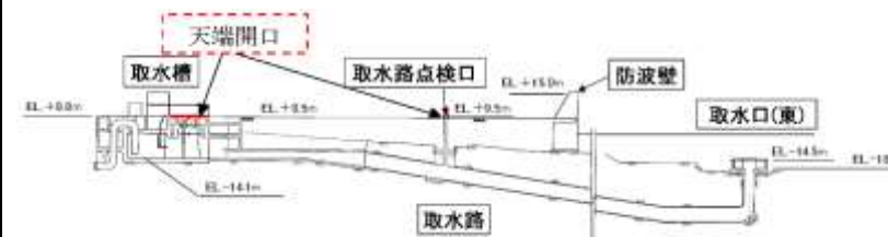
第 2.2-19 図 3号炉 取水施設の断面図
