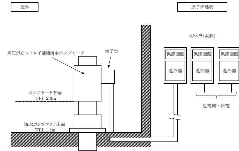
第 2.3-9 図 取水槽海水ポンプエリアに設置する設計基準対象施設の津波防護対象設備の機能喪失高さ
