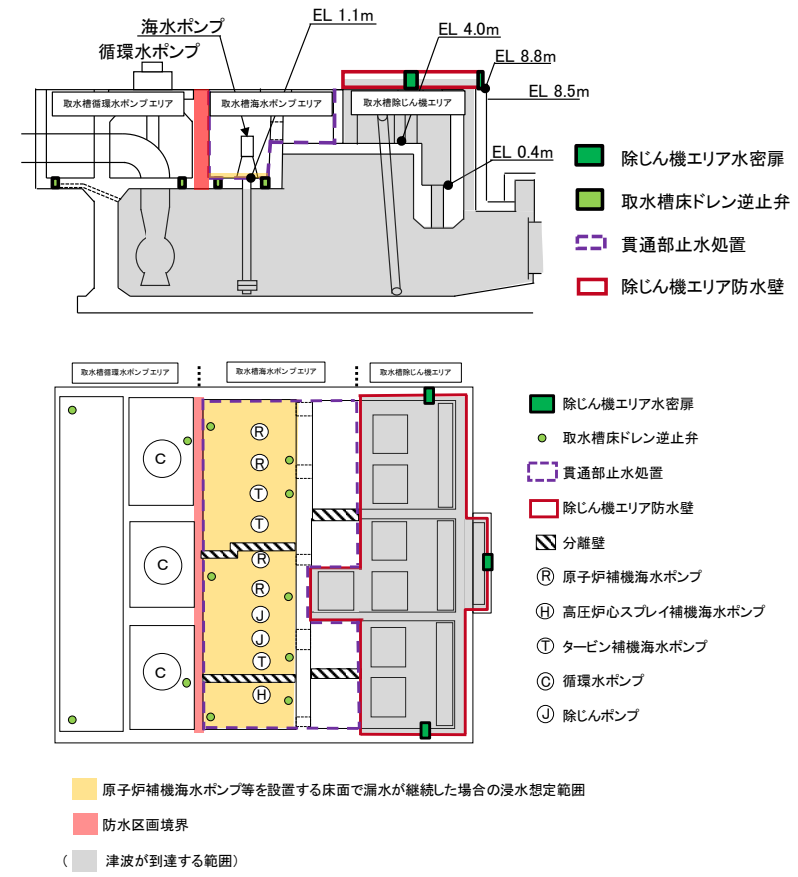
第2.3-7図 浸水想定範囲 (取水槽海水ポンプエリア) に対する防水区画化範囲
