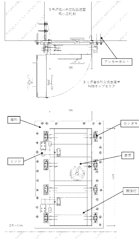
第10.6-8図 水密扉概念図
