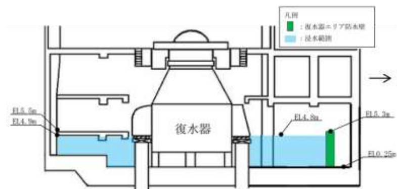
(A-A 断面)
