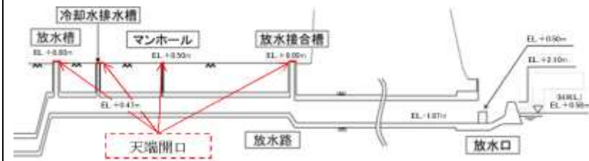
第 2.2-24 図 1号炉 放水施設の断面図
