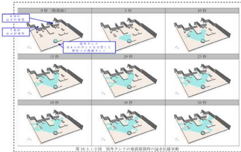
第10.1.1-2図 屋外タンクの地震損傷時の漏水伝播挙動
