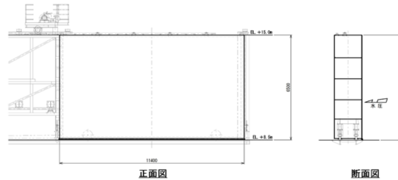
第4.1-7図 防波壁通路防波扉構造例
