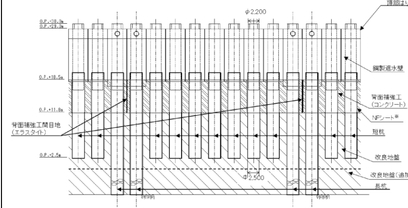
(a) 正面図
