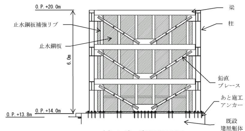
(c) A-A' 防潮壁正面図
