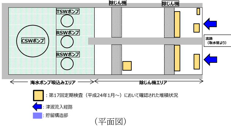
第2.5-3図 取水槽点検 (C水路) における堆積物確認結果
