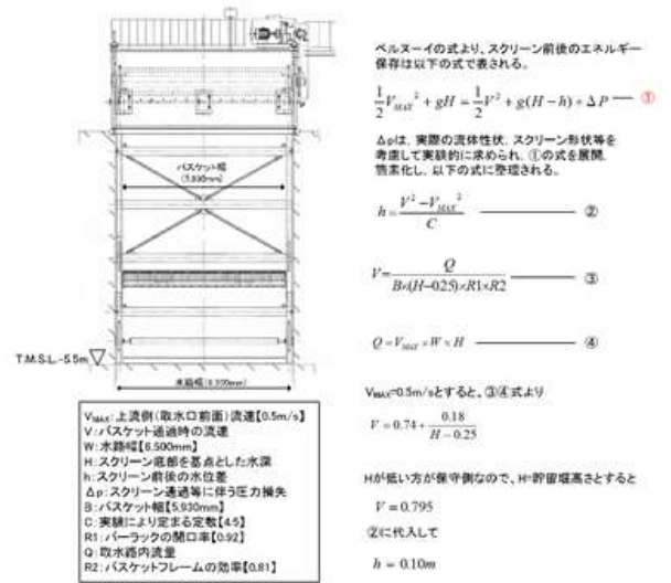
バー回転式スクリーン
