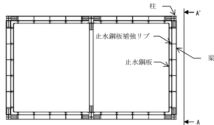
(b) 防潮壁平面図
