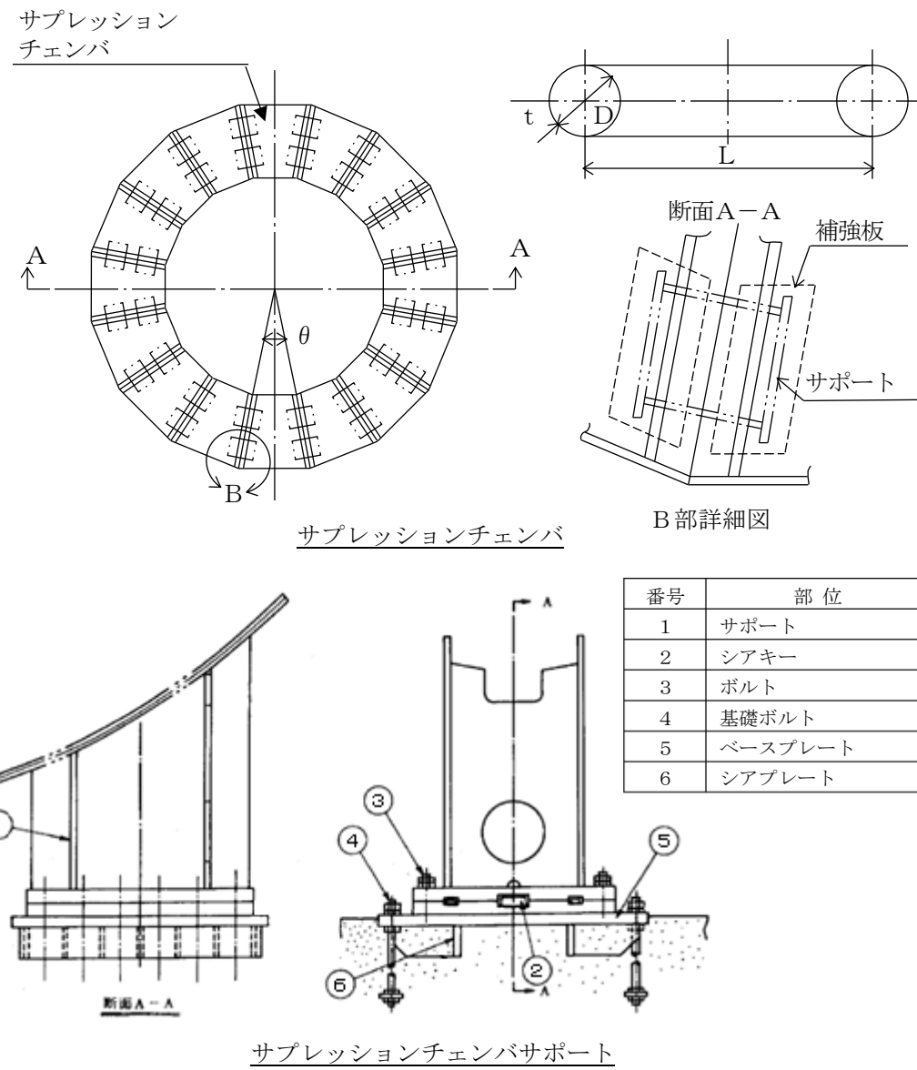
第 2.1-2 図 サプレッションチェンバ, サプレッションチェンバサポート概要図
