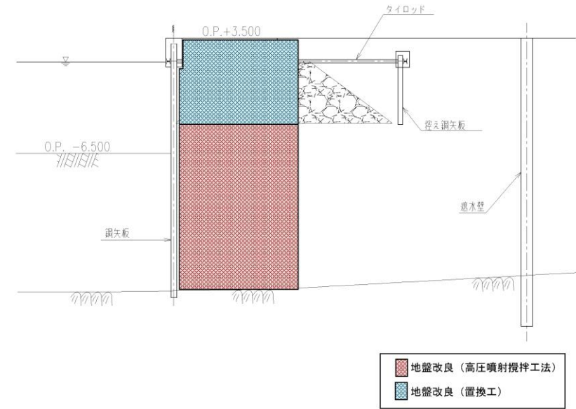
添付6-9図 前面護岸の断面図 (B-B断面)
