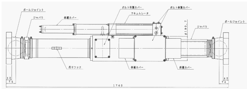
A-A オイルダンパー詳細図 (単位: mm)
