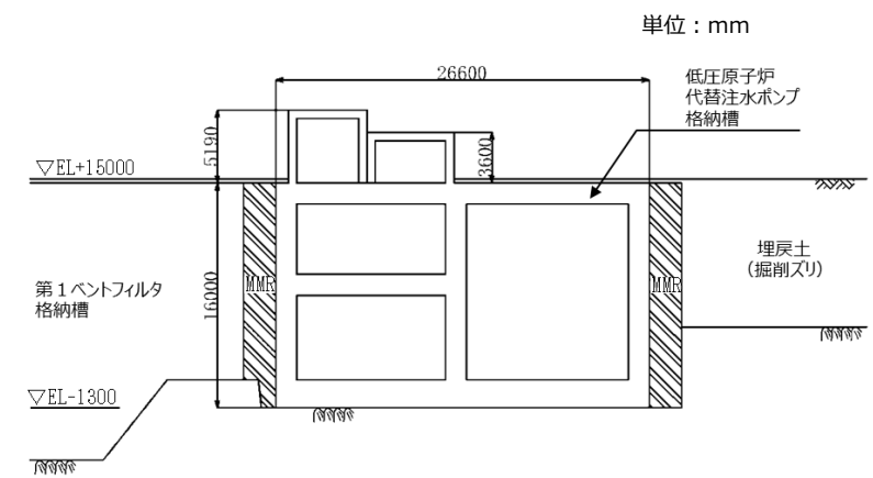
第6-2-4-3図 低圧原子炉代替注水ポンプ格納槽 縦断面図 (③断面)
