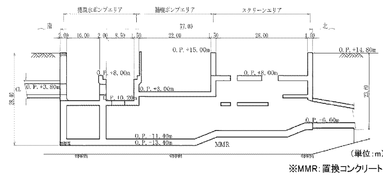
第II.1.2-2 図 海水ポンプ室断面図 (A-A 断面)
