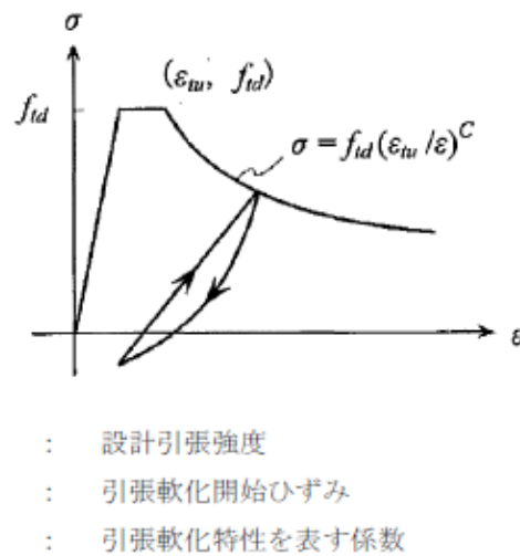
第 I. 2. 2-6 図 引張応力下における鉄筋とコンクリートの付着効果を考慮した応力-ひずみ関係
