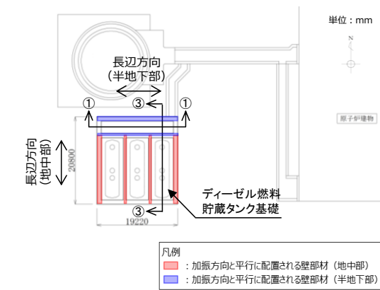
第6-2-3-1図 ディーゼル燃料貯蔵タンク基礎 配置図
