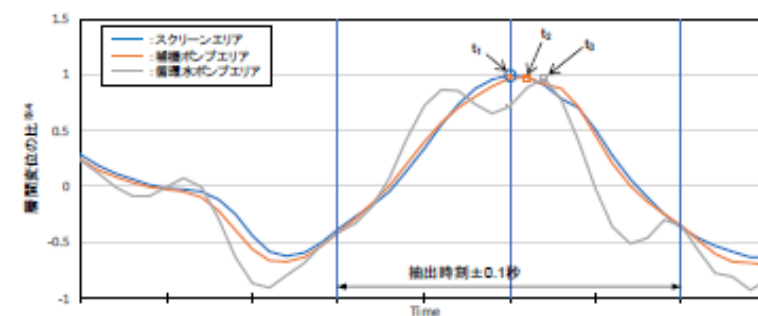
※4：最大層間変位と各時刻の層間変位の比（最大層間変位のととき1となる）。
