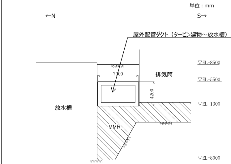
第6-2-8-5図 屋外配管ダクト (タービン建物～放水槽) 断面図 (③-③断面)
