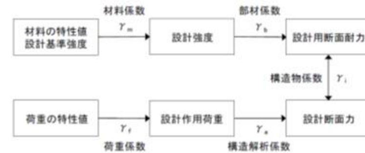
第5-2-5図 安全係数の考え方
