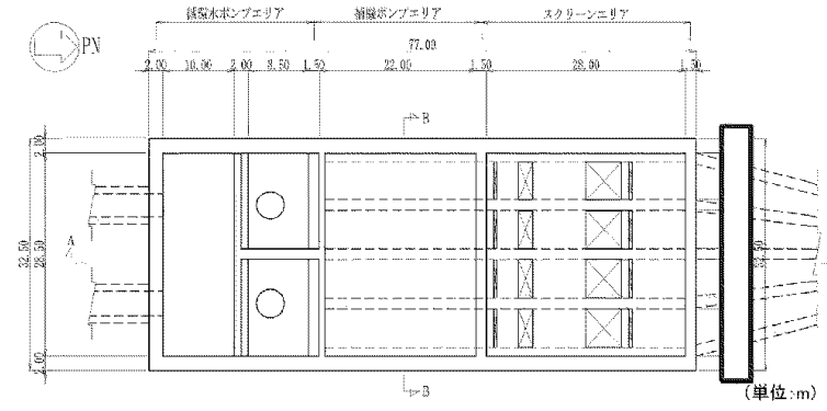
第II.1.2-1 図 海水ポンプ室平面図
