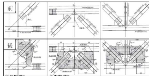
主トラス：補強前後
