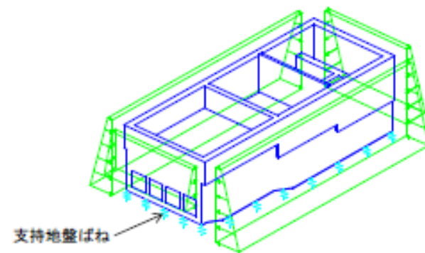
第II.3.3-1 図 静止土圧荷重イメージ
