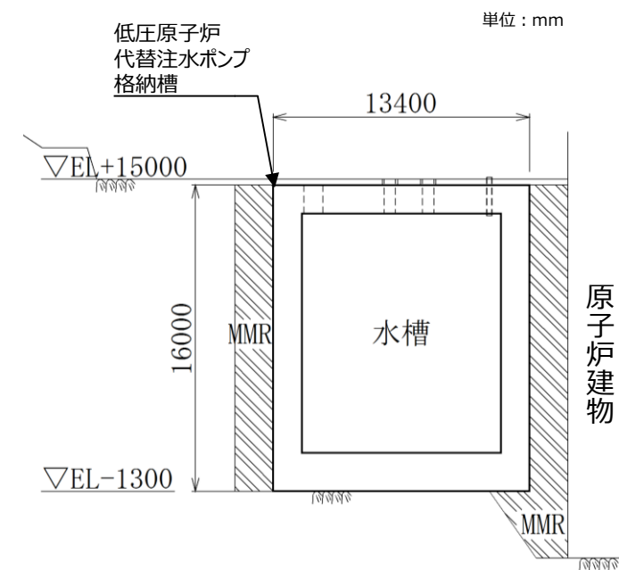
第6-2-4-5図 低圧原子炉代替注水ポンプ格納槽 断面図 (②) -②断面-
