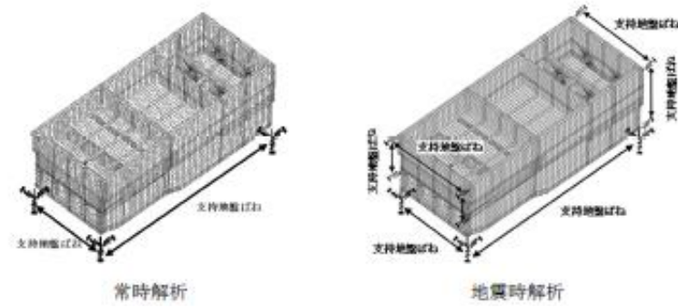
第II.3.2-1 図 三次元モデル
