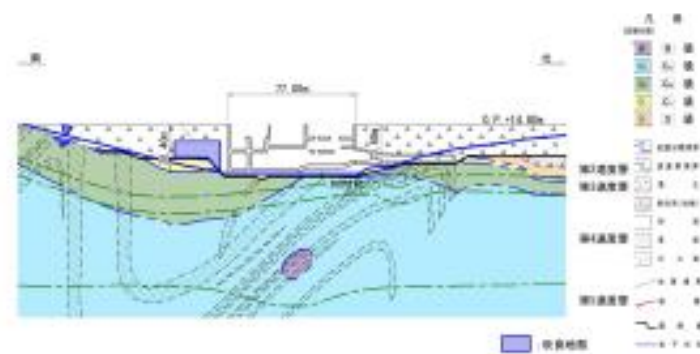
第II. 3. 4-4 図 改良範囲断面図 (B-B' 断面)
