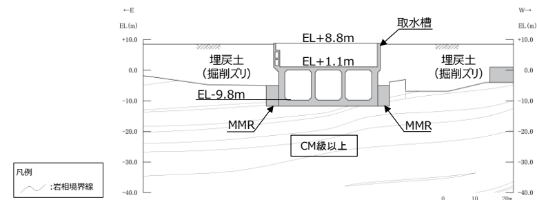
第6-2-2-12図 取水槽 岩級断面図 (②-②断面)
