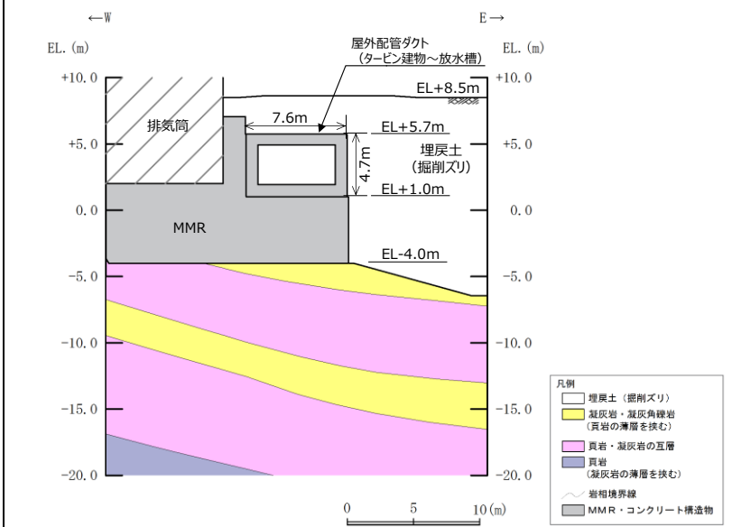
第6-2-8-6図 屋外配管ダクト (タービン建物～放水槽) 地質断面図 (②-②断面)
