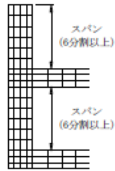
第Ⅱ. 6. 3-3 図 スパン分割の概略図
