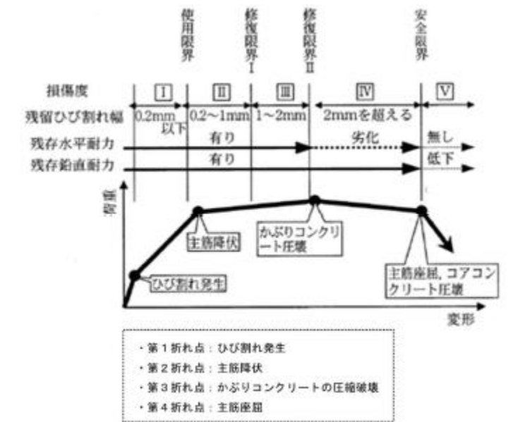
第 I. 2. 1-3 図 曲げ降伏先行型の部材の復元力特性と限界状態 (損傷度) の関係の概念図 (建築学会に加筆)
