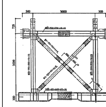
第2.5.2-2 図 試験体の概要 ((1)より引用)
