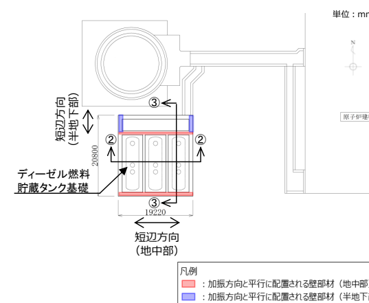
第6-2-3-2図 ディーゼル燃料貯蔵タンク基礎 平面図
