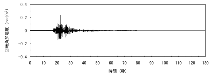
(e) 東西方向 (回転)
