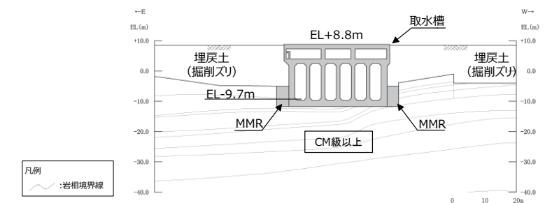
第6-2-2-13図 取水槽 岩級断面図 (③-③断面)
