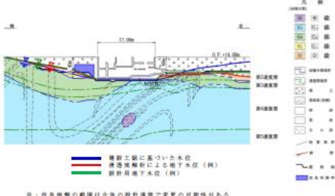
第3.1-9図 海水ポンプ室地質断面図 (横断)
