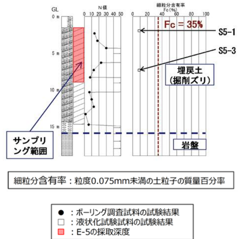
E-5 地点のボーリング調査試料及び液状化試験試料の試験結果 第3-1-11 図 液状化試験試料採取位置の基本物性 (E-5の埋戻土(掘削ズリ))
