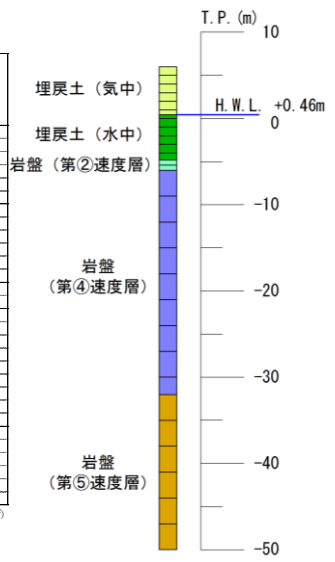
(e) 基本物性 (比較地点⑤)
