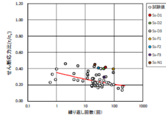
(a) 旧表土
