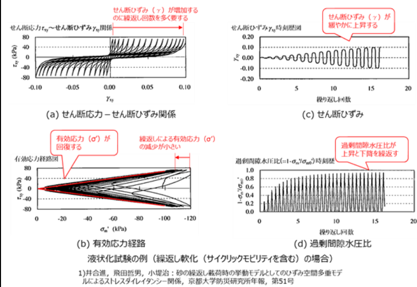
第3-2-6 図 密な砂の液状化試験結果
