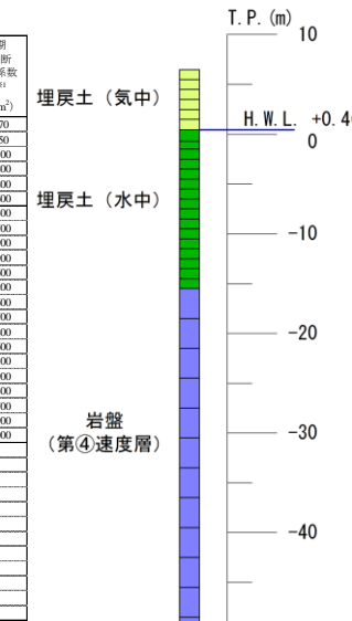
(b) 基本物性 (比較地点②)
