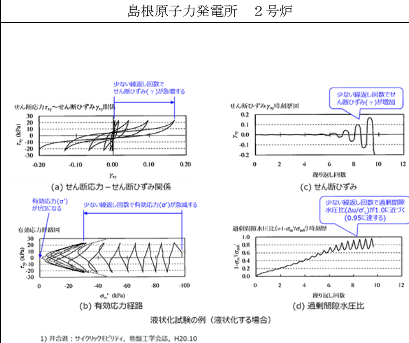
第3-2-5 図 緩い砂の液状化試験結果
