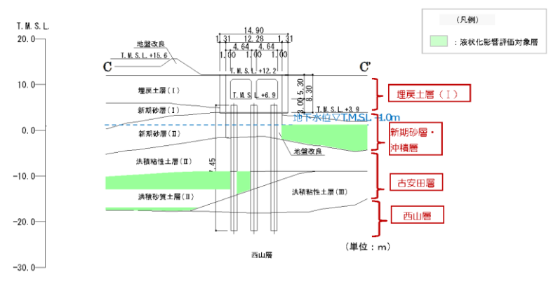
(2) 第一ガスタービン発電機基礎 (NS 断面)
