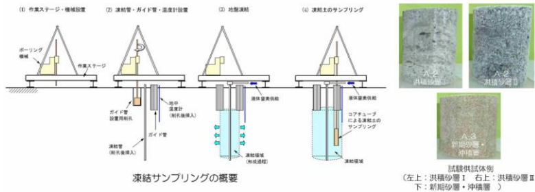
第11-4-4 図 凍結サンプリングの概要
