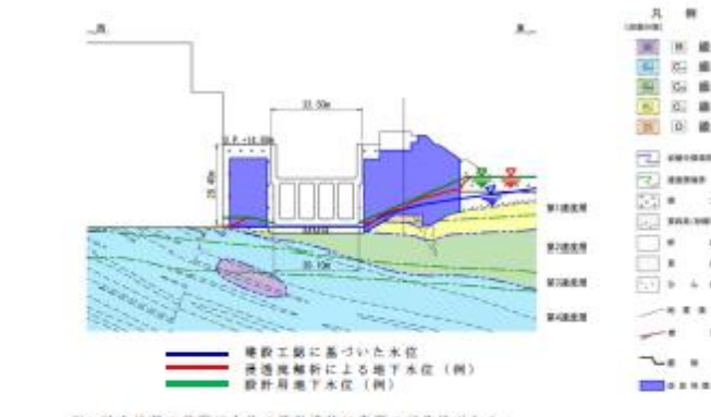
第3.1-8図 原子炉機器冷却海水配管ダクト地質断面図
