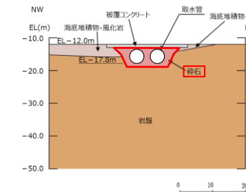
取水管
