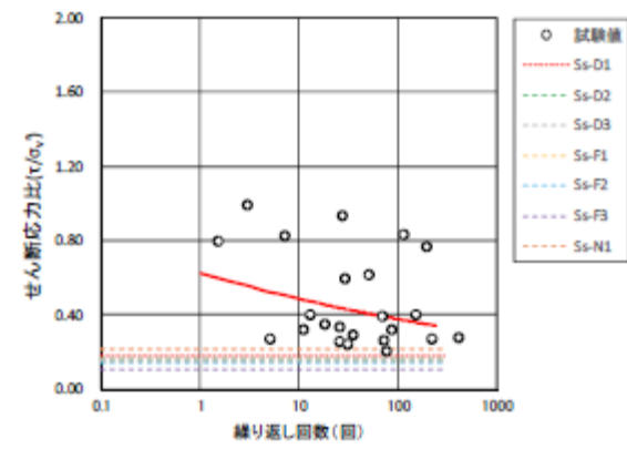
(b) 盛土
