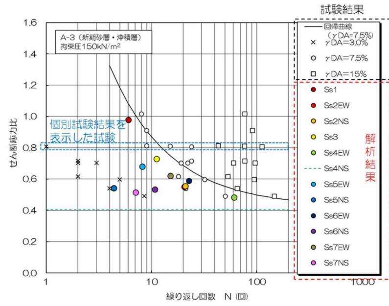
第11-6-9 図 累積損傷度理論に基づく評価結果 (A-3 地点の新时期砂層・沖積層)
