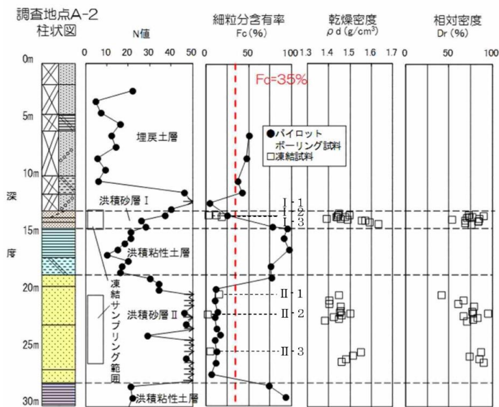
※古安田層中の砂層は、上から洪積砂層Ⅰと洪積砂層Ⅱに区分して試験を実施した。 (b) 基本物性 (N値・細粒分含有率・乾燥密度・相対密度) の深度分布
