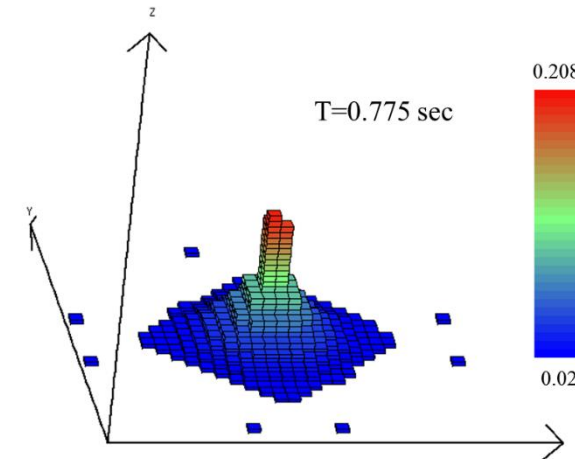
容器中心で最高高さとなった時点
