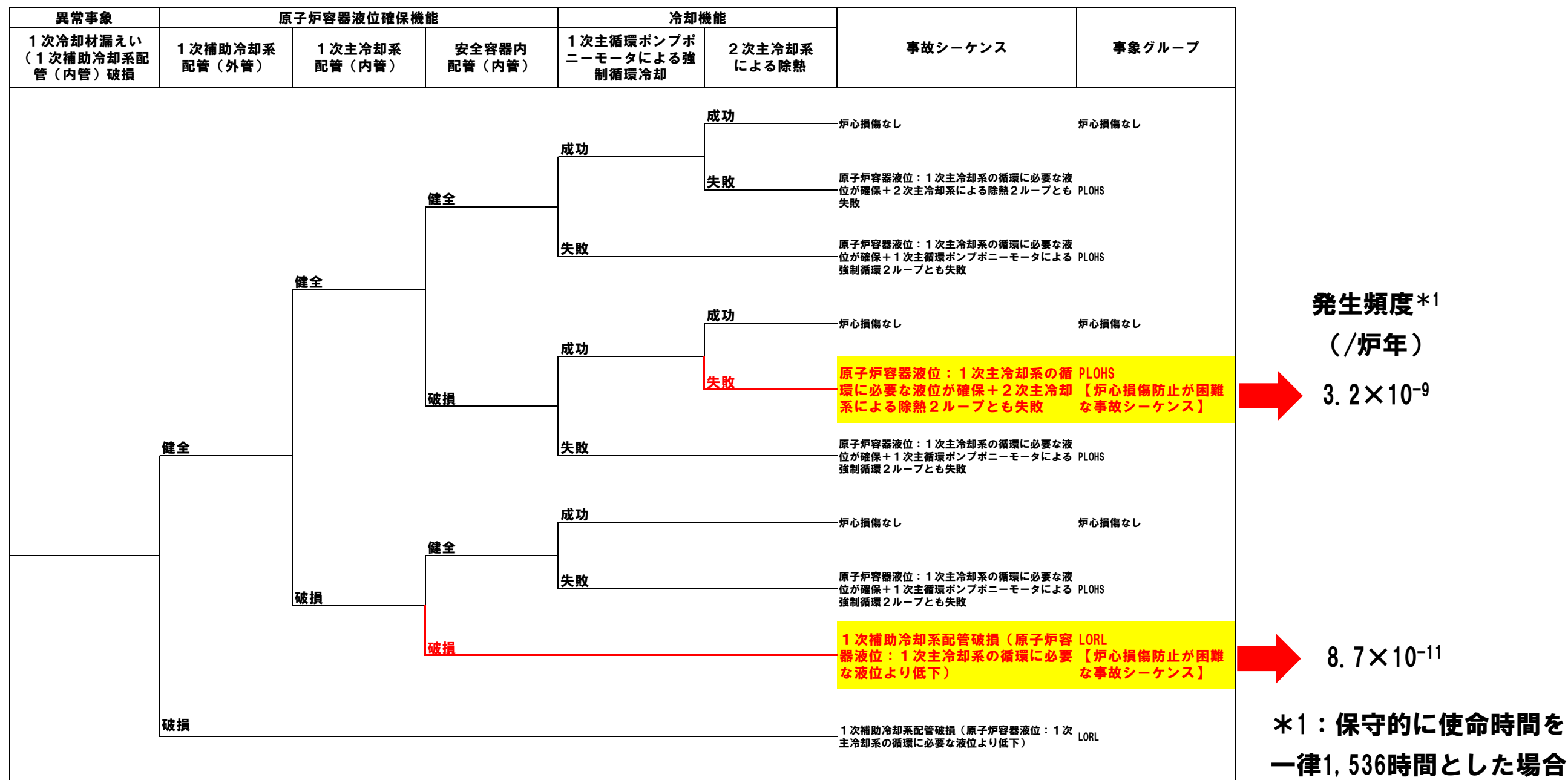
炉心損傷の防止が困難な事故シーケンスの一例
