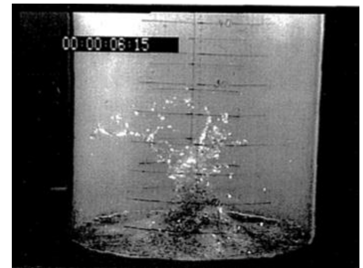
水が容器中心に集中して最高高さとなる。
