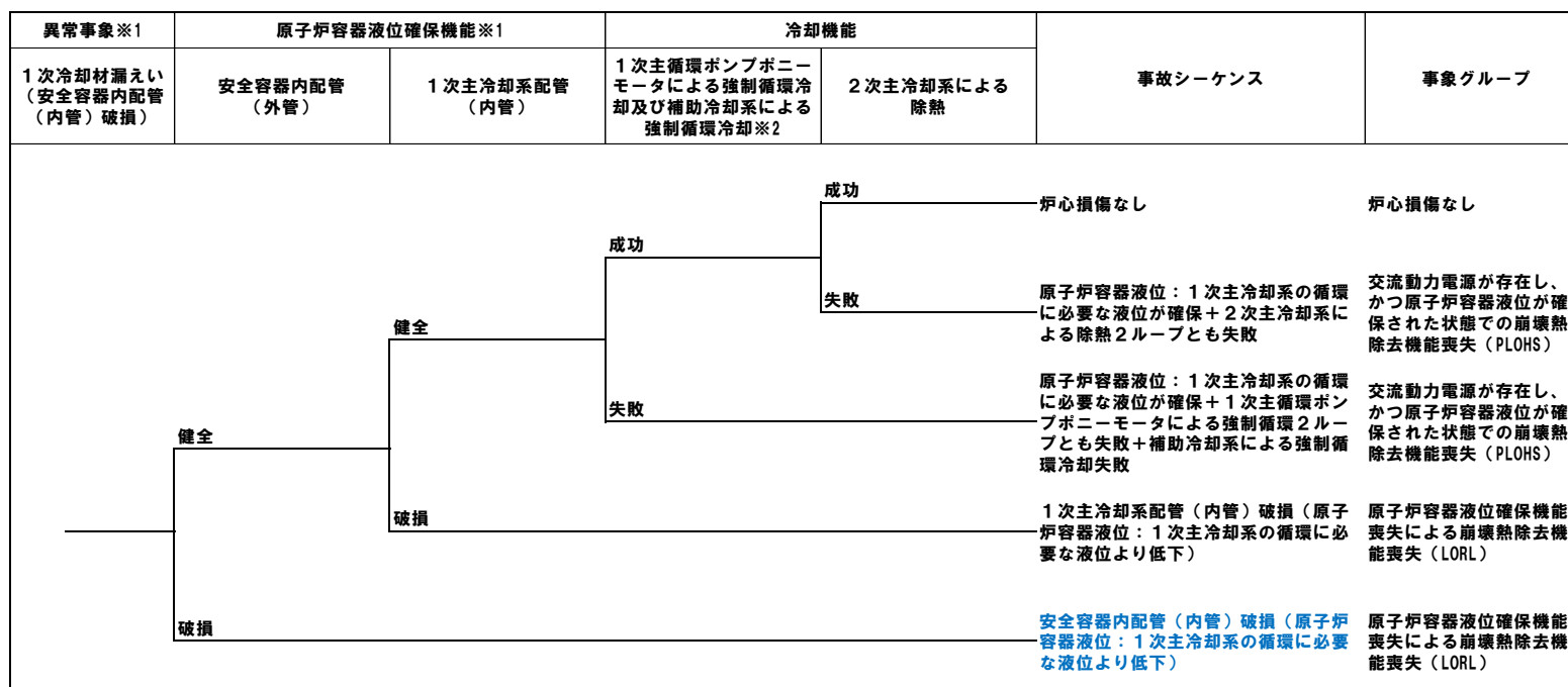
【異常事象（1次冷却材漏えい（安全容器内配管（内管）破損））のイベントツリー（冷却機能）】
