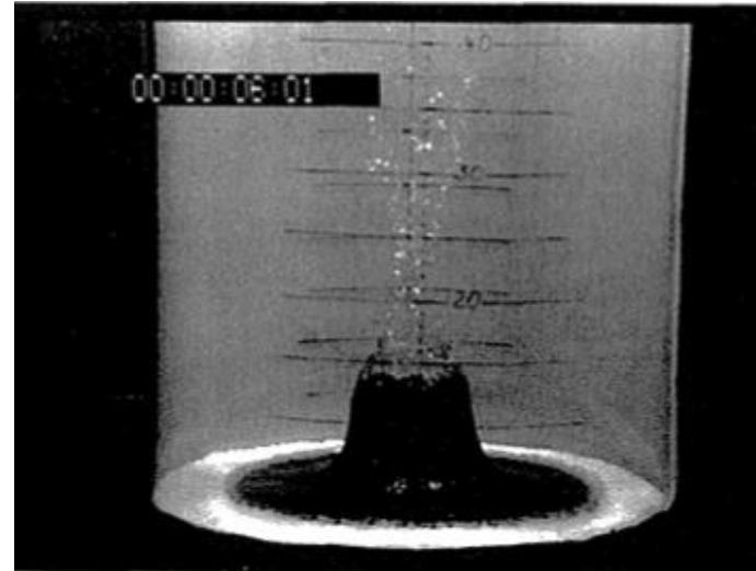
水柱の崩壊が進行する。
