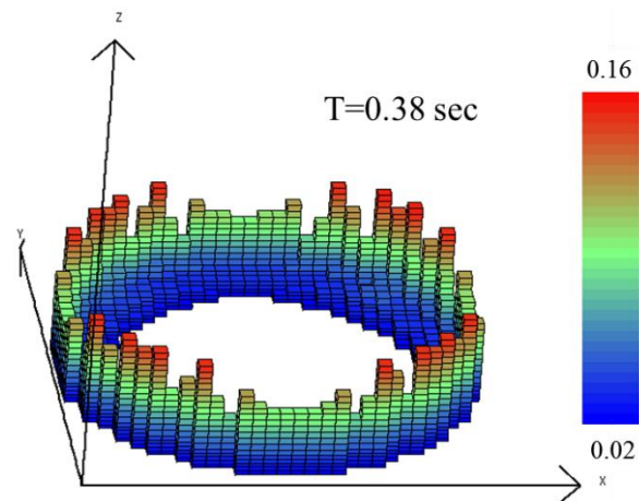
容器側面で最高高さとなった時点
