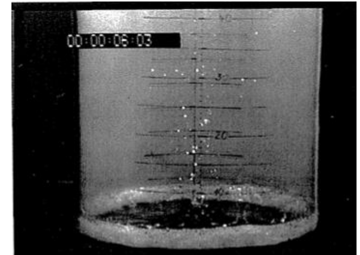
水は容器底面を広がり、側面に到達。
