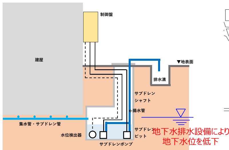
地下水排水設備の概要図
