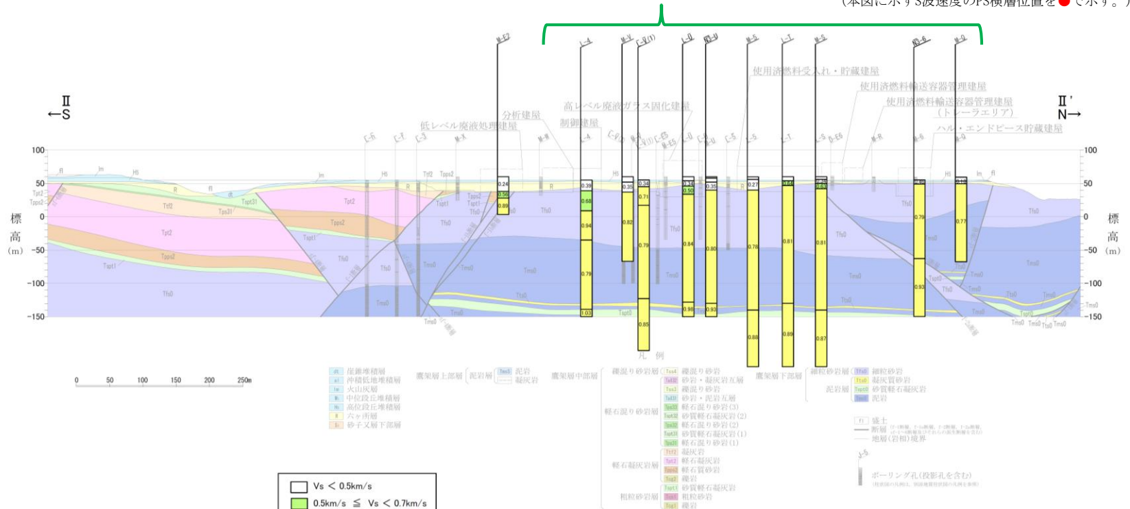
各エリア南北断面の地質断面図及びP S 検層結果 (中央地盤)
