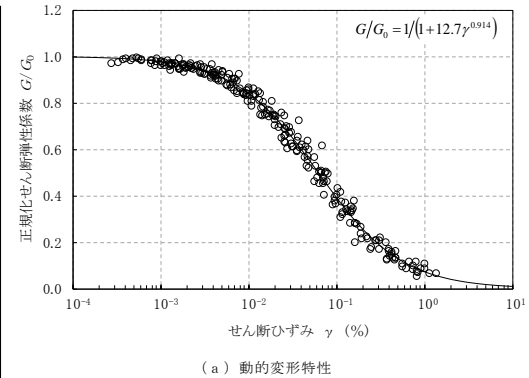
(a) 動的変形特性
