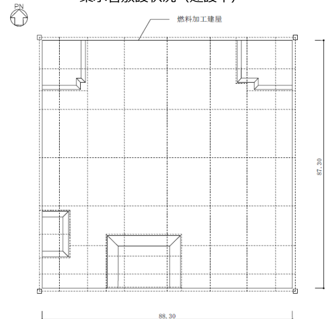
サブドレン管の敷設図 (燃料加工建屋の例)
