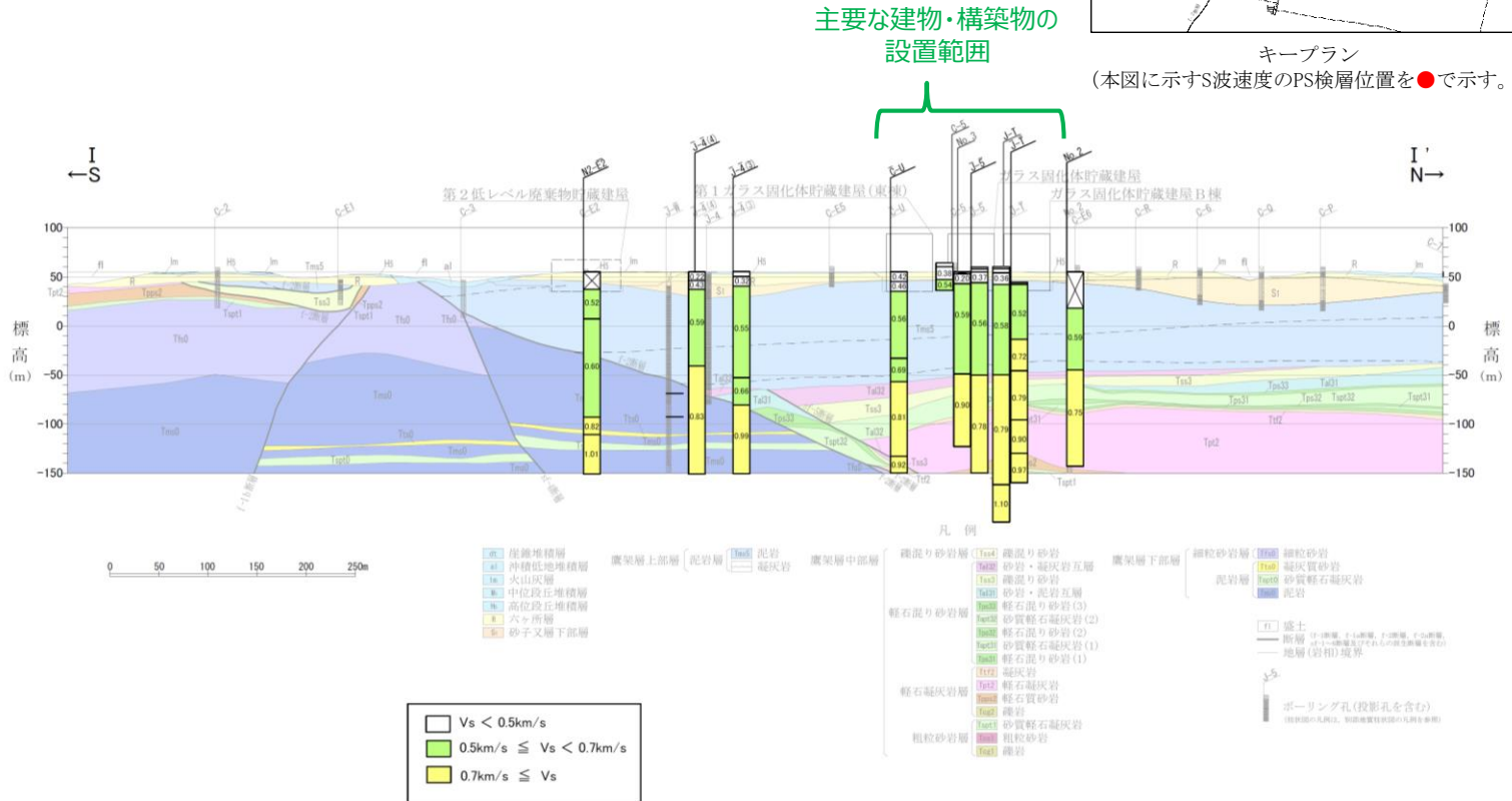
各エリア南北断面の地質断面図及びP S 検層結果 (西側地盤)
