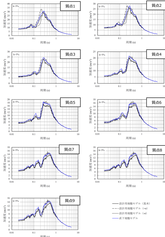
建屋床応答の比較 (床応答スペクトル) (EW方向)
