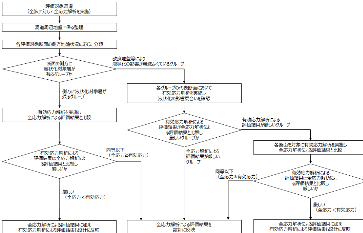
洞道の液状化評価フロー
