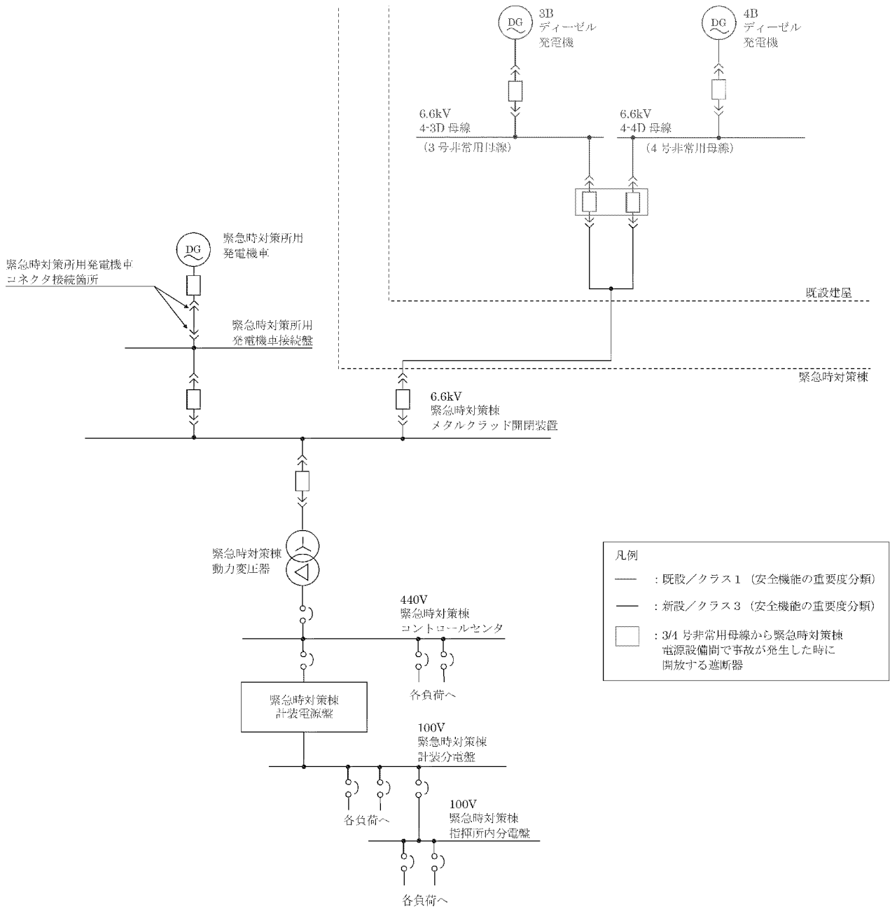
第 1 図 緊急時対策棟の電源系統図
