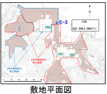
3号炉建設時の埋戻土 ボーリングNo. E-3 1.5m~17.4m
