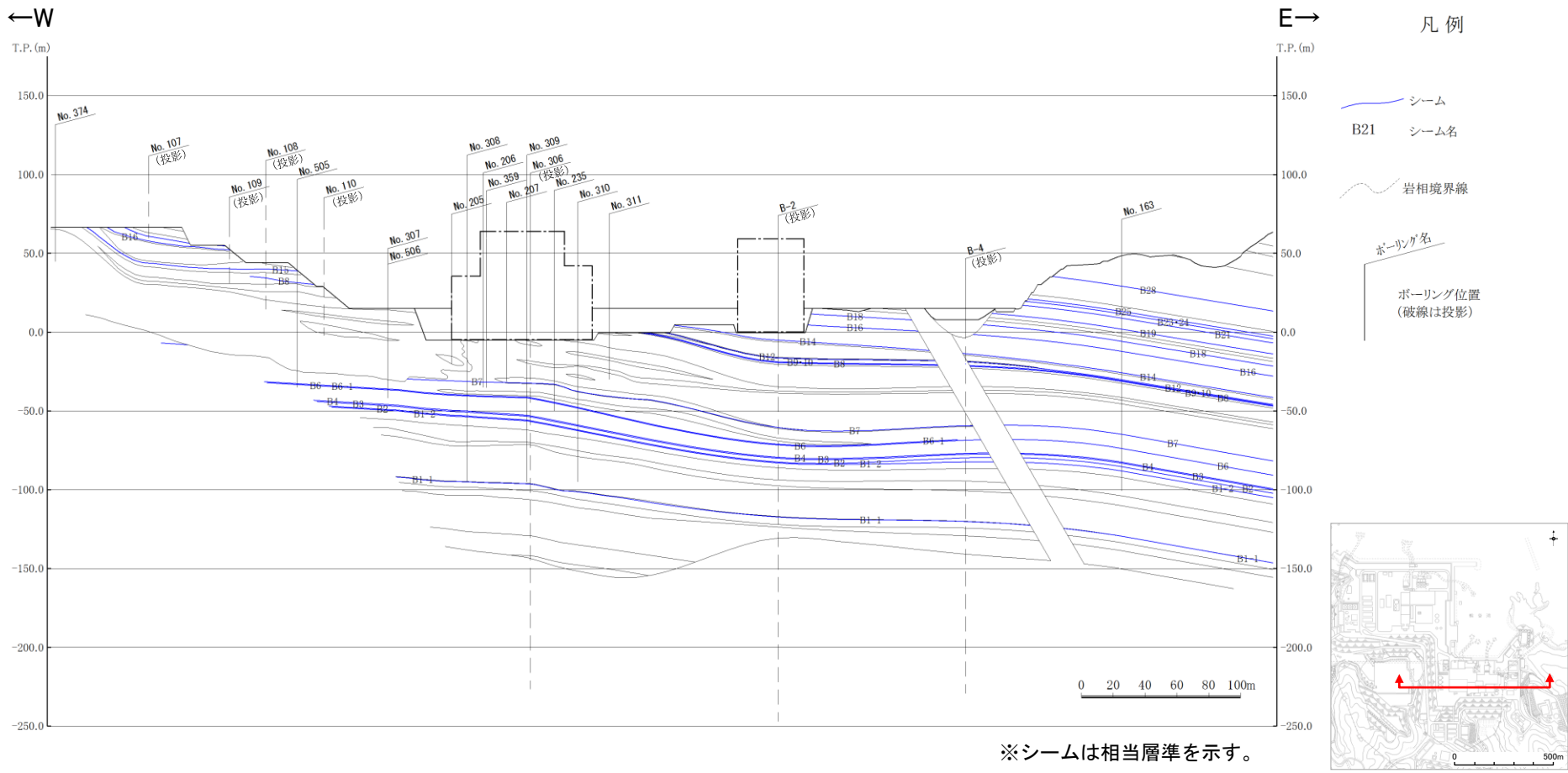
断面位置図
