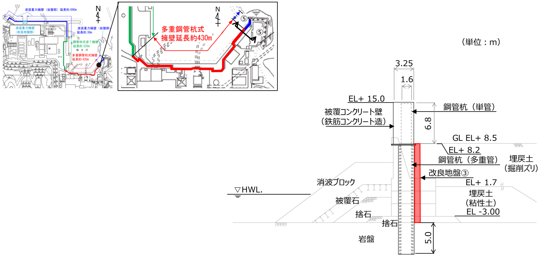
防波壁(多重鋼管杭式擁壁) 北東端部(⑤-⑤断面) 断面図
