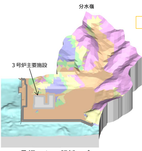
3号炉エリア 解析モデル
