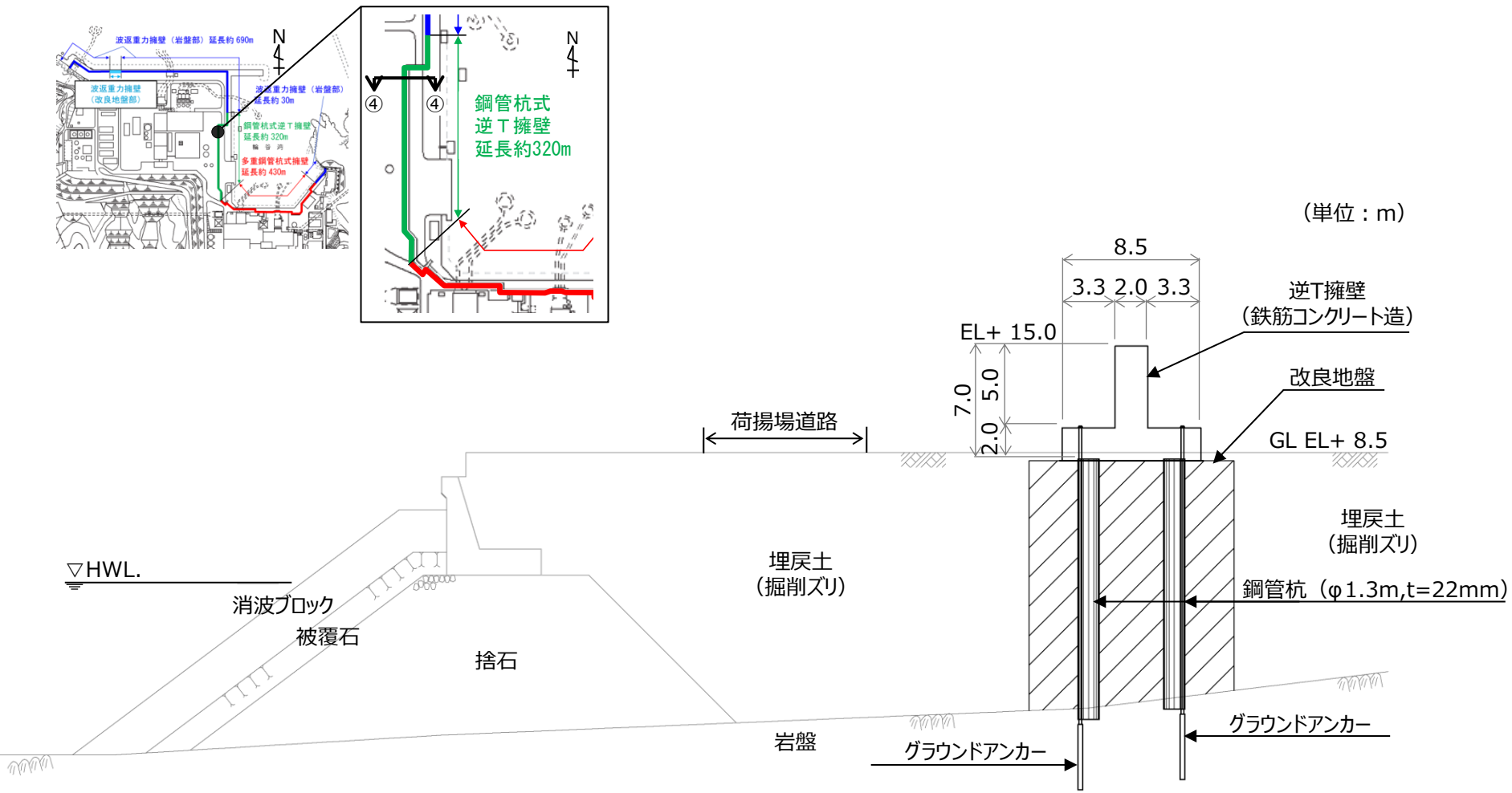
防波壁(鋼管杭式逆T擁壁)防波扉南側部(④-④断面) 断面図
