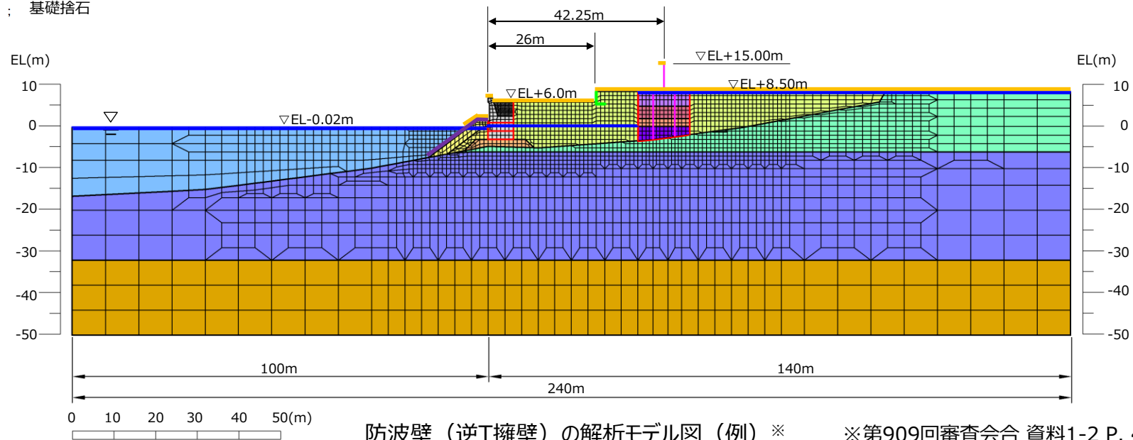
防波壁（逆T擁壁）の解析モデル図（例）※ ※第909回審査会合 資料1-2 P. 46記載
