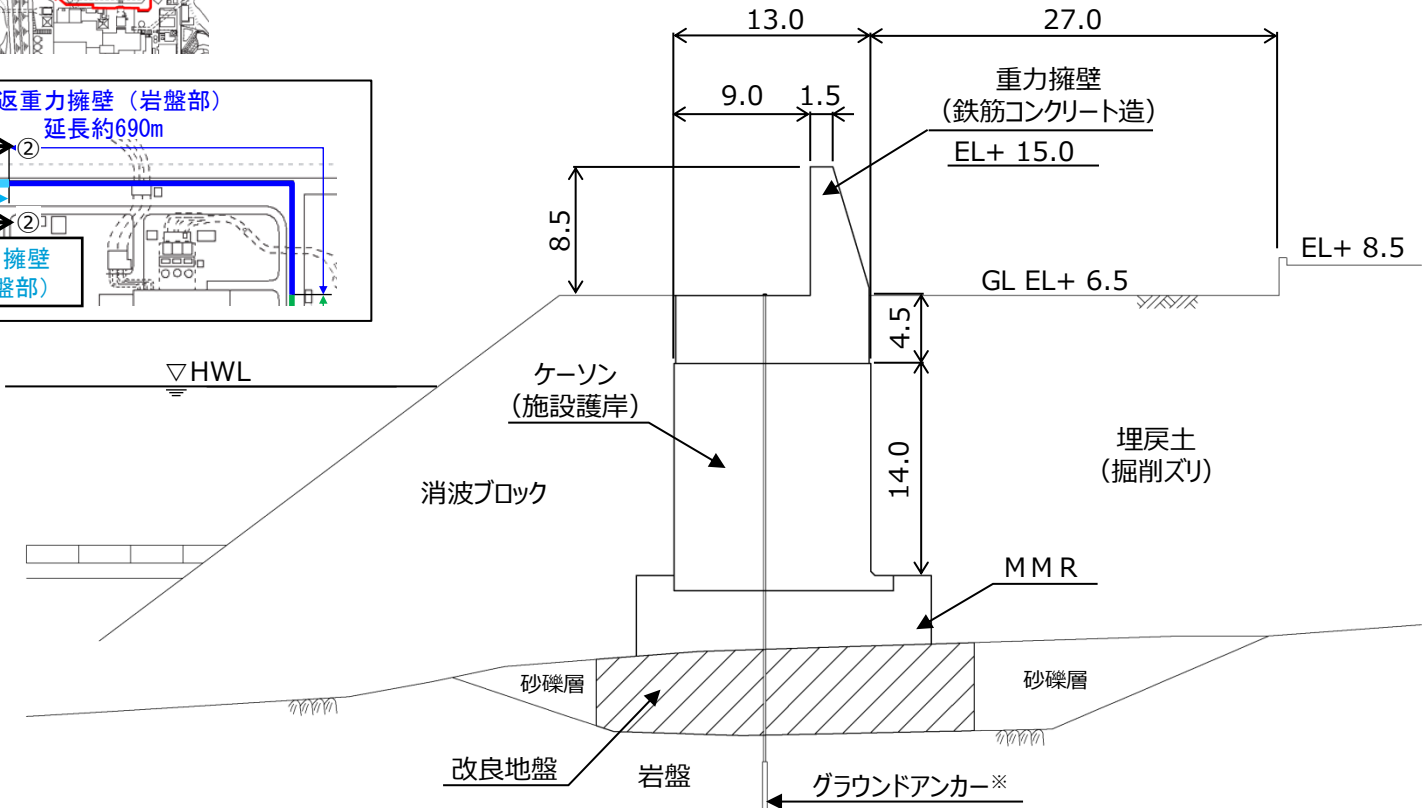
防波壁（波返重力擁壁）改良地盤部（②－②断面）断面図
