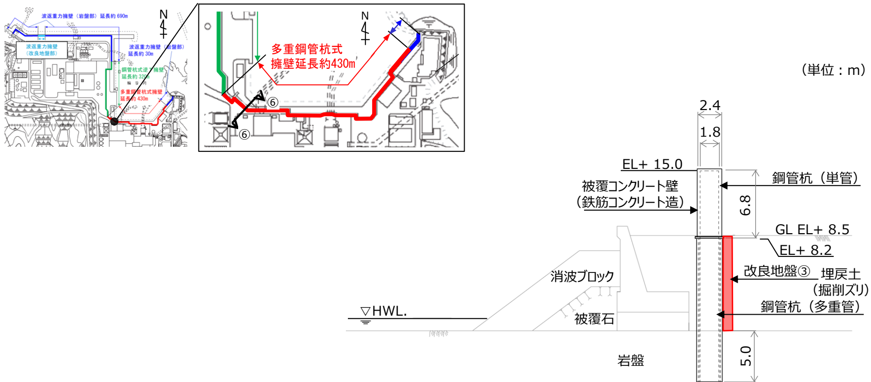
防波壁(多重鋼管杭式擁壁) 西端部(⑥-⑥断面) 断面図
