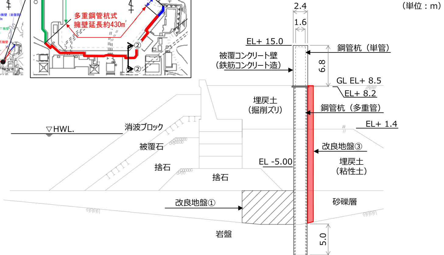
防波壁（多重鋼管杭式擁壁） 改良地盤部（②-②断面） 断面図
