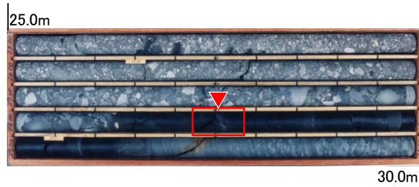
No.347コア写真 (GL-25.00～ - 30.00m)
