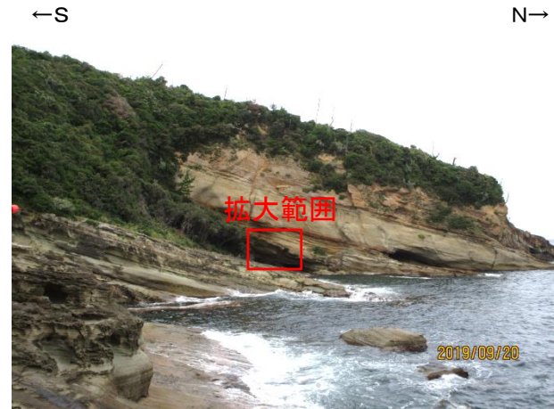
海岸露頭全景(2019年9月20日撮影)
