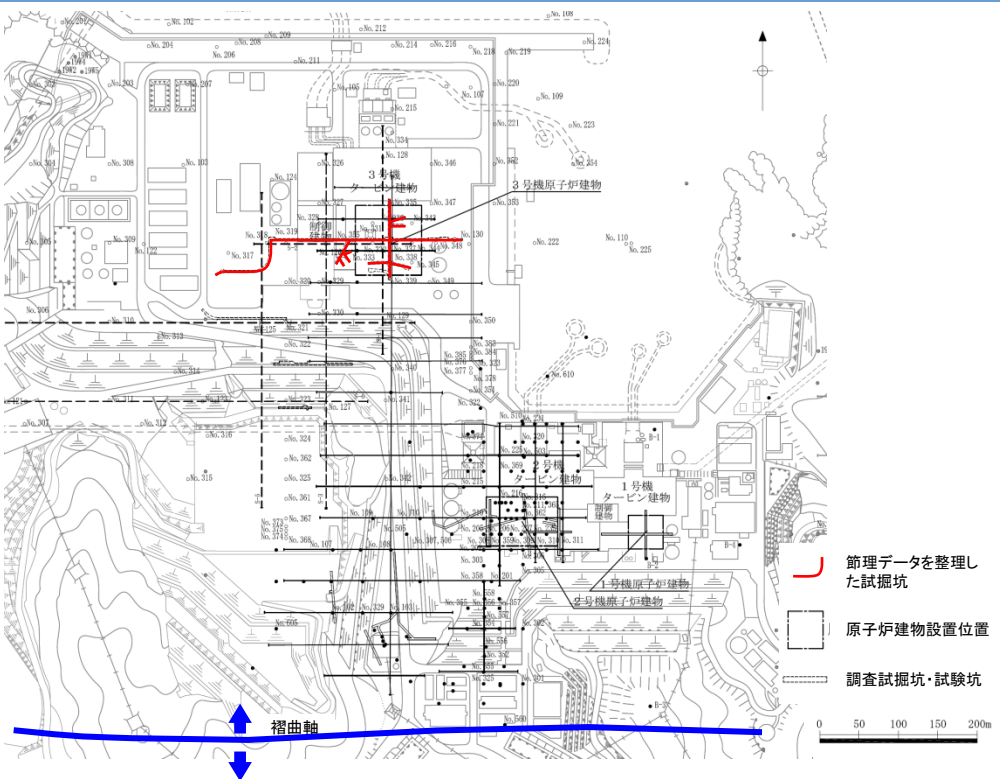
節理データを整理した試掘坑の位置図
