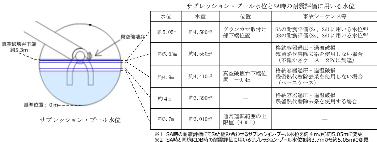
添付 8.12 図 重大事故時のサブプレッション・プール水位と耐震評価に用いる水位との関係
