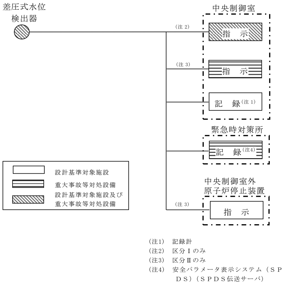
第58-6-18図 原子炉水位（広帯域）の概略構成図
