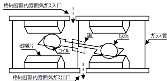
(正面図)
