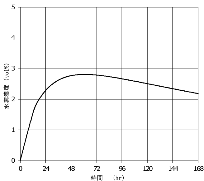
図 2. 2. 1. 2-2 原子炉建物原子炉棟 4 階の水素濃度の時間変化
