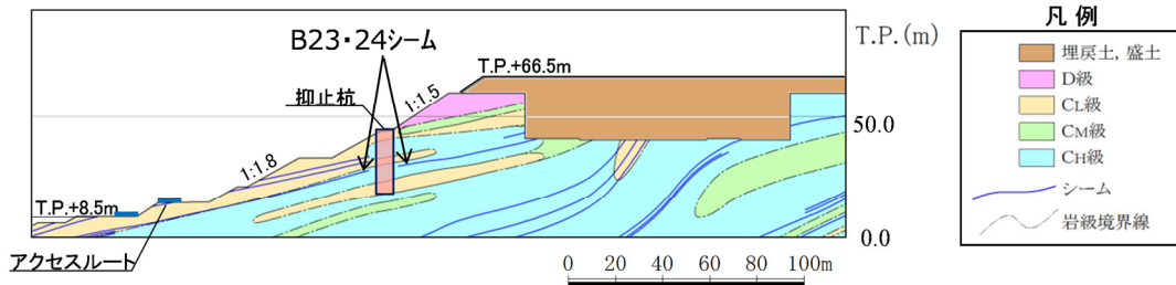
②-②' 断面
