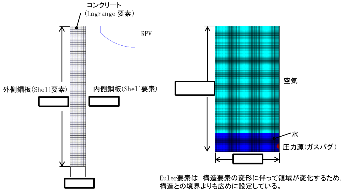
Shell要素及びLagrange要素
