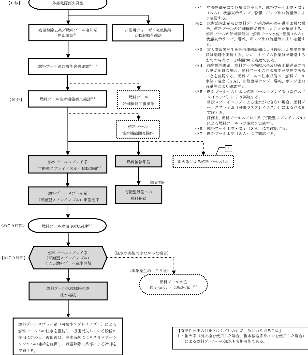
第 4.1.1-2 図 「想定事故 1」の対応手順の概要
