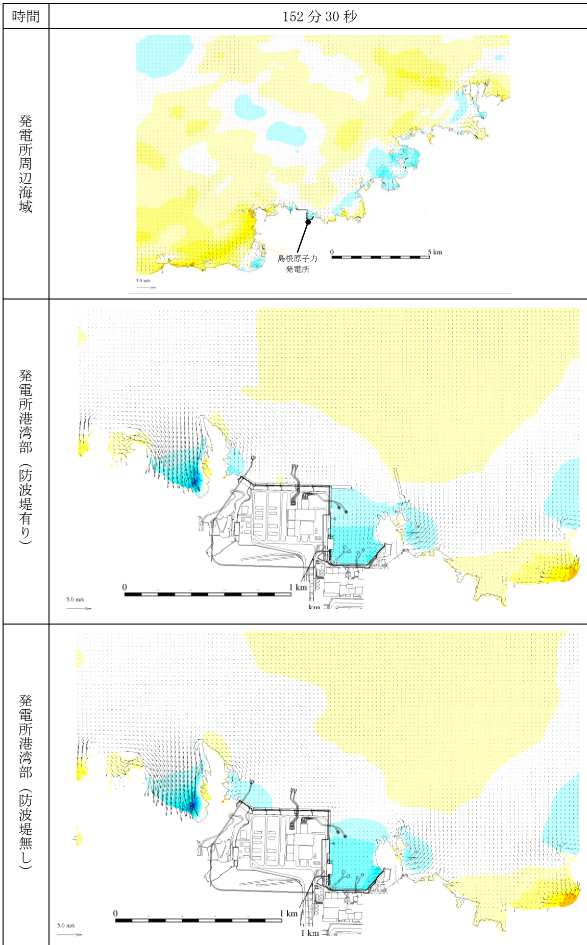
第 1 図(106) 基準津波 1 の水位変動・流向ベクトル
