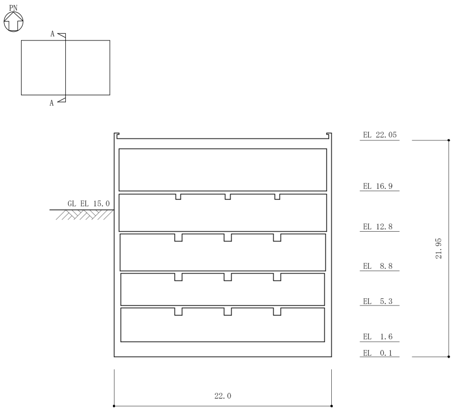
(EW断面)
