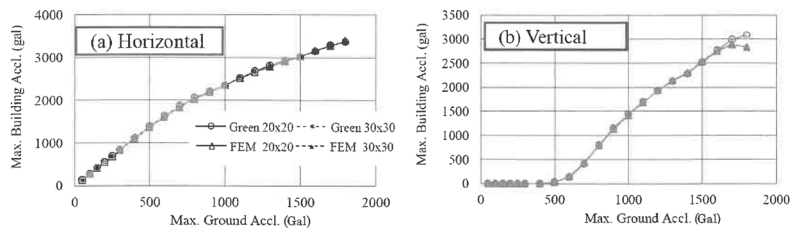
参図 3.5-16 入力加速度と建物最大応答加速度
