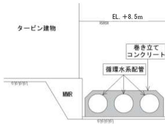
第 2.2-14-3 図 循環水排水路断面図 (①-①断面)
