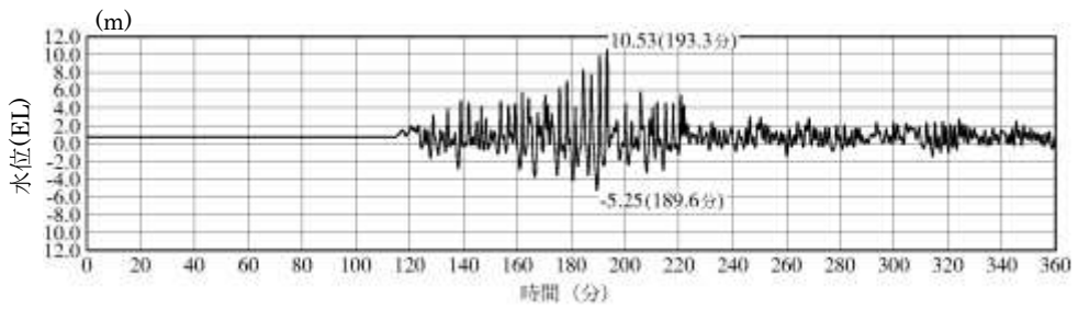
第 2.2-9 図 取水槽における入力津波の時刻歴波形（上昇側） （入力津波 1：防波堤無し）
