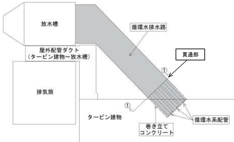
第 2.2-14-2 図 循環水排水路平面図
