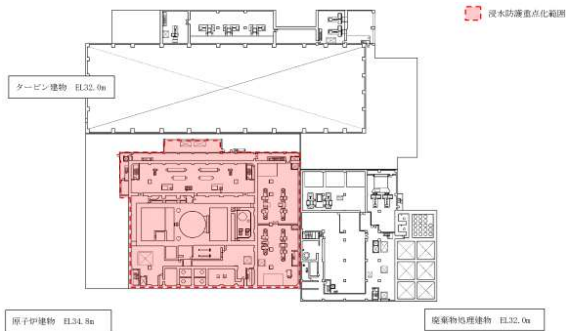
第 2.4-2 図(3) 浸水防護重点化範囲 (平面図)
