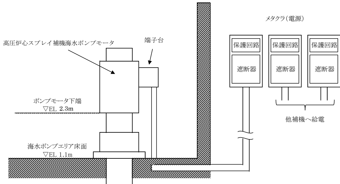
第 2.3-9 図 取水槽海水ポンプエリアに設置する設計基準対象施設の津波防護対象設備の機能喪失高さ
