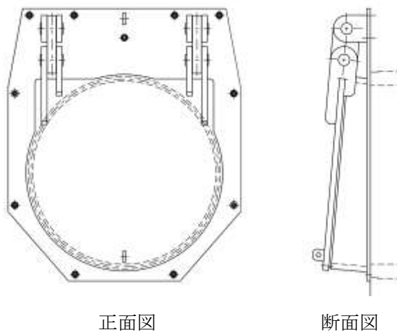
第10.5-8图 屋外排水路逆止弁概念图
