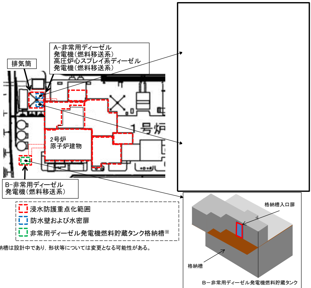
第 2.4-10 図 A-非常用ディーゼル発電機 (燃料移送系), 高压炉心スプレイ系ディーゼル発電機 (燃料移送系) 及び排気筒を設置するエリア及びB-非常用ディーゼル発電機 (燃料移送系) を設置するエリア配置図
