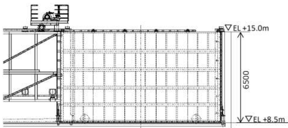
正面図
