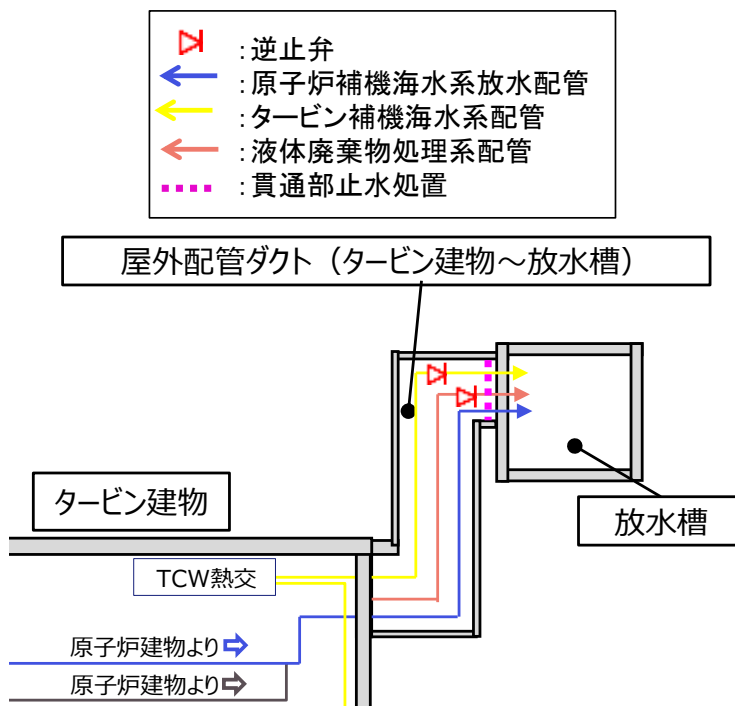
第 2.2-14-1 図 屋外配管ダクト平面図
