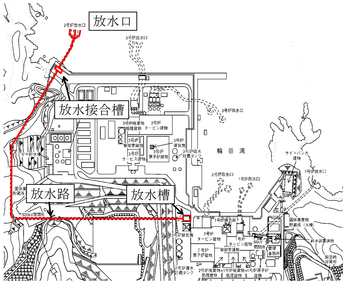
第2.2-11図 放水施設の配置図
