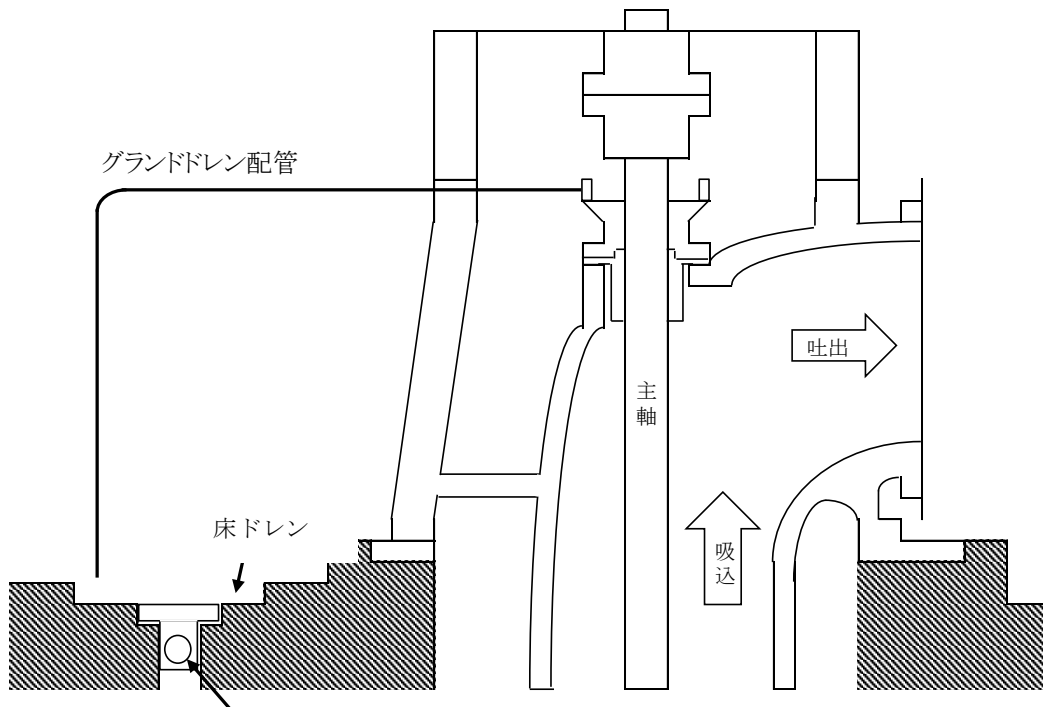
第 2.3-3 図 海水ポンプのグランドドレン配管ルート （原子炉補機海水ポンプの例）
