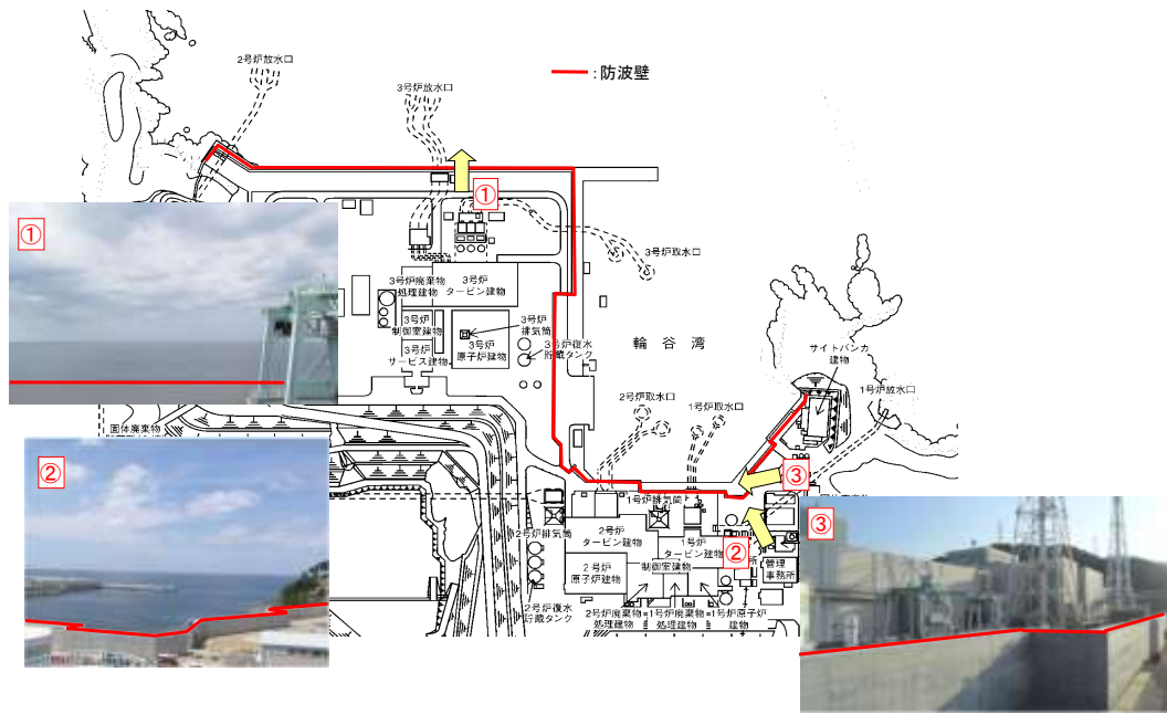
第 2.2-3 図 防波壁設置位置
