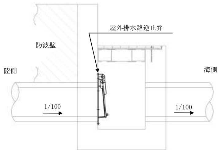
A-A断面图
