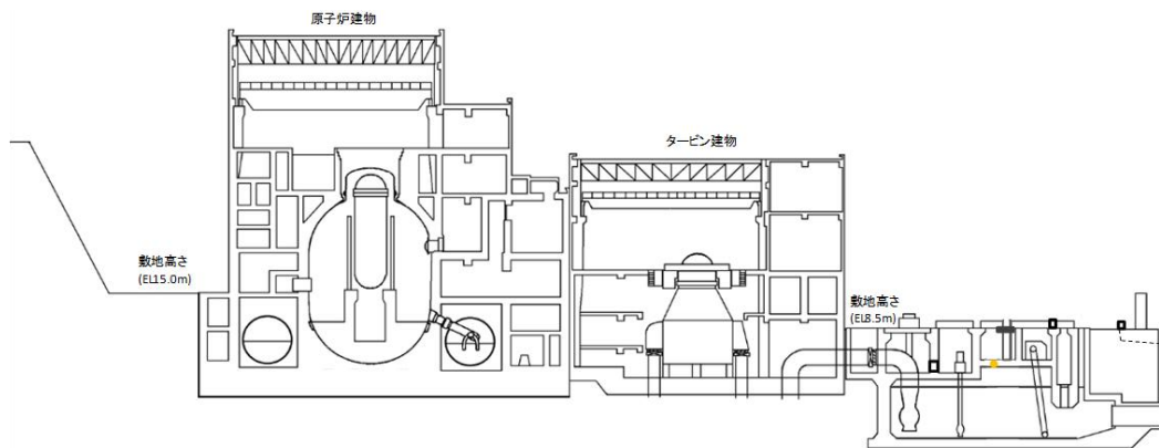
第 1.2-5 図 島根原子力発電所 主要断面図
