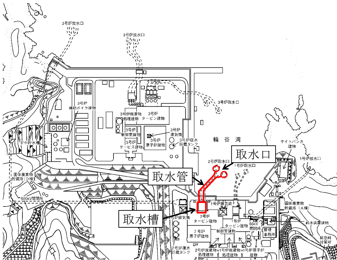
第 2.2-5 図 2号炉 取水施設の配置図
