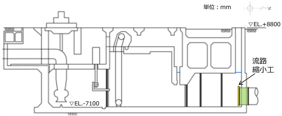
断面図
