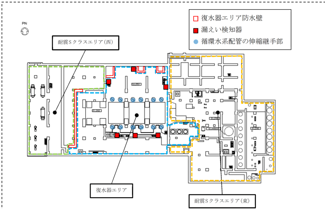
図 9-5 漏えい検知器設置箇所（タービン建物地下1階）
