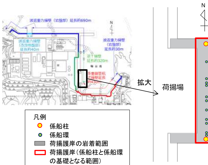
図 1 係船柱及び係船環配置図
