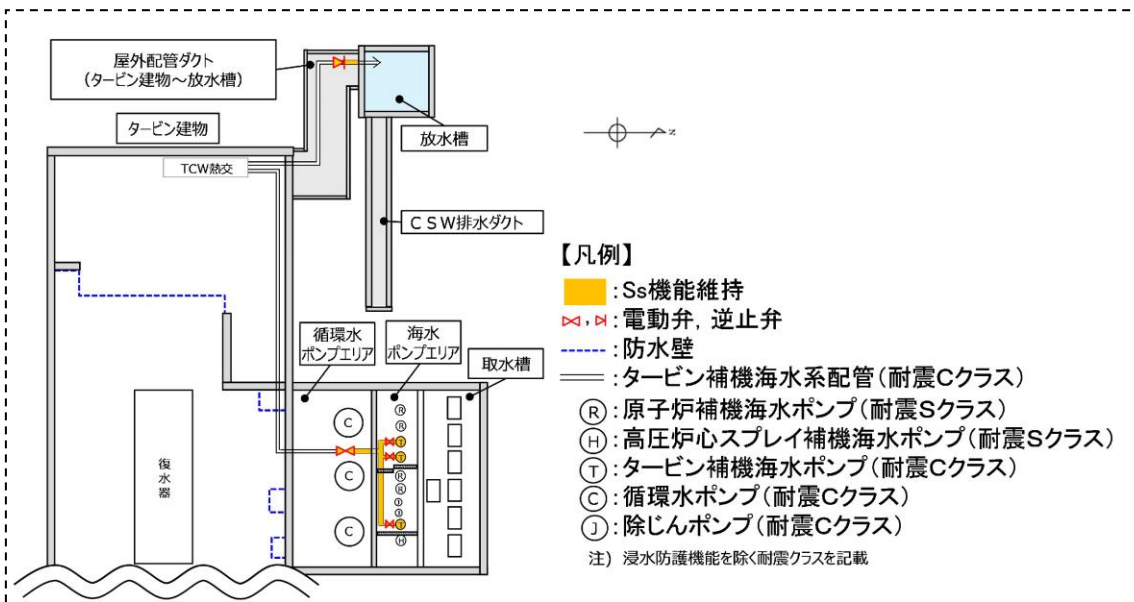
図 9-10-2 タービン補機海水系の対策概要 (平面図)
