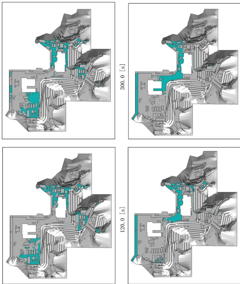
図 10-3-2 屋外タンクの溢水伝播挙動 (2/2)
