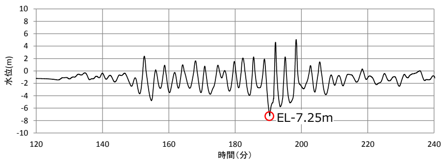
EL-7.25m=貝付着を考慮した取水管下端高さEL-7.25m 2号炉取水管端部（東）（循環水ポンプ運転時）
