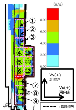
第 10 図 基準津波 1 (防波堤無し) における荷揚場周辺の 最大浸水深分布及び流速
