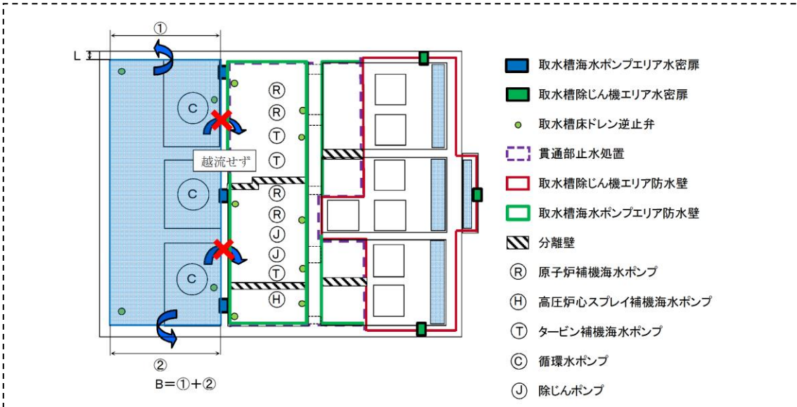
図 9-12 取水槽海水ポンプエリア平面図 (循環水系配管破損時)
