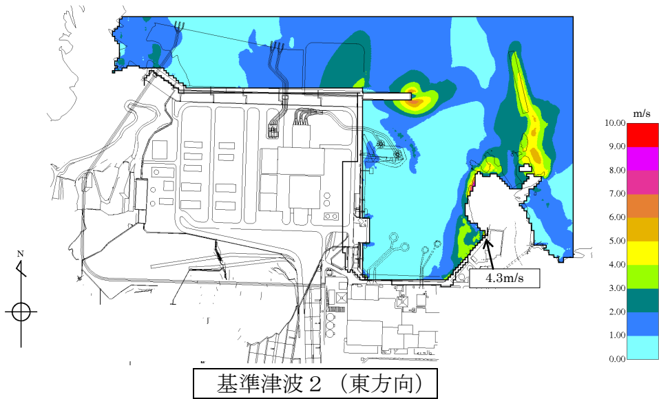
第4図 基準津波 2 最大流速分布 (2 / 2)
