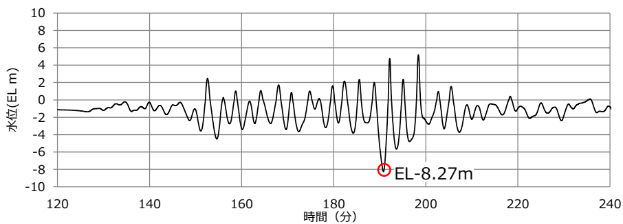
EL-8.27m(初期条件として地殻変動を考慮) > 許容高さEL-8.32m 2号炉取水槽（循環水ポンプ運転時）
