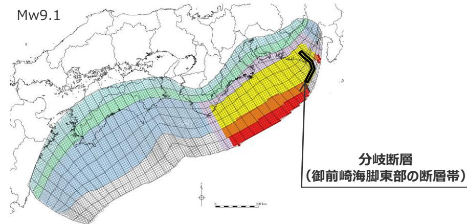
検討波源モデルB-2 (プレート境界面浅部・御前崎海脚東部の断層帯) の大すべり域の位置を西へ10kmとしたケース
