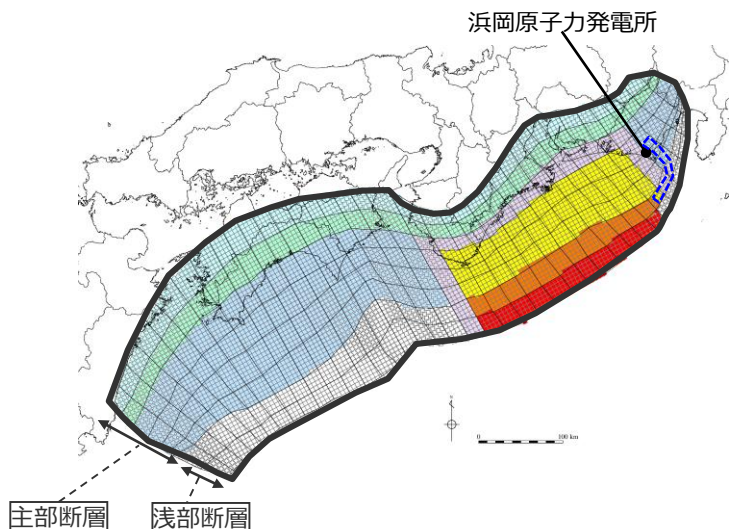
検討波源モデルB-2 (プレート境界面浅部・御前崎海脚東部の断層帯) の大すべり域の位置を西へ60kmとしたケース
