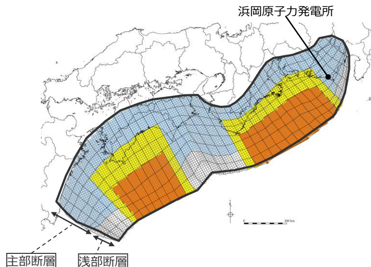
検討波源モデルC (土木学会(2016)手法モデル) の大すべり域の位置を西へ60kmとしたケース
