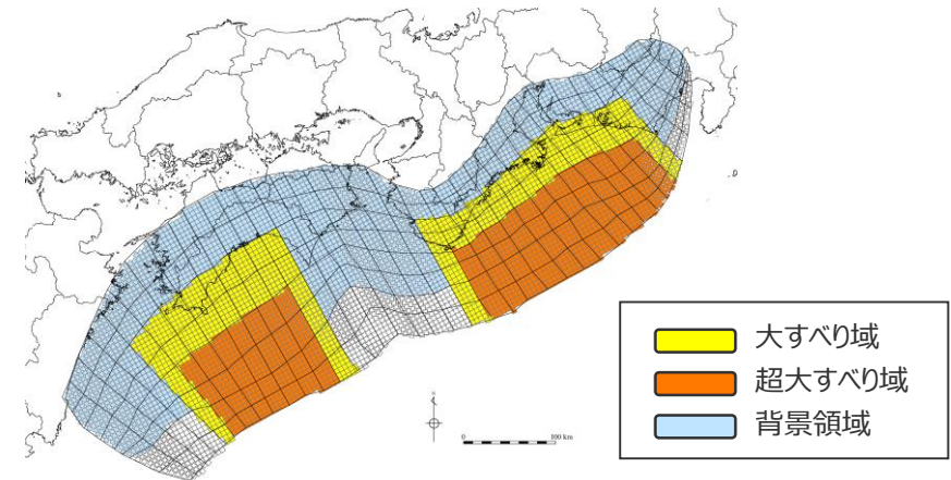
検討波源モデルC (土木学会(2016)手法モデル) の大すべり域の位置を西へ40kmとしたケース
