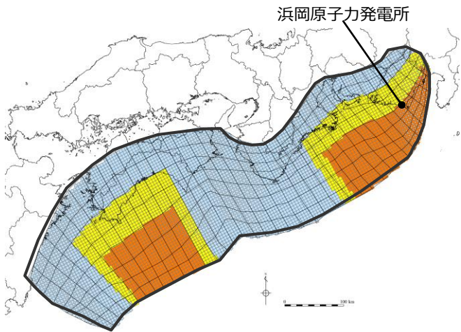
検討波源モデル① (日本海溝の津波評価手法モデル① (広域モデル)) の大すべり域の位置を東へ50kmとしたケース
