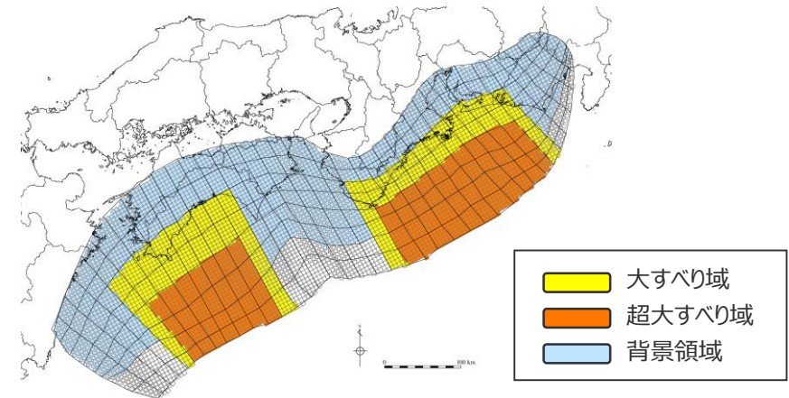
検討波源モデルC (土木学会(2016)手法モデル) の大すべり域の位置を西へ60kmとしたケース
