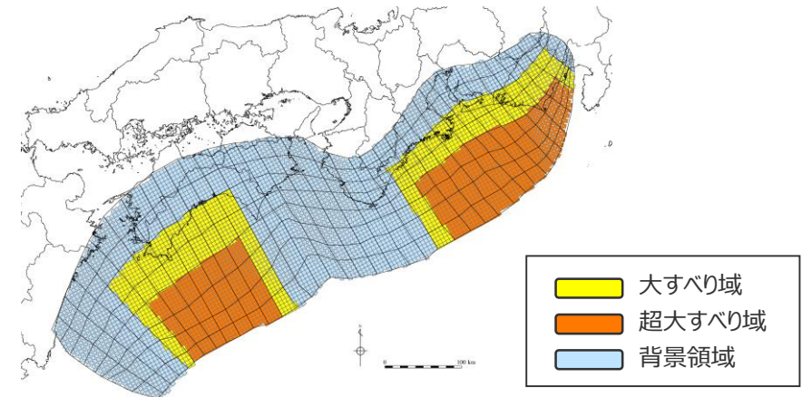
検討波源モデル① (日本海溝の津波評価手法モデル① (広域モデル) ) の大すべり域の位置を東へ20kmとしたケース
