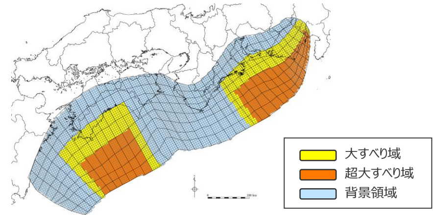
検討波源モデル① (日本海溝の津波評価手法モデル① (広域モデル) ) の大すべり域の位置を東へ50kmとしたケース
