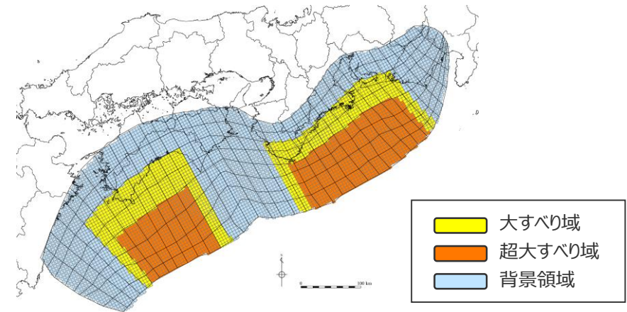
検討波源モデル① (日本海溝の津波評価手法モデル① (広域モデル) ) の大すべり域の位置を西へ70kmとしたケース
