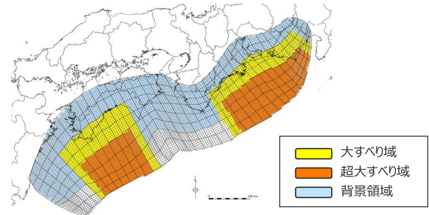
検討波源モデルC (土木学会(2016)手法モデル) の大すべり域の位置を東へ10kmとしたケース
