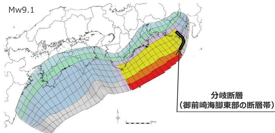
検討波源モデルB-2 (プレート境界面浅部・御前崎海脚東部の断層帯) の大すべり域の位置を西へ30kmとしたケース
