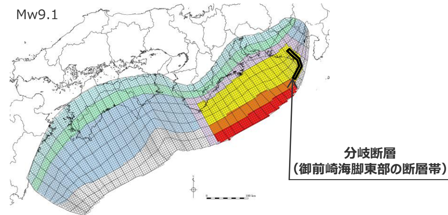
検討波源モデルB-2 (プレート境界面浅部・御前崎海脚東部の断層帯) の大すべり域の位置を西へ20kmとしたケース
