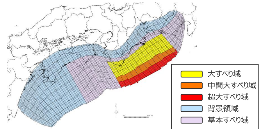
検討波源モデル③ (日本海溝の津波評価手法モデル③ (狭域モデル)) の大すべり域の位置を西へ80kmとしたケース
