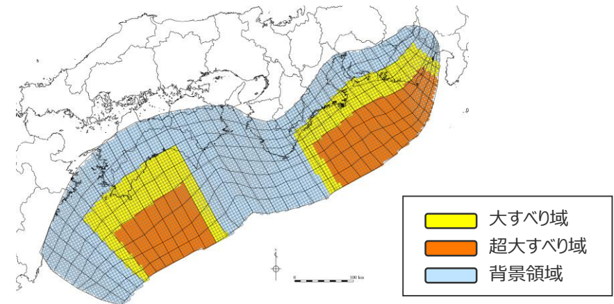
検討波源モデル① (日本海溝の津波評価手法モデル① (広域モデル) ) の大すべり域の位置を東へ10kmとしたケース
