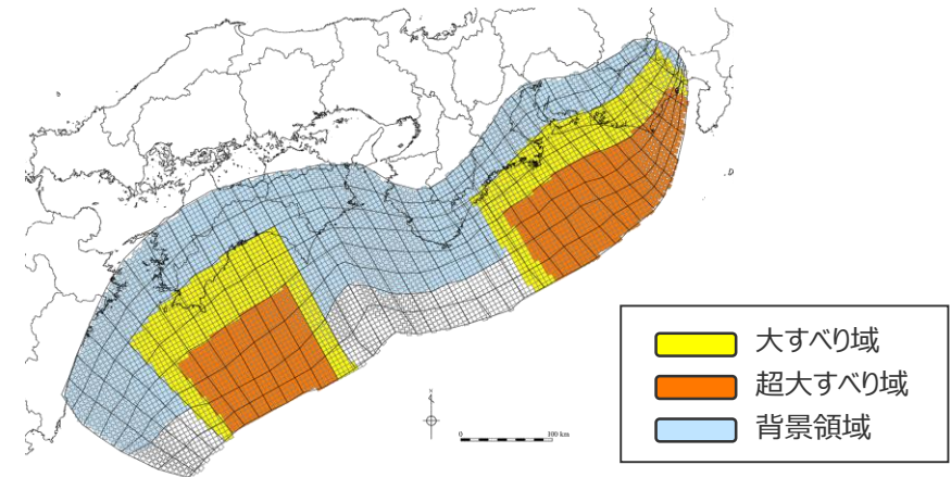
検討波源モデルC (土木学会(2016)手法モデル) の大すべり域の位置を東へ30kmとしたケース
