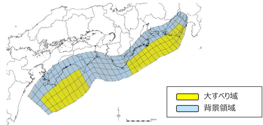
南海トラフ広域の痕跡再現モデル （応力降下量：1.7MPa）
