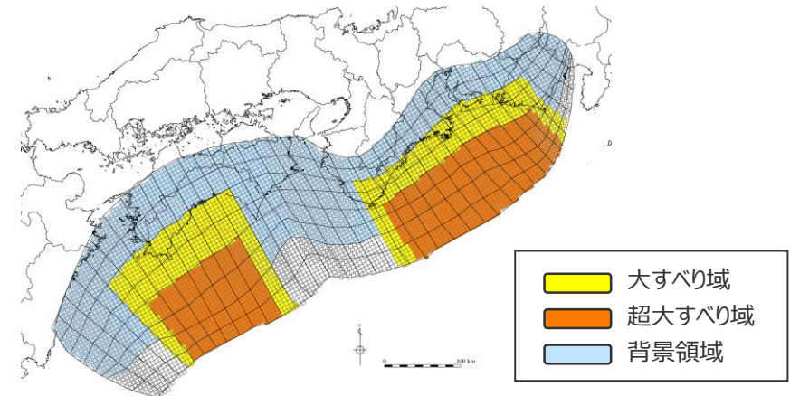
検討波源モデルC (土木学会(2016)手法モデル) の大すべり域の位置を西へ30kmとしたケース
