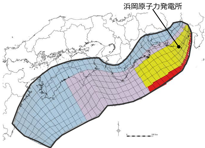
検討波源モデル② (日本海溝の津波評価手法モデル②（狭域モデル） の大すべり域の位置を東へ40kmとしたケース
