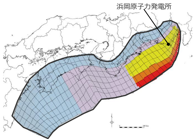
検討波源モデル③ (日本海溝の津波評価手法モデル③(狭域モデル)) の大すべり域の位置を東へ30kmとしたケース
