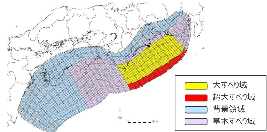
検討波源モデル② (日本海溝の津波評価手法モデル② (狭域モデル)) の大すべり域の位置を西へ60kmとしたケース
