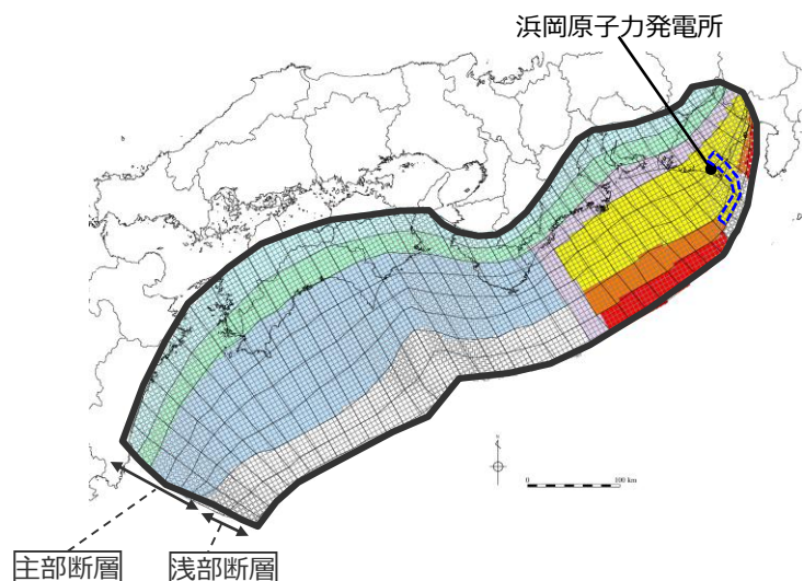
検討波源モデルB-2 (プレート境界面浅部・御前崎海脚東部の断層帯) の大すべり域の位置を東へ40kmとしたケース
