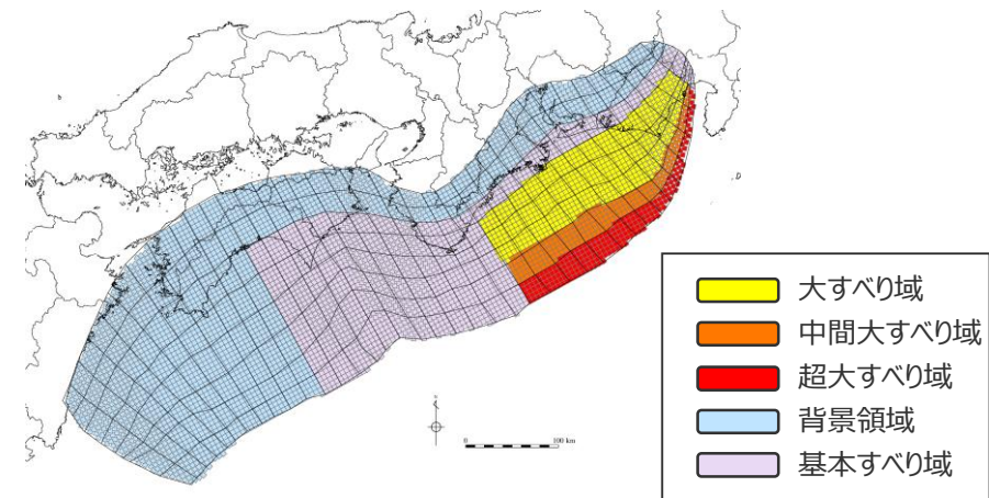
検討波源モデル③ (日本海溝の津波評価手法モデル③ (狭域モデル)) の大すべり域の位置を東へ20kmとしたケース
