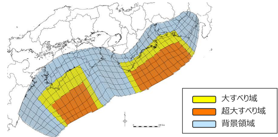
検討波源モデル① (日本海溝の津波評価手法モデル① (広域モデル) ) の大すべり域の位置を西へ60kmとしたケース
