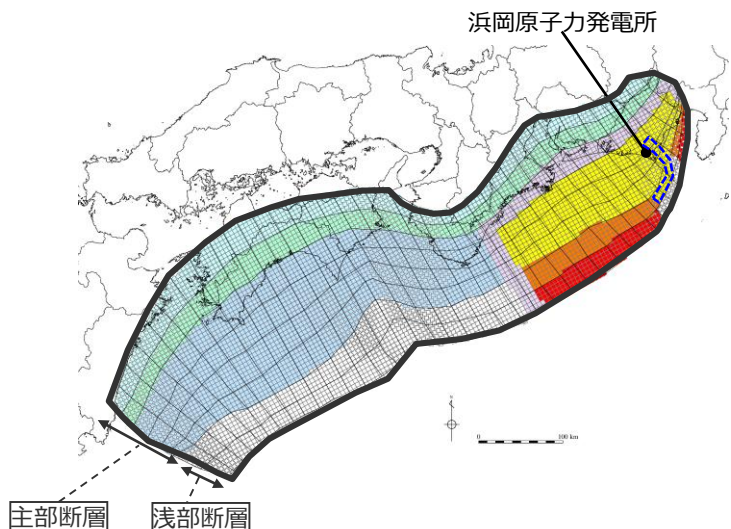
検討波源モデルB-2 (プレート境界面浅部・御前崎海脚東部の断層帯) の大すべり域の位置を東へ30kmとしたケース
