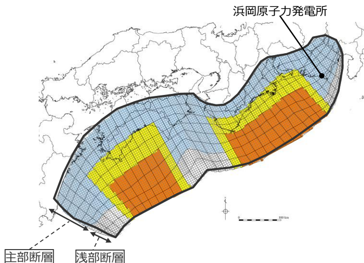
検討波源モデルC (土木学会(2016)手法モデル) の大すべり域の位置を西へ80kmとしたケース
