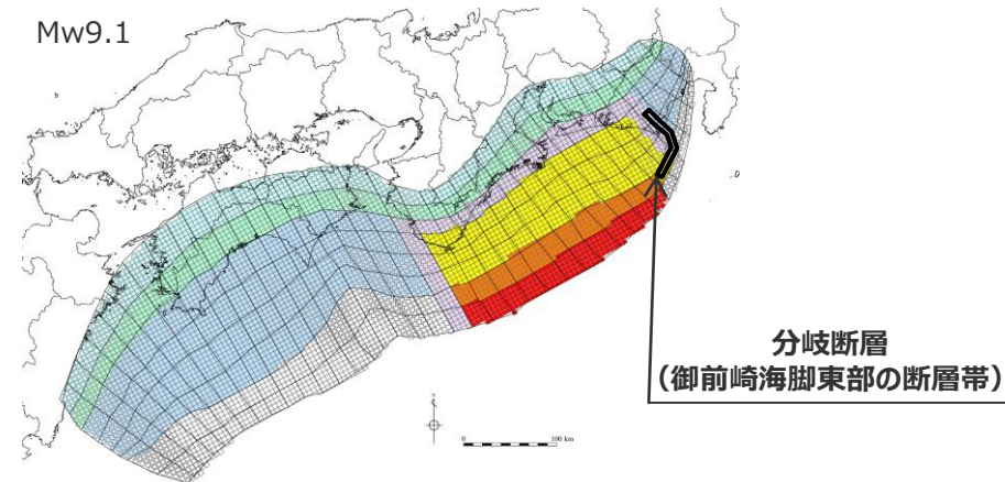
検討波源モデルB-2 (プレート境界面浅部・御前崎海脚東部の断層帯) の大すべり域の位置を西へ50kmとしたケース
