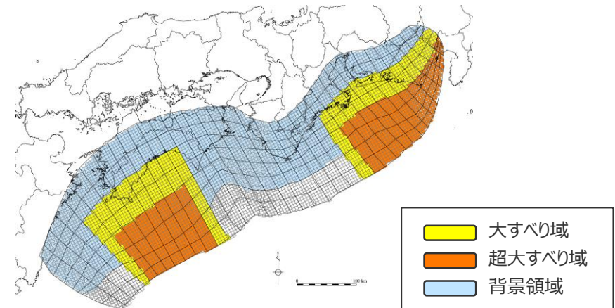
検討波源モデルC (土木学会(2016)手法モデル) の大すべり域の位置を東へ60kmとしたケース
