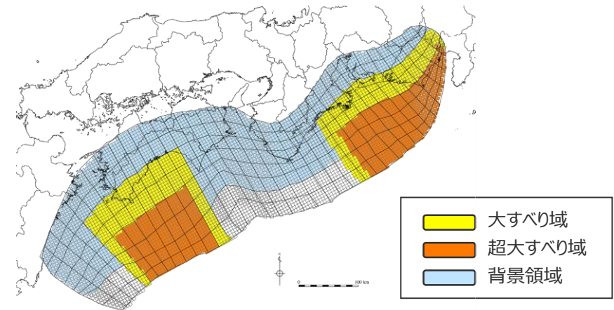
検討波源モデルC (土木学会(2016)手法モデル) の大すべり域の位置を東へ50kmとしたケース
