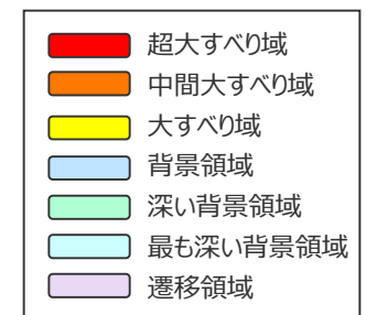
検討波源モデルB-2 (プレート境界面浅部・御前崎海脚東部の断層帯) の大すべり域の位置を西へ20kmとしたケース
