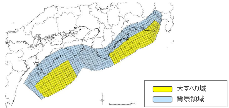
南海トラフ広域の痕跡再現モデル （応力降下量：1.6MPa）
