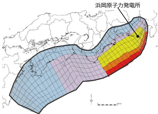
検討波源モデル③ (日本海溝の津波評価手法モデル③（狭域モデル）) の大すべり域の位置を基準位置としたケース
