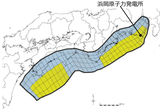
南海トラフ広域の痕跡再現モデル （応力降下量：1.7MPa）
