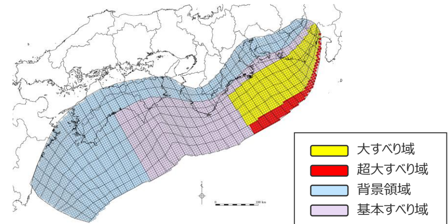
検討波源モデル② (日本海溝の津波評価手法モデル② (狭域モデル)) の大すべり域の位置を東へ40kmとしたケース
