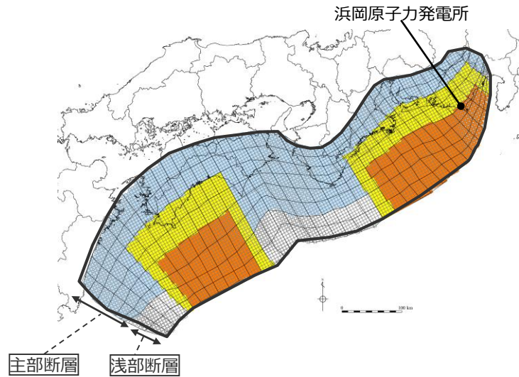
検討波源モデルC (土木学会(2016)手法モデル) の大すべり域の位置を東へ20kmとしたケース
