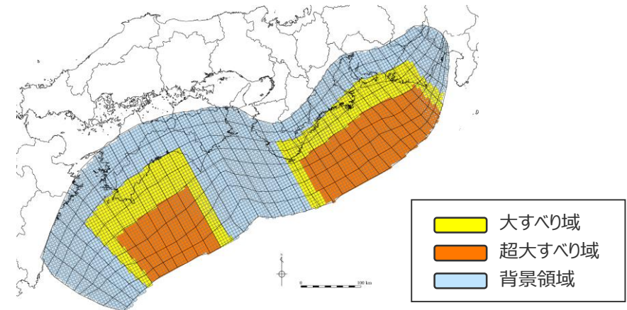
検討波源モデル① (日本海溝の津波評価手法モデル① (広域モデル) ) の大すべり域の位置を西へ30kmとしたケース
