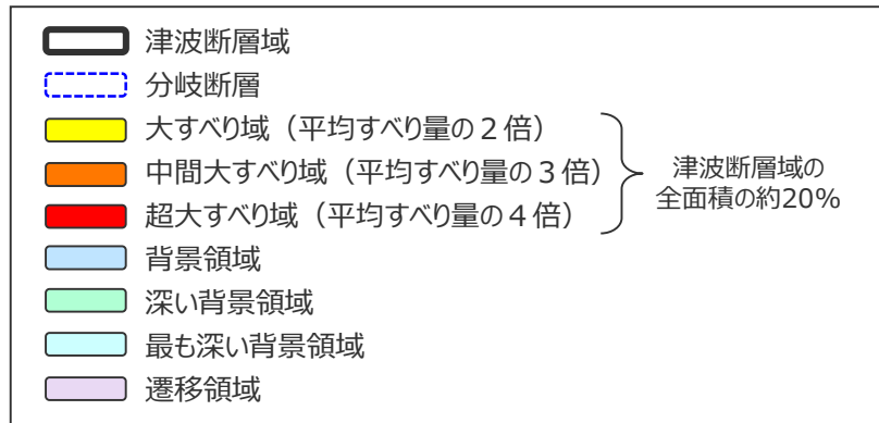
検討波源モデルB-2 (プレート境界面浅部・御前崎海脚東部の断層帯) の大すべり域の位置を西へ30kmとしたケースの小断層のすべり量分布 (m)
