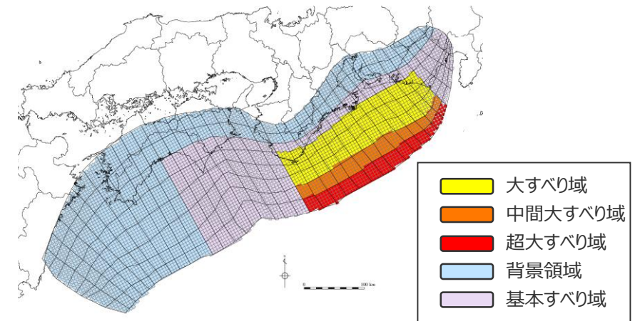
検討波源モデル③ (日本海溝の津波評価手法モデル③ (狭域モデル)) の大すべり域の位置を西へ40kmとしたケース
