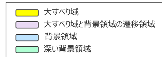
プレートの沈み込み速度を考慮したモデル （応力降下量：1.7MPa）
