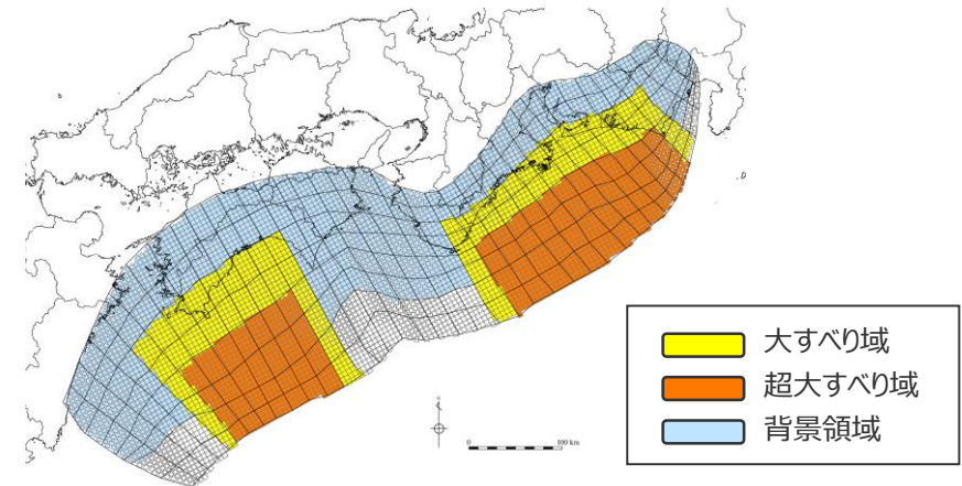
検討波源モデルC (土木学会(2016)手法モデル) の大すべり域の位置を西へ20kmとしたケース
