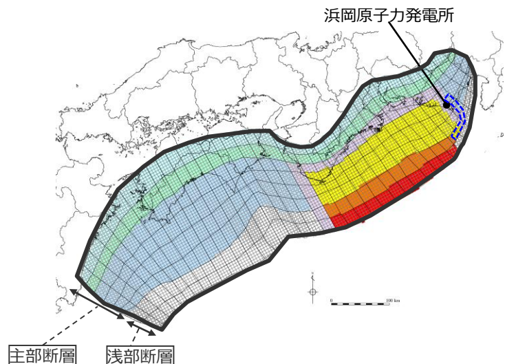
検討波源モデルB-2 (プレート境界面浅部・御前崎海脚東部の断層帯) の大すべり域の位置を西へ50kmとしたケース
