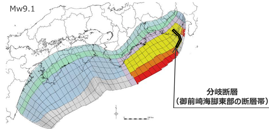
検討波源モデルB-2 (プレート境界面浅部・御前崎海脚東部の断層帯) の大すべり域の位置を基準位置としたケース
