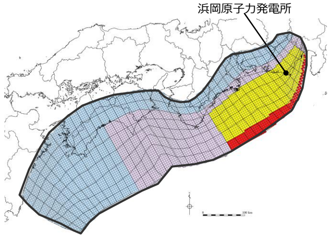
検討波源モデル② (日本海溝の津波評価手法モデル②（狭域モデル） の大すべり域の位置を東へ20kmとしたケース
