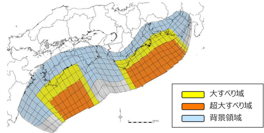
検討波源モデルC (土木学会(2016)手法モデル) の大すべり域の位置を西へ50kmとしたケース
