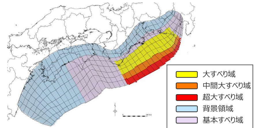
検討波源モデル③ (日本海溝の津波評価手法モデル③ (狭域モデル))
