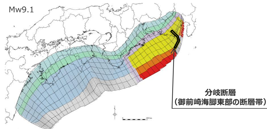
検討波源モデルB-2 (プレート境界面浅部・御前崎海脚東部の断層帯) の大すべり域の位置を東へ30kmとしたケース
