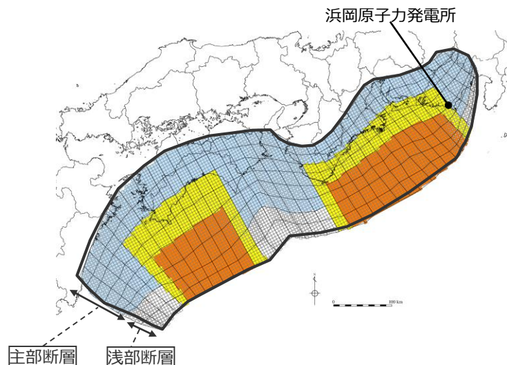
検討波源モデルC (土木学会(2016)手法モデル) の大すべり域の位置を西へ40kmとしたケース
