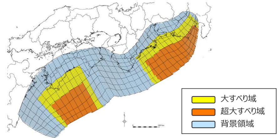
検討波源モデル① (日本海溝の津波評価手法モデル① (広域モデル) ) の大すべり域の位置を東へ30kmとしたケース
