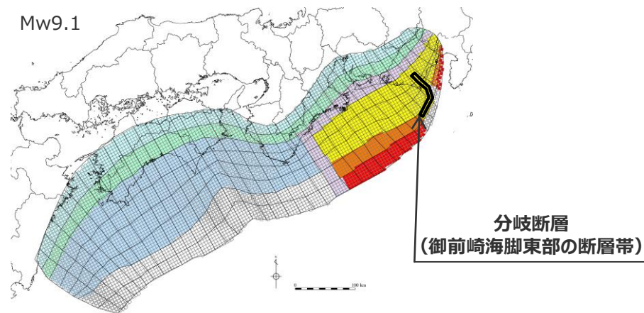
検討波源モデルB-2 (プレート境界面浅部・御前崎海脚東部の断層帯) の大すべり域の位置を東へ40kmとしたケース
