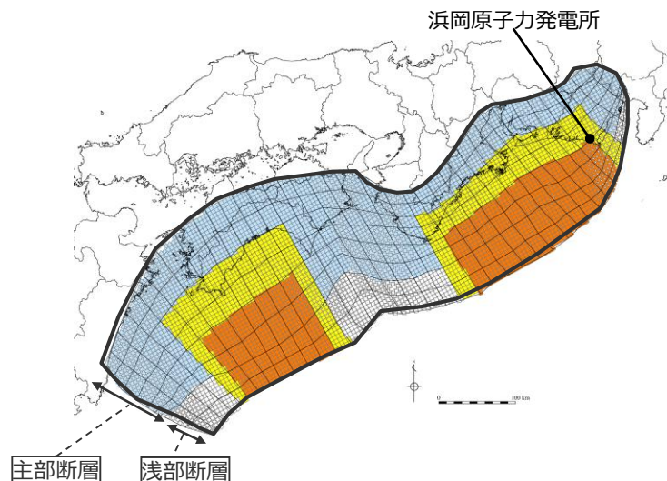
検討波源モデルC (土木学会(2016)手法モデル) の大すべり域の位置を西へ20kmとしたケース
