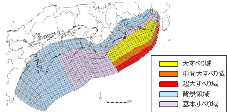
検討波源モデル③ (日本海溝の津波評価手法モデル③ (狭域モデル)) の大すべり域の位置を基準位置としたケース
