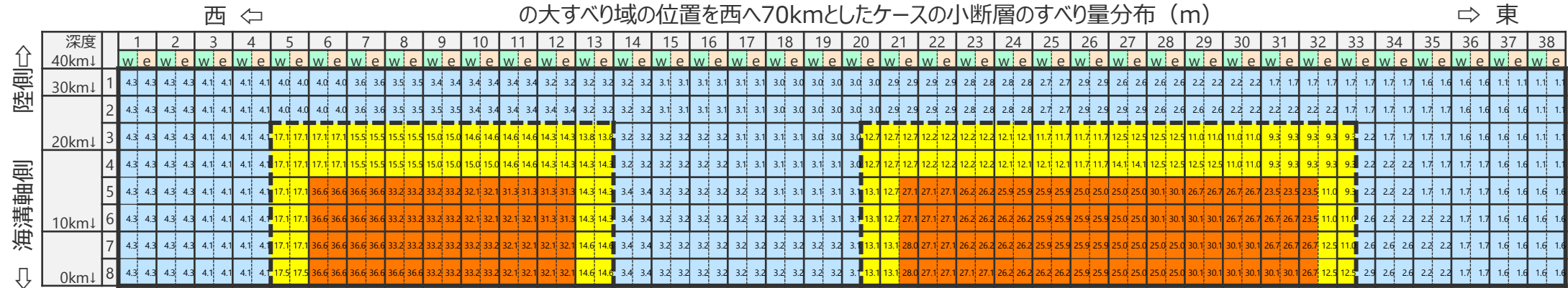
検討波源モデル① (日本海溝の津波評価手法モデル① (広域モデル)) の大すべり域の位置を西へ70kmとしたケース
