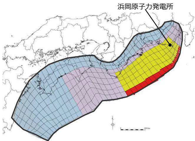
検討波源モデル② (日本海溝の津波評価手法モデル②（狭域モデル）) の大すべり域の位置を西へ20kmとしたケース
