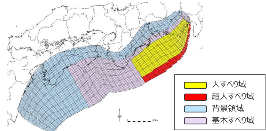
検討波源モデル② (日本海溝の津波評価手法モデル② (狭域モデル)) の大すべり域の位置を東へ20kmとしたケース
