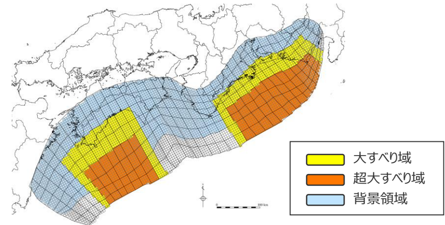
検討波源モデルC (土木学会(2016)手法モデル) の大すべり域の位置を基準位置としたケース
