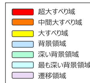
検討波源モデルB-2 (プレート境界面浅部・御前崎海脚東部の断層帯) の大すべり域の位置を東へ40kmとしたケース
