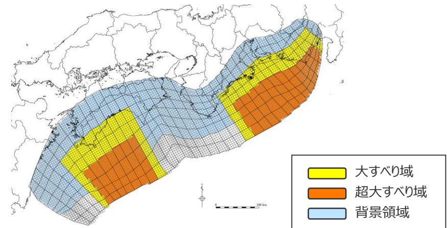
検討波源モデルC (土木学会(2016)手法モデル) の大すべり域の位置を東へ20kmとしたケース
