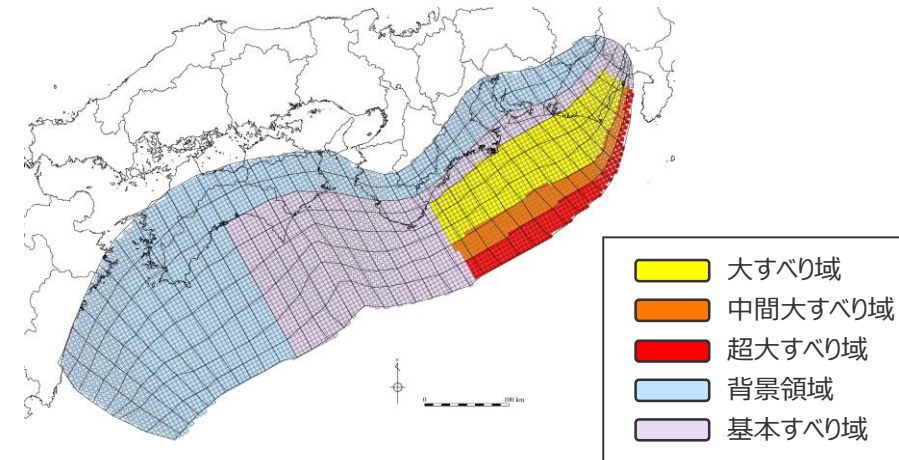
検討波源モデル③ (日本海溝の津波評価手法モデル③ (狭域モデル)) の大すべり域の位置を東へ10kmとしたケース
