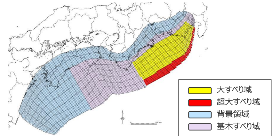
検討波源モデル② (日本海溝の津波評価手法モデル② (狭域モデル)) の大すべり域の位置を東へ10kmとしたケース
