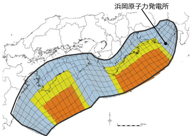
検討波源モデル① (日本海溝の津波評価手法モデル①（広域モデル）) の大すべり域の位置を西へ60kmとしたケース
