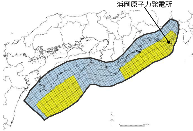
南海トラフ広域の痕跡再現モデル （応力降下量：1.6MPa）
