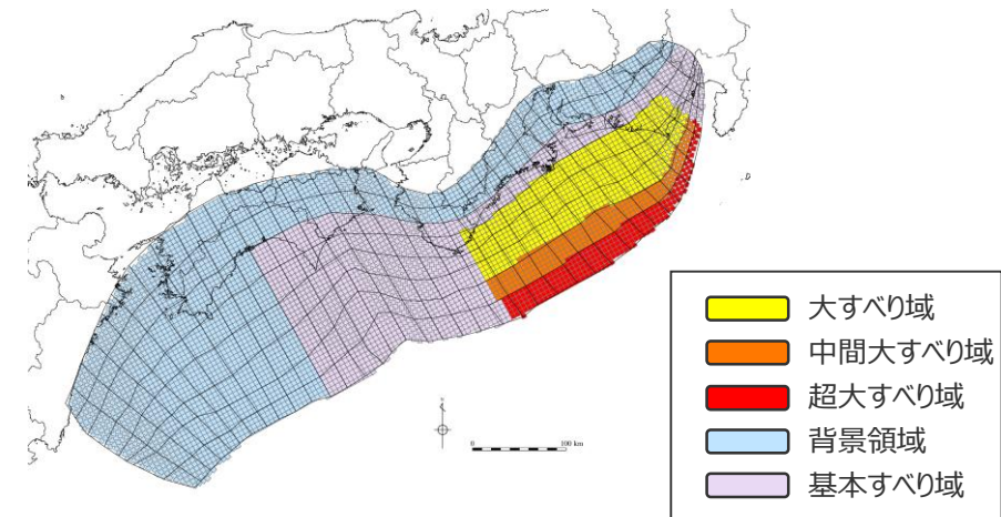
検討波源モデル③ (日本海溝の津波評価手法モデル③ (狭域モデル)) の大すべり域の位置を西へ10kmとしたケース
