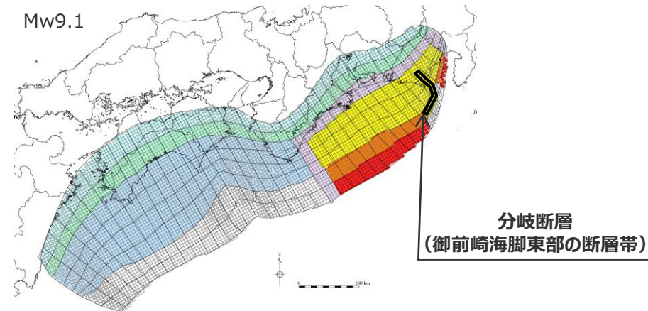
検討波源モデルB-2 (プレート境界面浅部・御前崎海脚東部の断層帯) の大すべり域の位置を東へ20kmとしたケース
