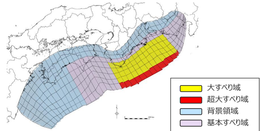
検討波源モデル② (日本海溝の津波評価手法モデル② (狭域モデル)) の大すべり域の位置を西へ80kmとしたケース
