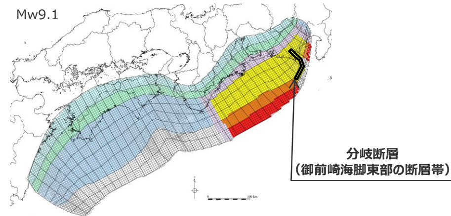
検討波源モデルB-2 (プレート境界面浅部・御前崎海脚東部の断層帯) の大すべり域の位置を東へ10kmとしたケース
