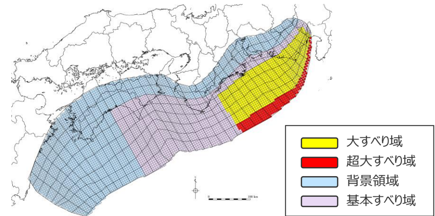
検討波源モデル② (日本海溝の津波評価手法モデル② (狭域モデル)) の大すべり域の位置を東へ30kmとしたケース
