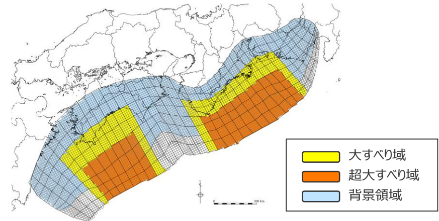
検討波源モデルC (土木学会(2016)手法モデル) の大すべり域の位置を西へ80kmとしたケース
