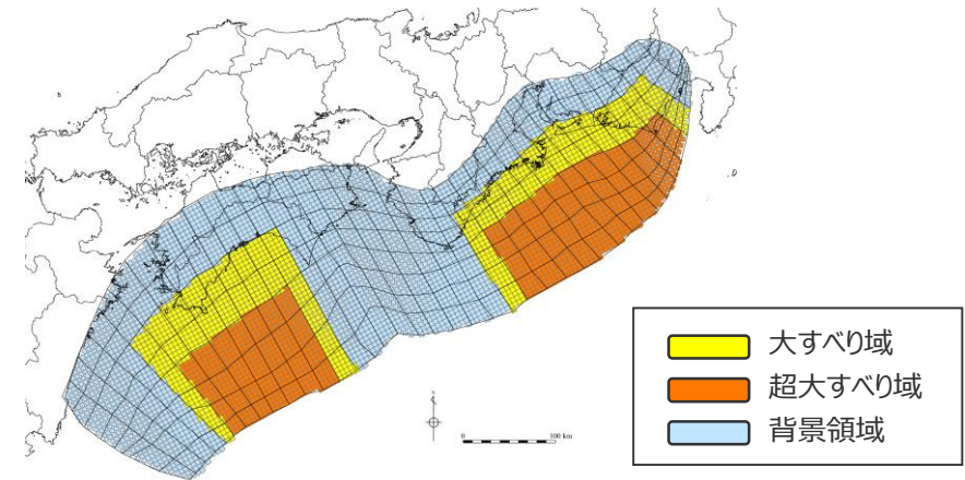
検討波源モデル① (日本海溝の津波評価手法モデル① (広域モデル) ) の大すべり域の位置を基準位置としたケース
