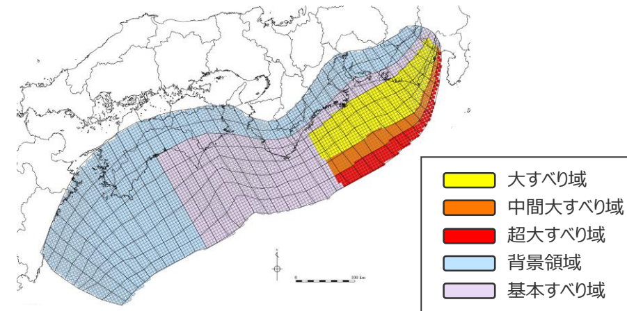
検討波源モデル③ (日本海溝の津波評価手法モデル③ (狭域モデル)) の大すべり域の位置を東へ30kmとしたケース
