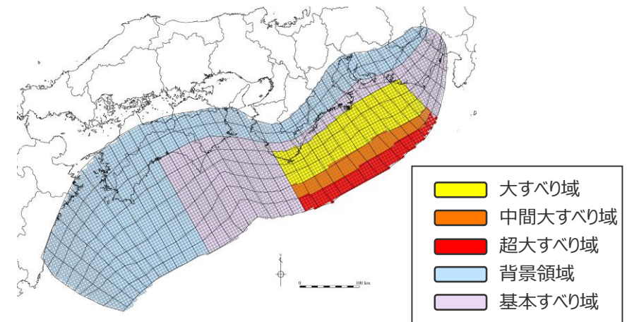
検討波源モデル③ (日本海溝の津波評価手法モデル③ (狭域モデル)) の大すべり域の位置を西へ60kmとしたケース
