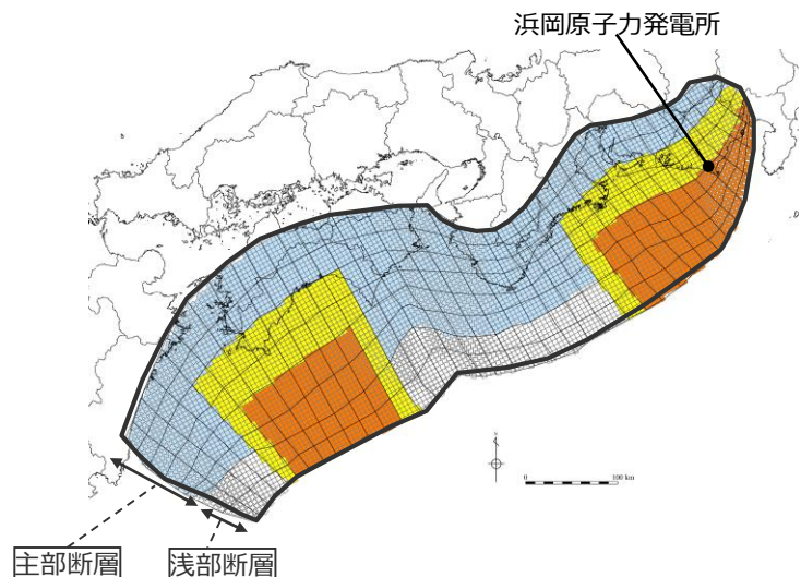
検討波源モデルC (土木学会(2016)手法モデル) の大すべり域の位置を東へ60kmとしたケース
