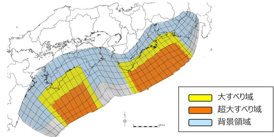
検討波源モデルC (土木学会(2016)手法モデル) の大すべり域の位置を西へ70kmとしたケース
