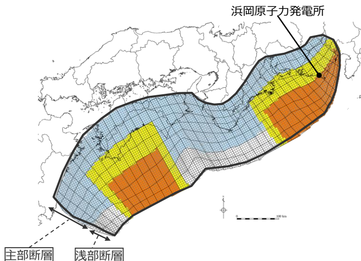
検討波源モデルC (土木学会(2016)手法モデル) の大すべり域の位置を東へ50kmとしたケース
