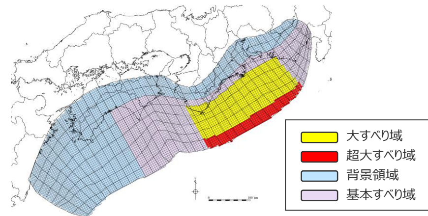
検討波源モデル② (日本海溝の津波評価手法モデル② (狭域モデル)) の大すべり域の位置を西へ70kmとしたケース
