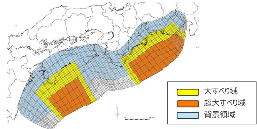
検討波源モデルC (土木学会(2016)手法モデル) の大すべり域の位置を西へ10kmとしたケース
