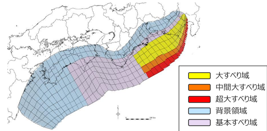
検討波源モデル③ (日本海溝の津波評価手法モデル③ (狭域モデル)) の大すべり域の位置を東へ40kmとしたケース
