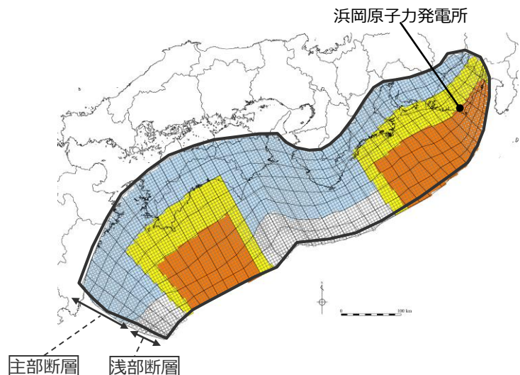
検討波源モデルC (土木学会(2016)手法モデル) の大すべり域の位置を東へ40kmとしたケース
