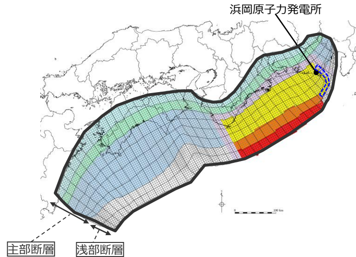
検討波源モデルB-2 (プレート境界面浅部・御前崎海脚東部の断層帯) の大すべり域の位置を西へ30kmとしたケース
