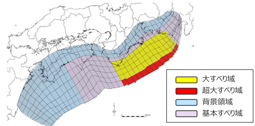
検討波源モデル② (日本海溝の津波評価手法モデル② (狭域モデル)) の大すべり域の位置を西へ50kmとしたケース
