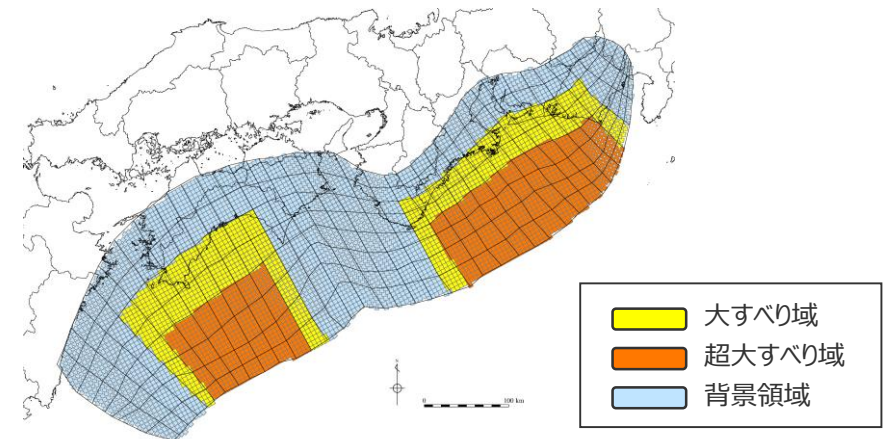
検討波源モデル① (日本海溝の津波評価手法モデル① (広域モデル) ) の大すべり域の位置を西へ20kmとしたケース
