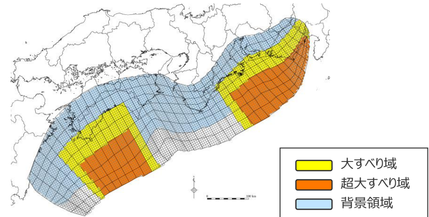
検討波源モデルC (土木学会(2016)手法モデル) の大すべり域の位置を東へ40kmとしたケース
