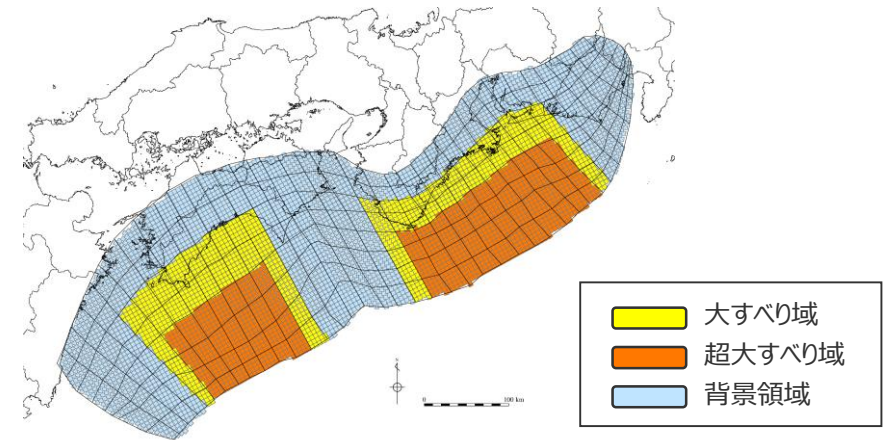
検討波源モデル① (日本海溝の津波評価手法モデル① (広域モデル) ) の大すべり域の位置を西へ80kmとしたケース
