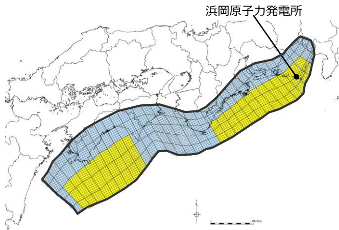
南海トラフ広域の痕跡再現モデル （応力降下量：1.9MPa）
