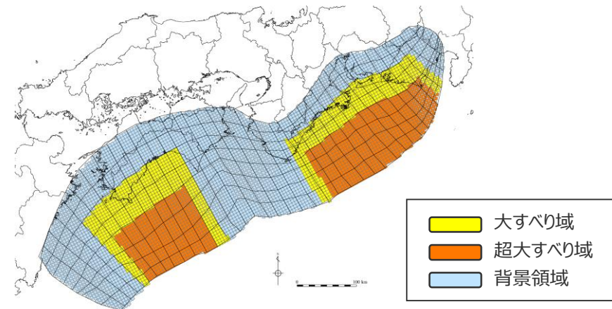
検討波源モデル① (日本海溝の津波評価手法モデル① (広域モデル) ) の大すべり域の位置を西へ10kmとしたケース
