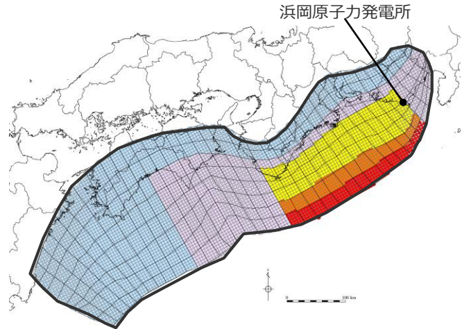
検討波源モデル③ (日本海溝の津波評価手法モデル③(狭域モデル)) の大すべり域の位置を西へ40kmとしたケース
