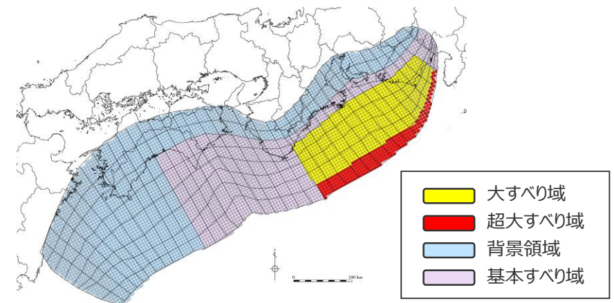
検討波源モデル② (日本海溝の津波評価手法モデル② (狭域モデル)) の大すべり域の位置を基準位置としたケース
