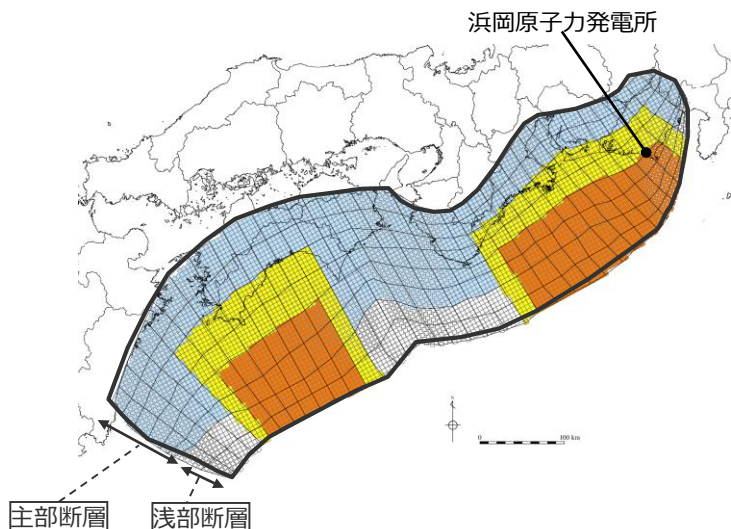
検討波源モデルC (土木学会(2016)手法モデル) の大すべり域の位置を基準位置としたケース
