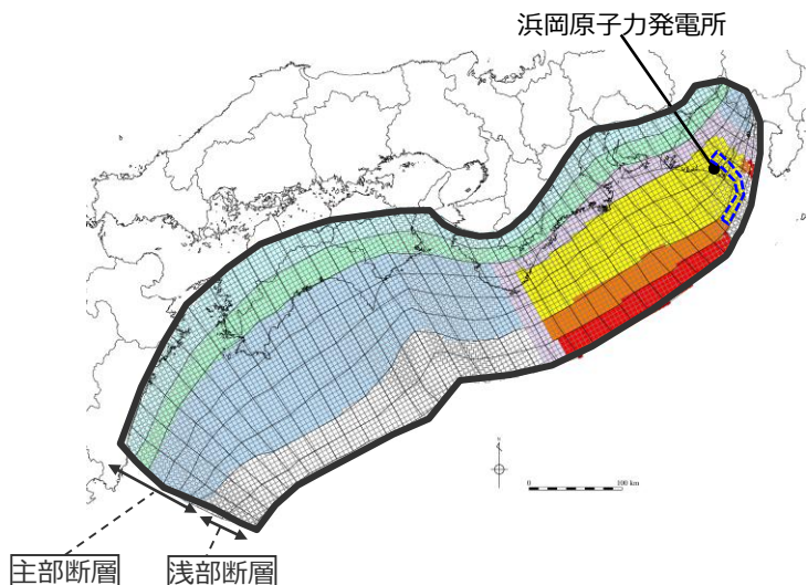
検討波源モデルB-2 (プレート境界面浅部・御前崎海脚東部の断層帯) の大すべり域の位置を西へ10kmとしたケース
