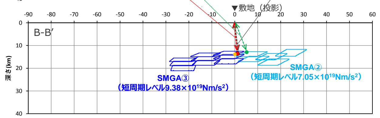
(断面図 (投影))
