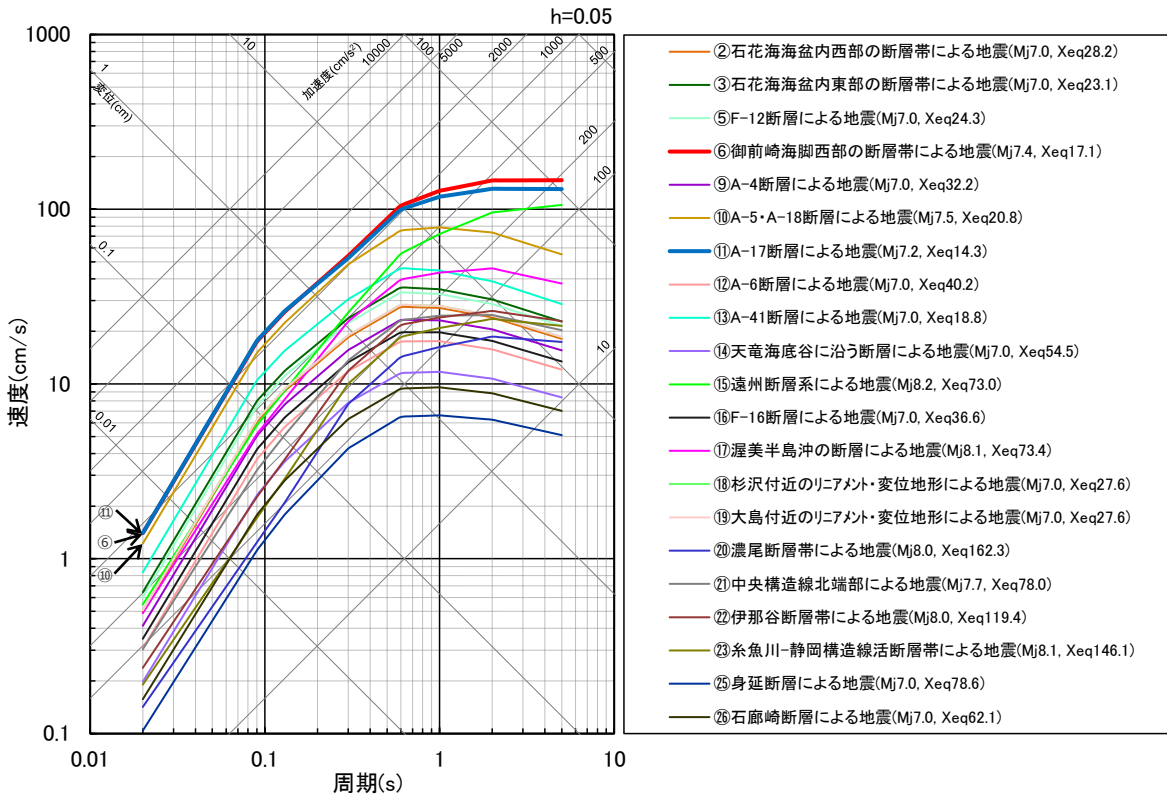
<Noda et al.(2002)による応答スペクトルの比較※1> (内陸地殻内地震の震源として考慮する活断層による地震（一様断層モデル）)
