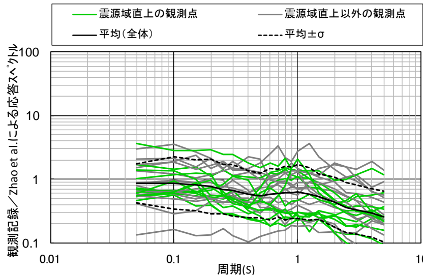
<1985年チリ地震の観測記録と Zhao et al.(2006)による応答スペクトルとの比>
