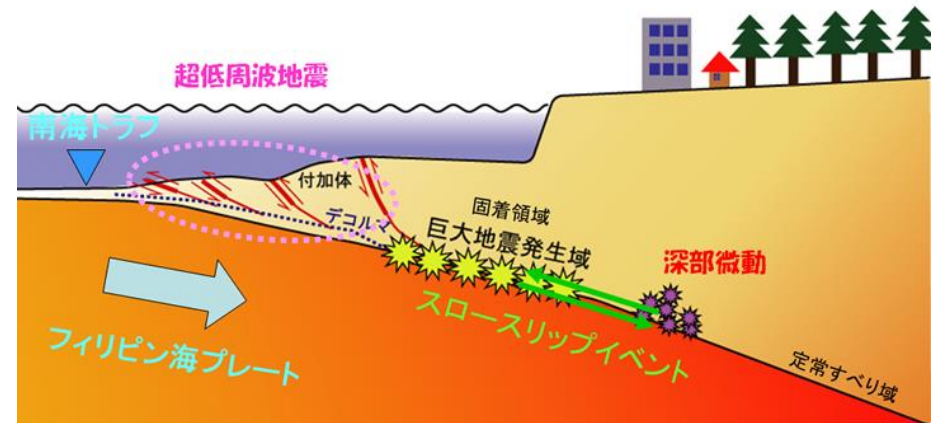
<西南日本におけるプレート沈み込み帯の模式図> (防災科研「2010年12月10日プレス発表」より引用)
