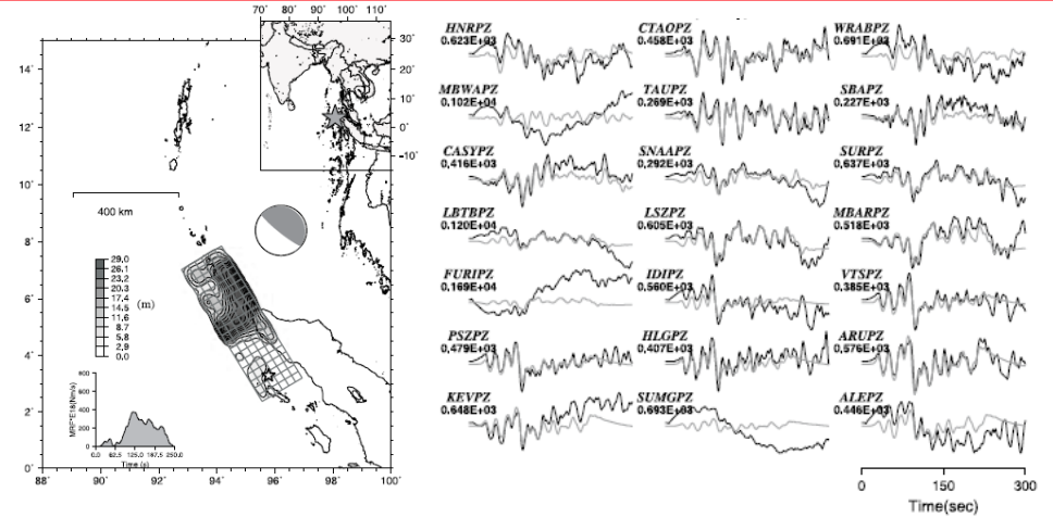
＜震源インバージョン解析による2004年Sumatra地震 (Mw9.1) の最終すべり分布 (左) 及び観測波形と理論波形の比較 (右) の例＞ (八木(2004)による)
