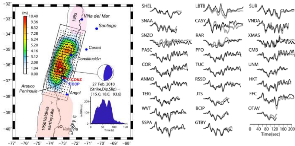
＜震源インバージョン解析による2010年Maule地震 (Mw8.8) の最終すべり分布 (左) 及び観測波形と理論波形の比較 (右) の例＞ (Pulido et al.(2011)による)
