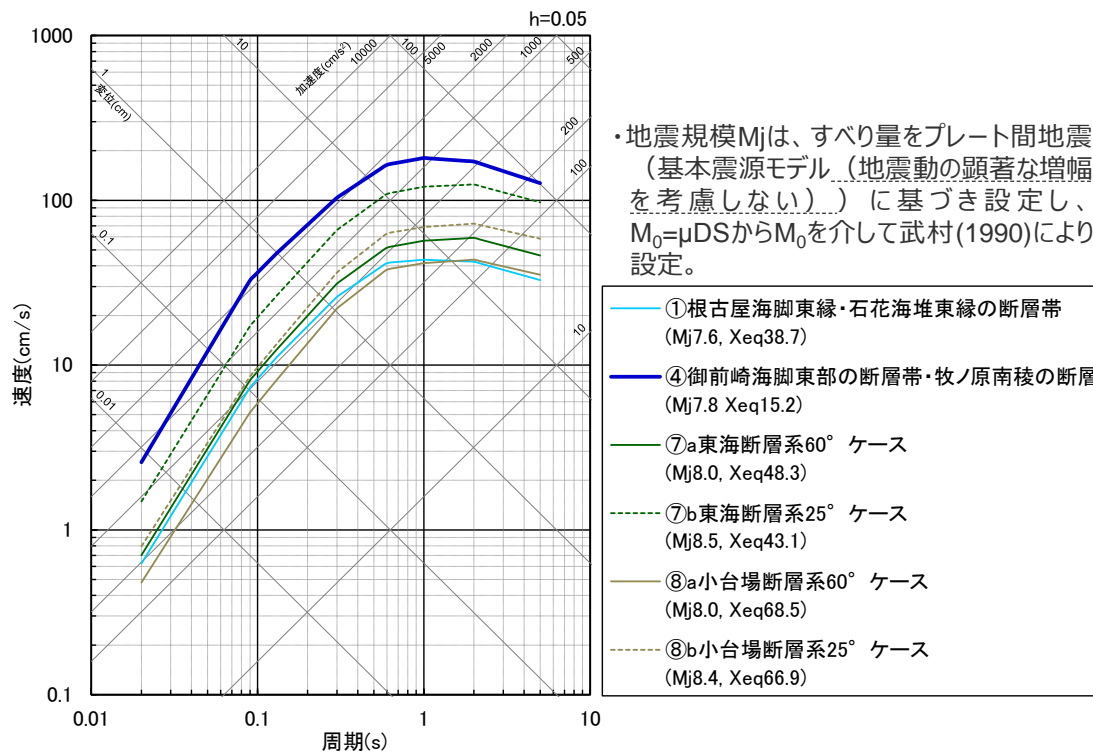
<Noda et al.(2002)による応答スペクトルの比較※1> (プレート間地震に伴う分岐断層)
