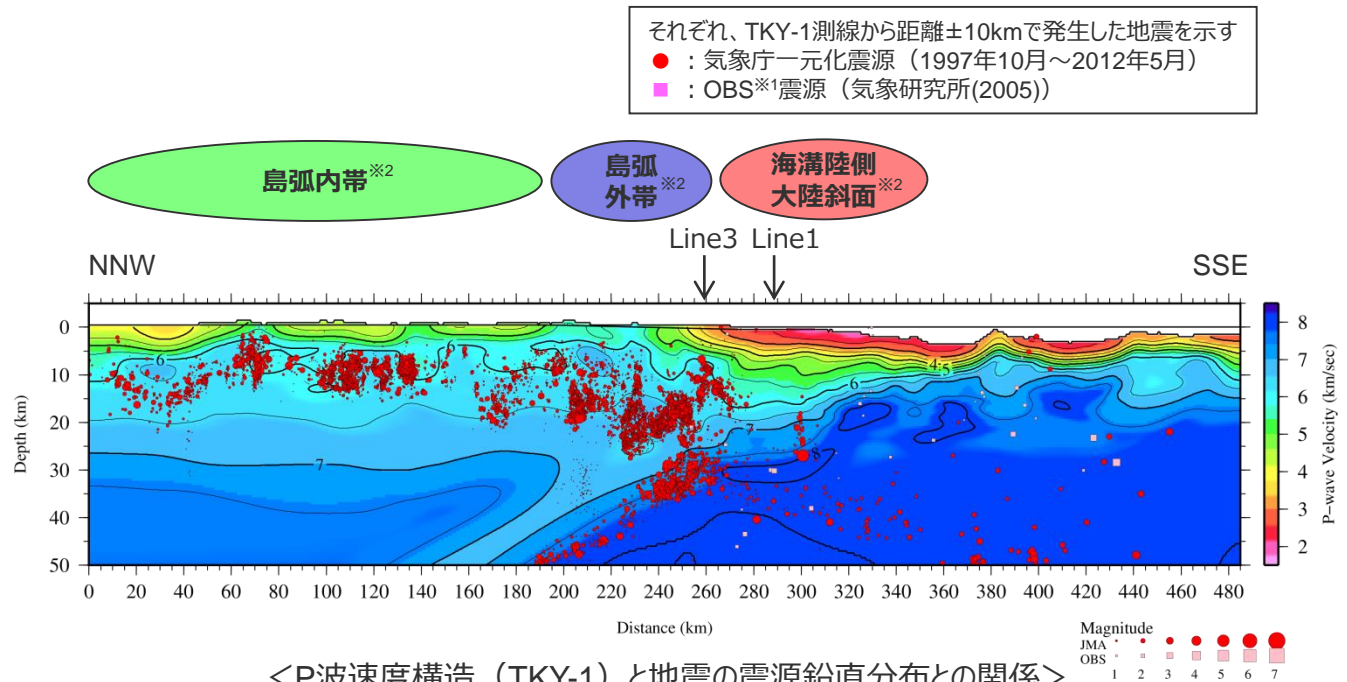
<P波速度構造 (TKY-1) と地震の震源鉛直分布との関係> (Kodaira et al.(2004)に地震地体構造区分・震源鉛直分布を重ね描き)
