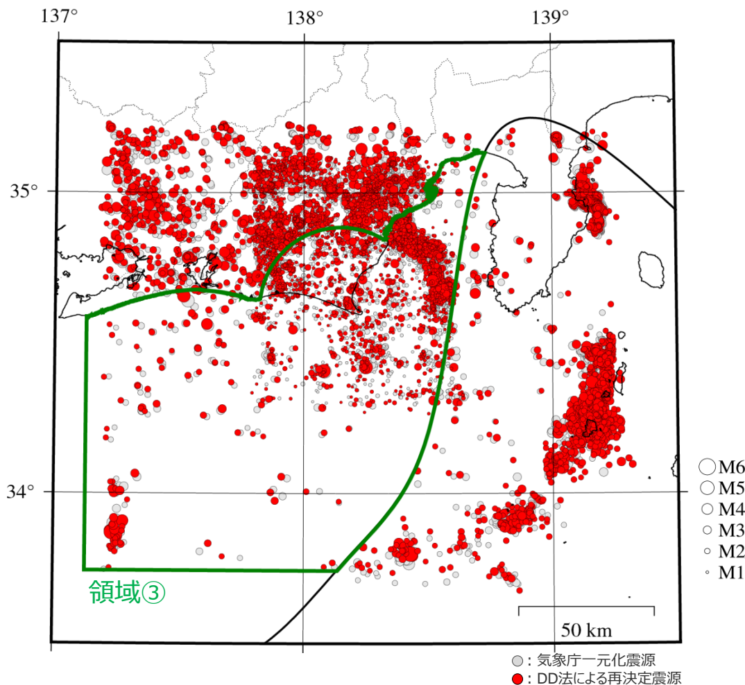
<DD法による再決定震源と気象庁一元化震源の分布> (観測期間1997年10月～2015年12月)
