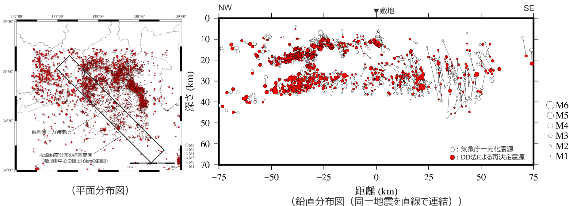
<気象庁一元化震源とDD法による再決定震源の微小地震分布との比較> (観測期間1997年10月～2015年12月)
