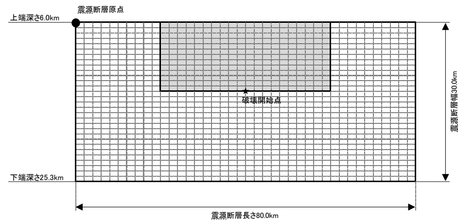
（展開図）
