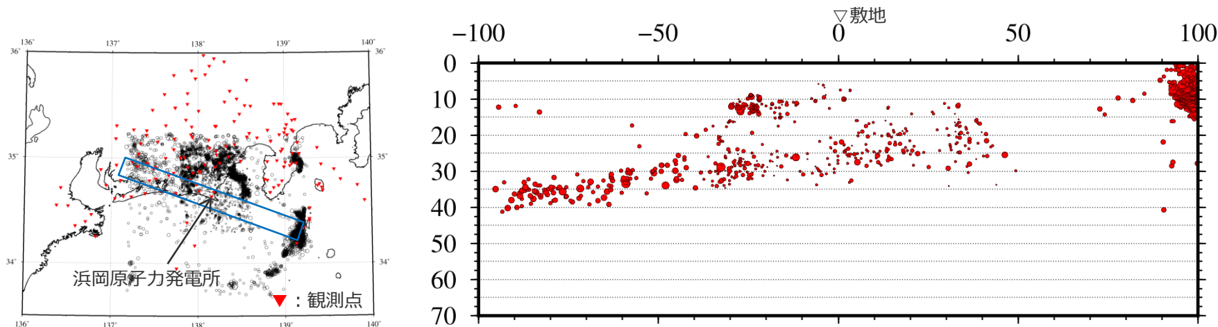
<敷地周辺の震源鉛直分布> (震源再決定)
