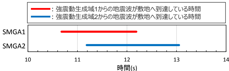
＜各強震動生成域からの地震波の重なり＞
