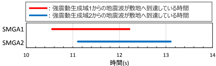
<各強震動生成域からの地震波の重なり>
