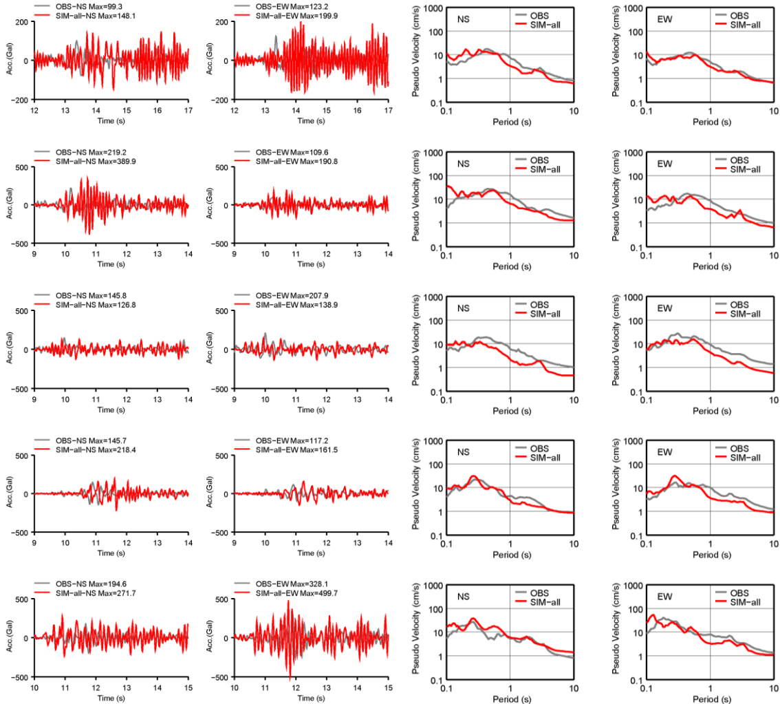
<経験的グリーン関数法によるシミュレーション結果と観測記録との比較（広域②）>
