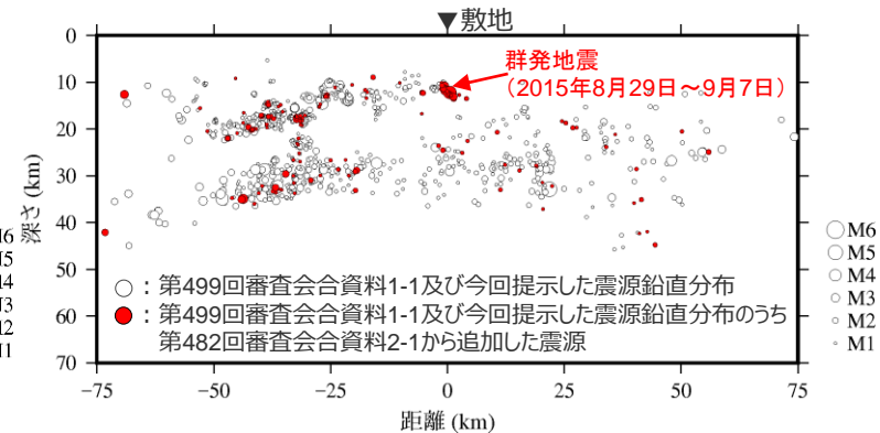
<第499回審査会合資料1-1及び今回提示した震央分布及び震源鉛直分布> データ期間:1997年10月～2015年12月、震源の数:11,629個、走時の数:2,025,903本
