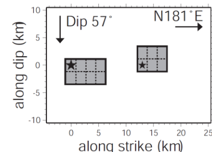
(2001年芸予地震、Asano et al.(2004))
