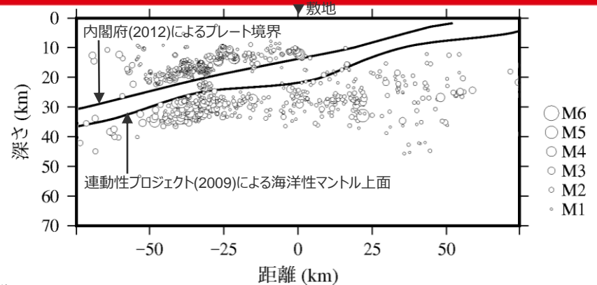
<敷地周辺の震源鉛直分布（観測期間1997年10月～2015年12月）>
