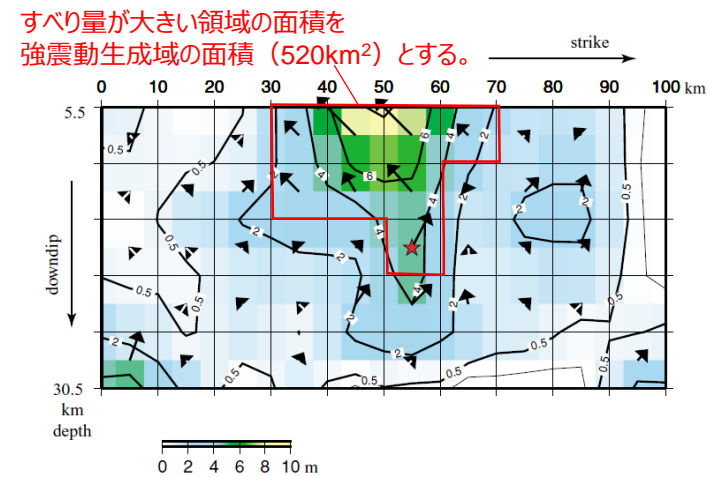
<2004年紀伊半島南東沖の地震の震源インバージョン結果> (Park and Mori(2005)にすべり量大きい領域を加筆)
