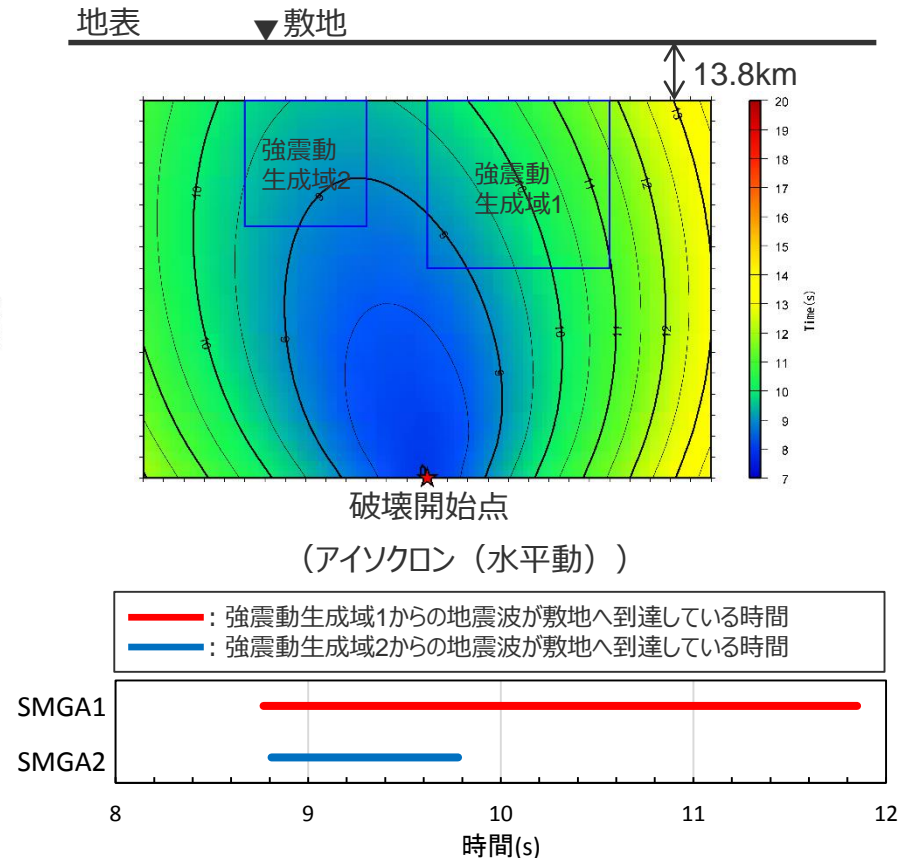
(各強震動生成域からの地震波の重なり) <震源深さの不確かさを考慮した震源モデル (断層位置の不確かさを考慮した震源モデルに基づく) (地震動の顕著な増幅を考慮しない)>
