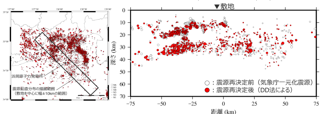
<第499回審査会合資料1-1及び今回提示した震央分布及び震源鉛直分布> データ期間:1997年10月～2015年12月、震源の数:11,629個、走時の数:2,025,903本
