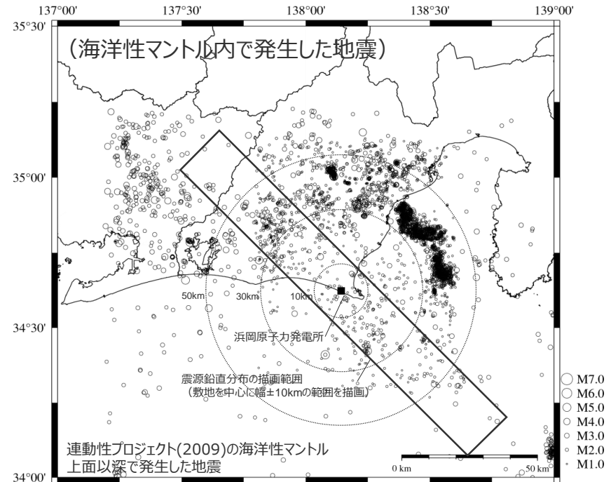
<敷地を中心として広域で発生した地震の震央分布（観測期間1997年10月～2015年12月）>
