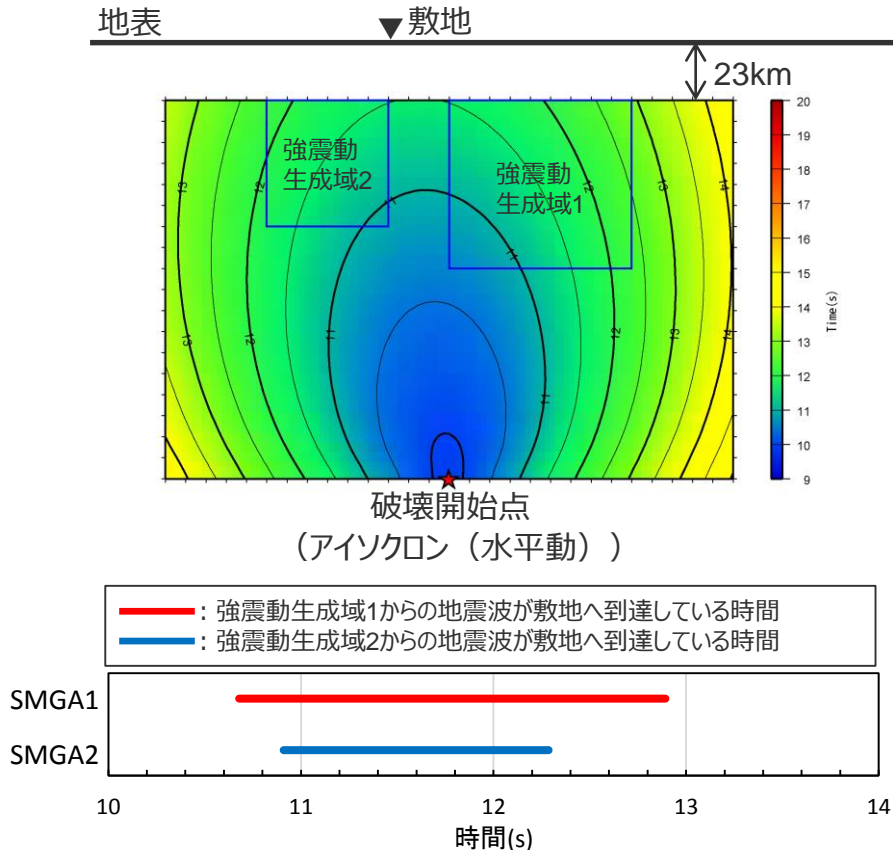
(各強震動生成域からの地震波の重なり) <断層位置の不確かさを考慮した震源モデル (地震動の顕著な増幅を考慮しない)>
