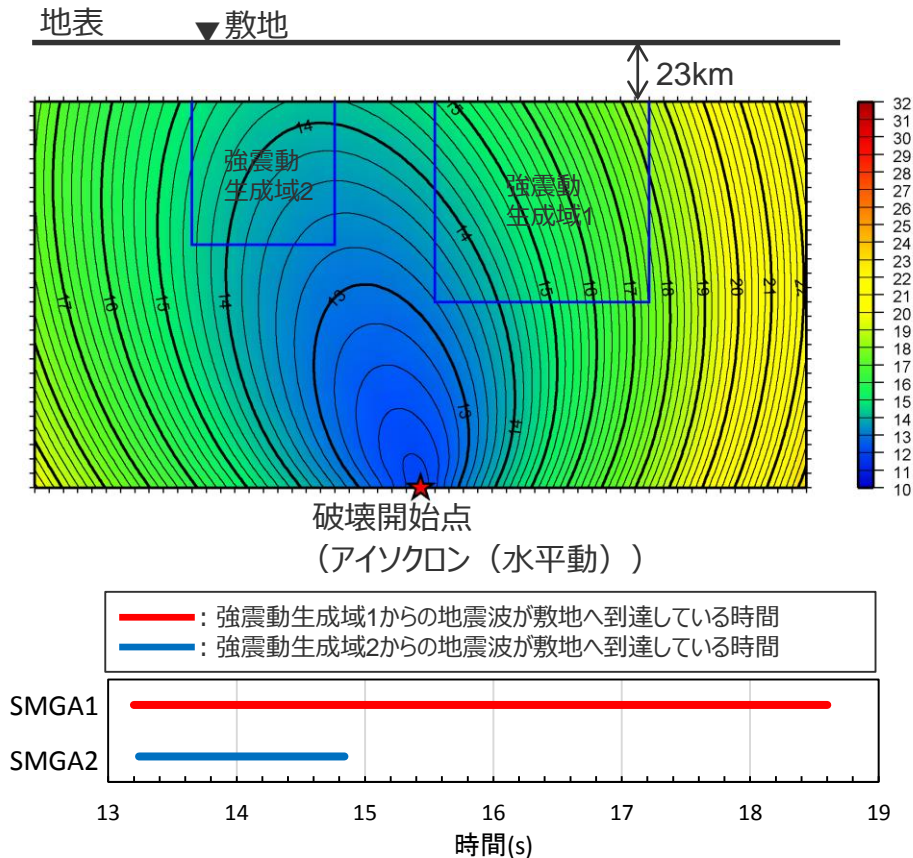
(各強震動生成域からの地震波の重なり) <地震規模の不確かさを考慮した震源モデル (断層位置の不確かさを考慮した震源モデルに基づく) (地震動の顕著な増幅を考慮しない)>
