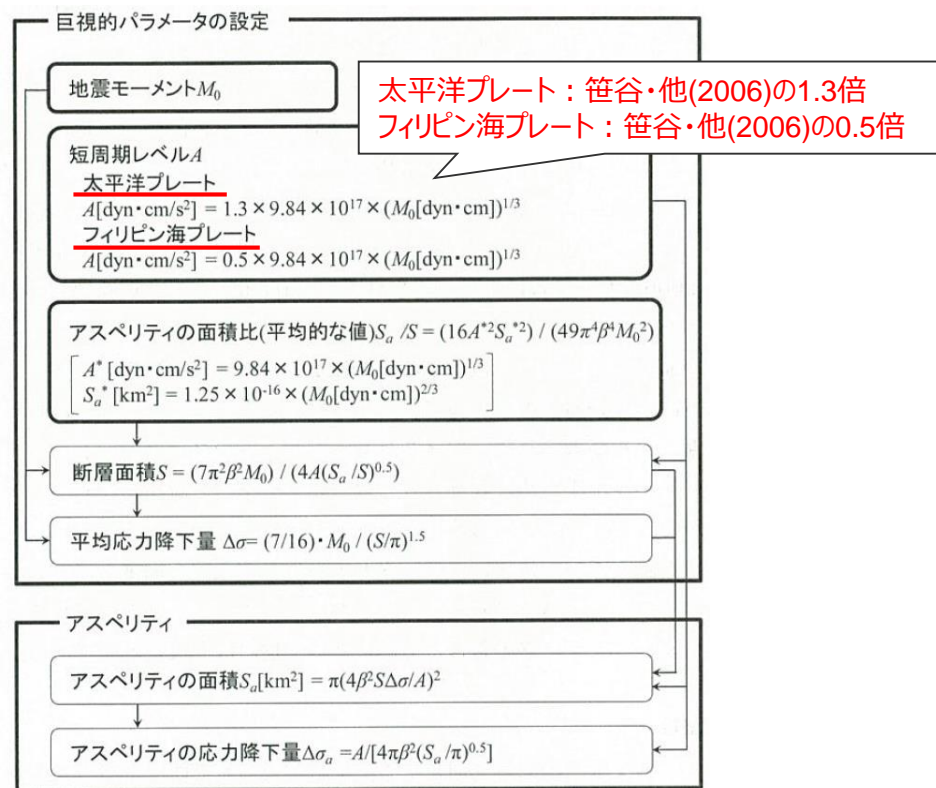
<スラブ内地震の断層パラメータ設定方法> (新井・他(2015)に下線、笹谷・他(2006)との関係を加筆)
