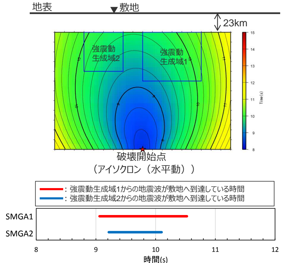
(各強震動生成域からの地震波の重なり) <短周期レベルの不確かさを考慮した震源モデル (断層位置の不確かさを考慮した震源モデルに基づく) (地震動の顕著な増幅を考慮しない)>
