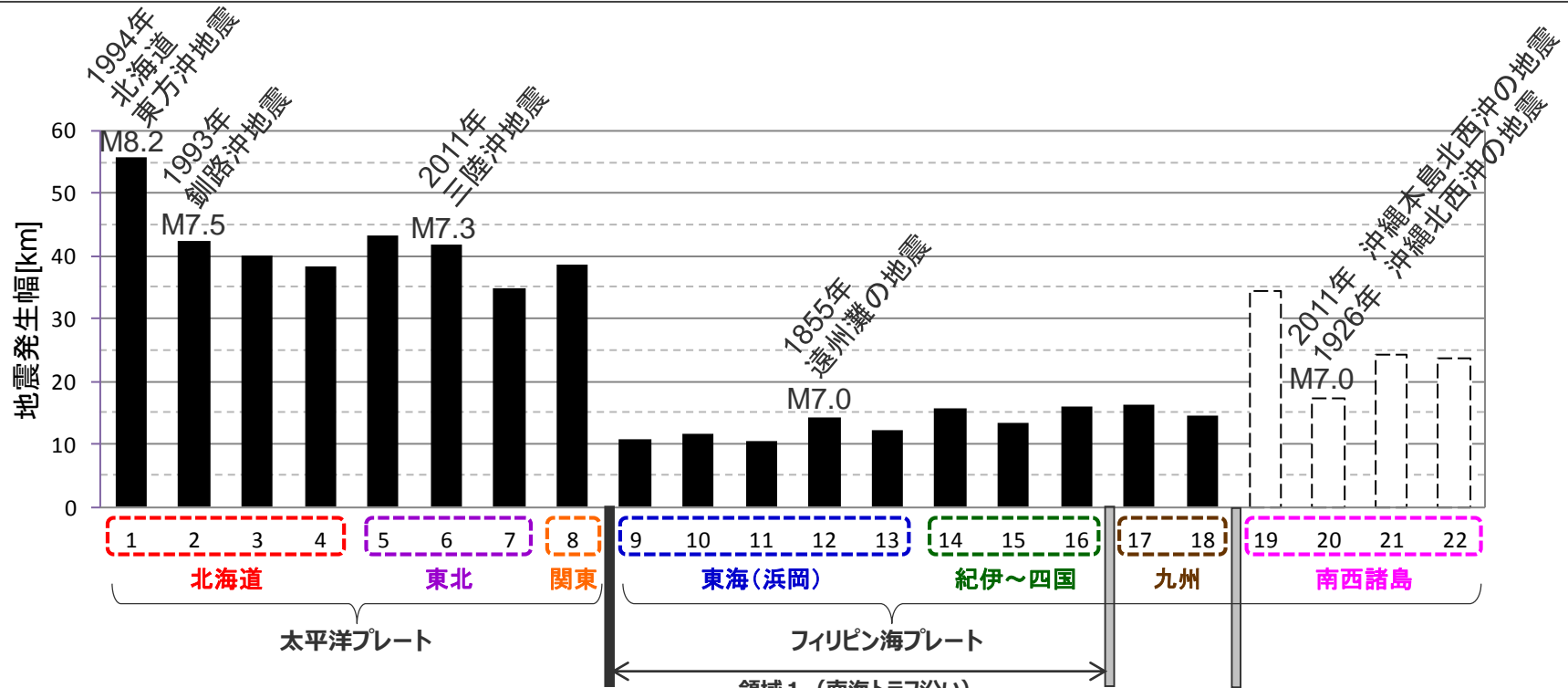
<日本周辺の地震発生層の幅>
