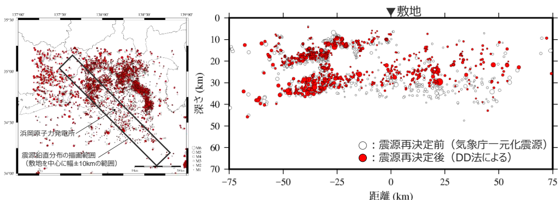
<第482回審査会合資料2-1で提示した震央分布及び震源鉛直分布> データ期間:1997年10月～2013年7月、震源の数:10,836個、走時の数:1,957,494本
