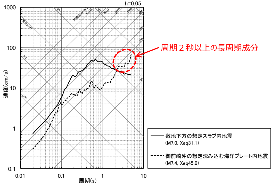
<Noda et al.(2002)による地震動評価結果の比較>
