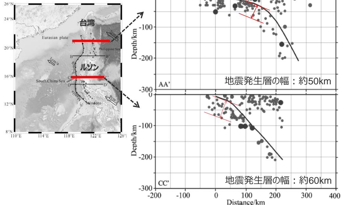
<台湾南西部及びルソン島西部における地震発生層の幅> (Gao et al.(2012)に地域名称、測線位置、地震発生層の幅の位置を加筆)
