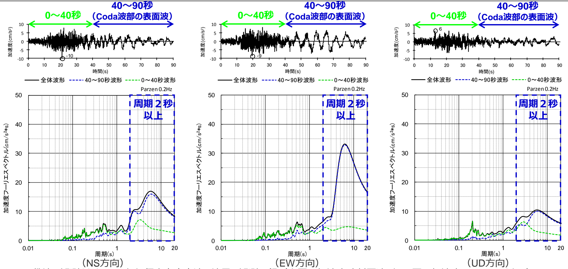
<敷地で観測された2004年紀伊半島南東沖の地震の観測記録（上図：加速度時刻歴波形、下図：加速度フーリエスペクトル）>
