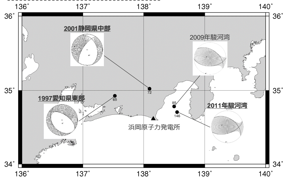
<敷地周辺で発生した地震のCMT解>
