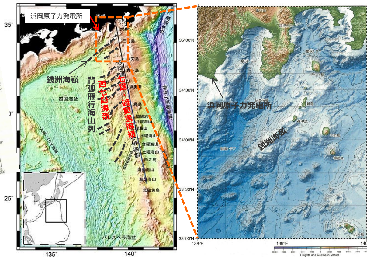
<伊豆小笠原島弧の地形>
