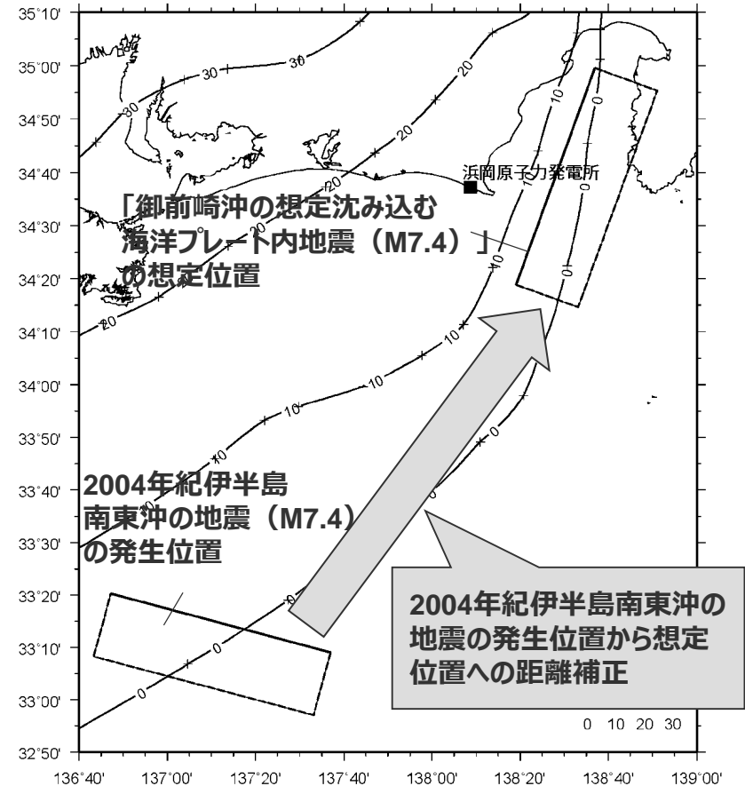
<2004年紀伊半島南東沖の地震の距離補正のイメージ>
