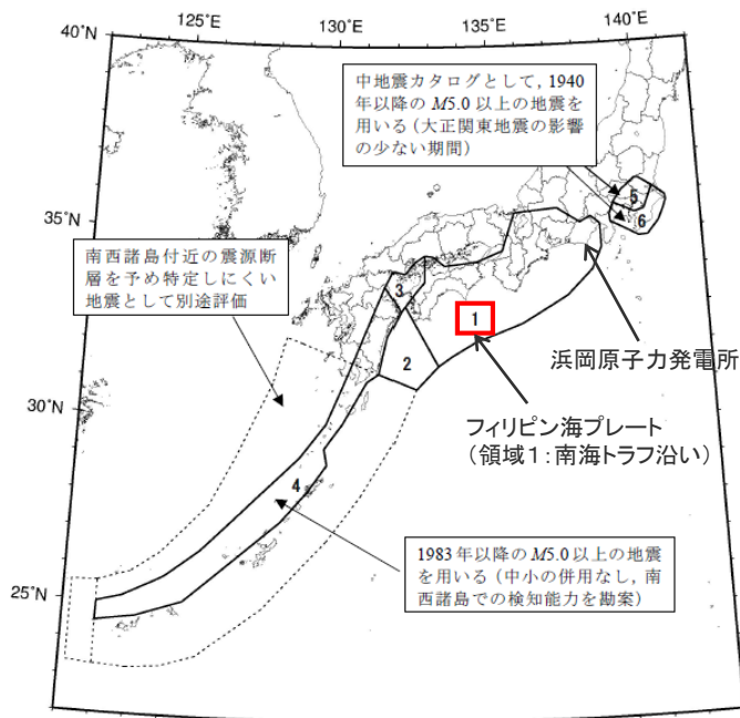
<震源を予め特定しにくい地震の地域区分> (地震調査委員会(2009)に敷地位置、領域の説明、赤い四角を加筆)
