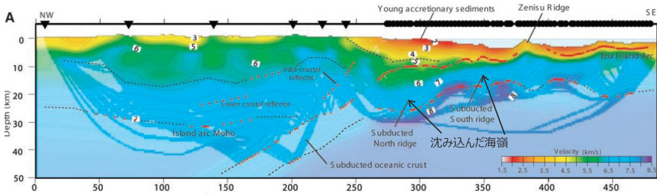
<遠州灘のP波速度構造 (Kodaira et al(2009)に敷地位置、沈み込んだ海嶺の位置を加筆>
