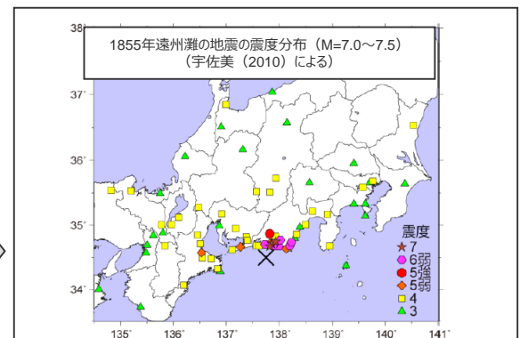
宇佐美 (2010) の震度分布に相対震度を考慮した補正震度をターゲットとし、作成した震度距離減衰式を用いてMを再推定
