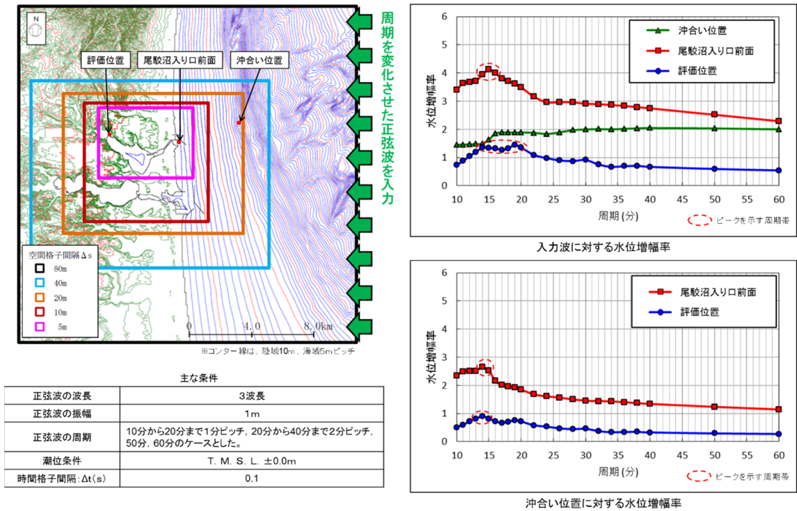
第 17 図 正弦波入力による検討結果
