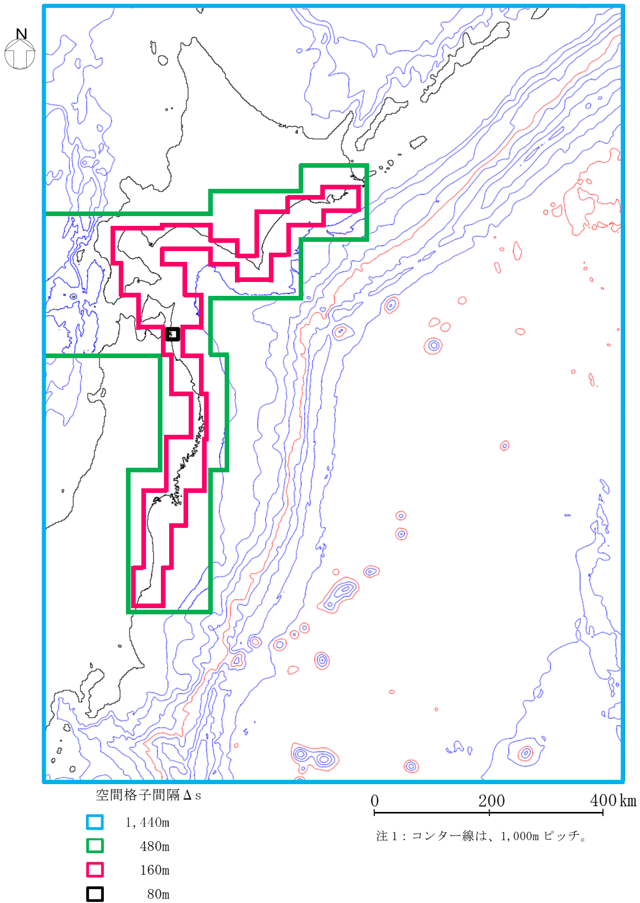
第5図 計算領域とその水深及び格子分割
