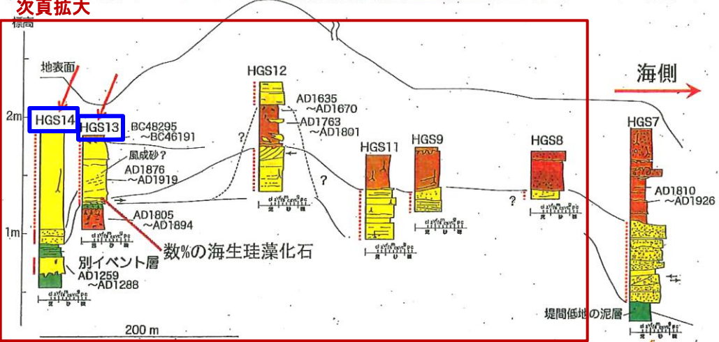
柱状断面図2
