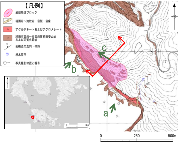
地質踏査の結果想定される岩盤崩壊土塊 (LsO-44)
