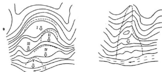
多丘形凸状台地状地形
