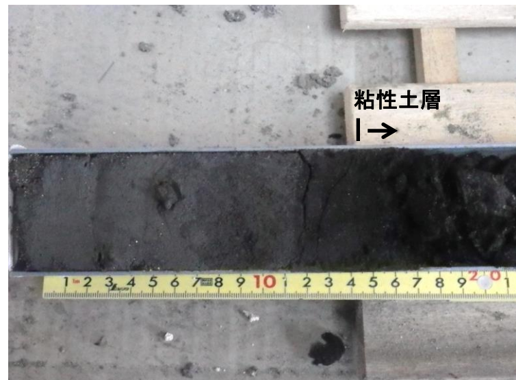
SS-4-①(-3.0~-3.2m)
