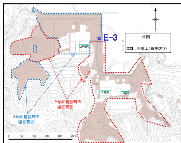
敷地平面図
