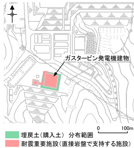
埋戻土(購入土) 分布範囲
