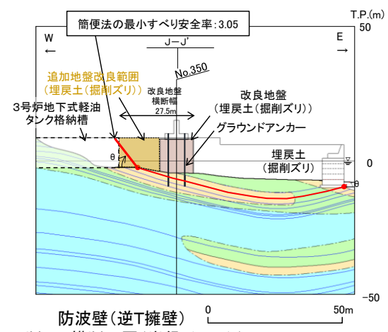
防波壁(逆T擁壁) 縦断面図(岩級・シーム)
