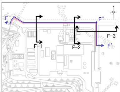
断面位置図
