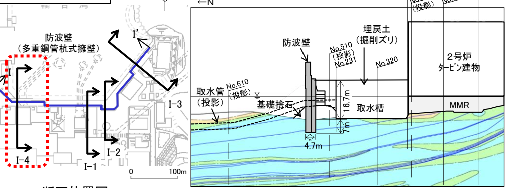
断面位置図
