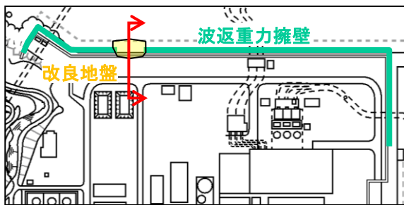
位置図
