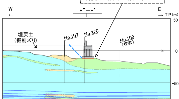
防波壁(波返重力擁壁) F-3断面横断面図(岩級・シーム)
