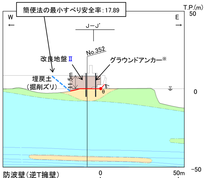
防波壁(逆T擁壁) ⑨-⑨'断面 横断面図(岩級・シーム)
