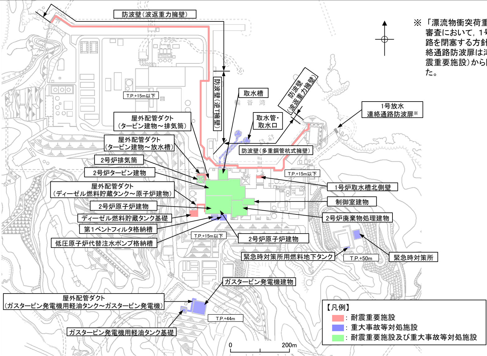
評価対象施設配置図
