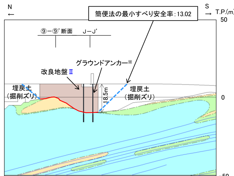
防波壁(逆T擁壁) ⑩-⑩'断面 横断面図(岩級・シーム)
