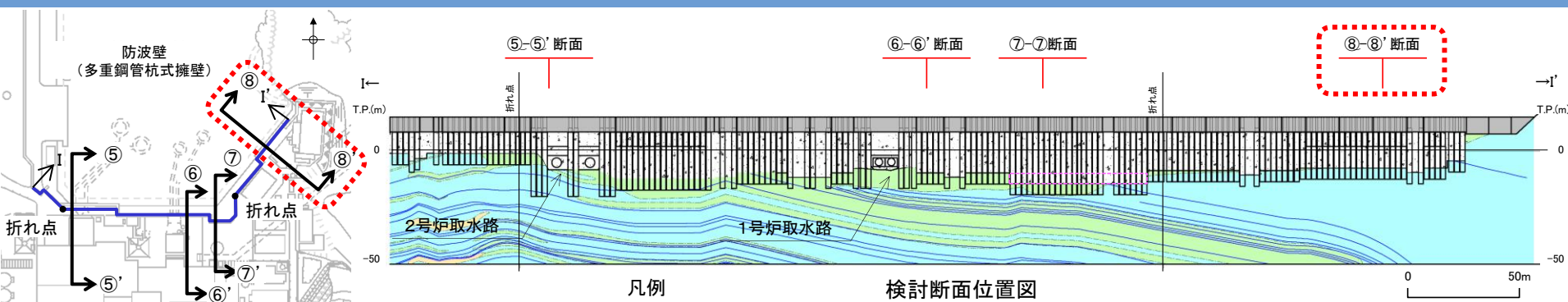
断面位置図
