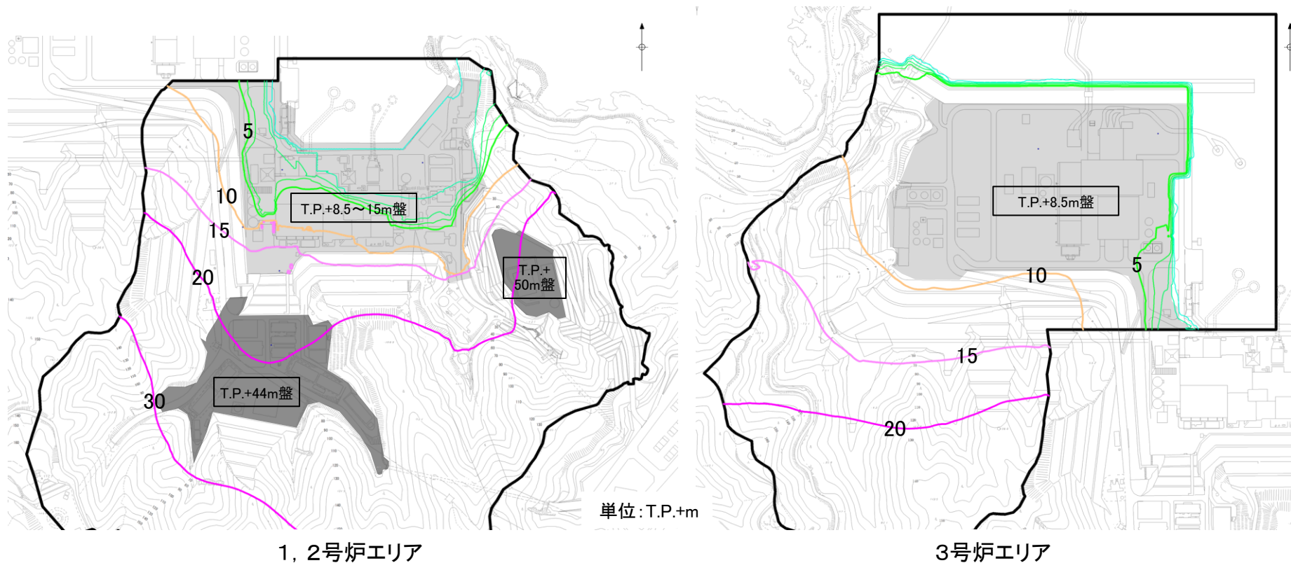
3次元浸透流解析結果(定常解析)の等水位線図 (解析条件は補足説明12章を参照)
