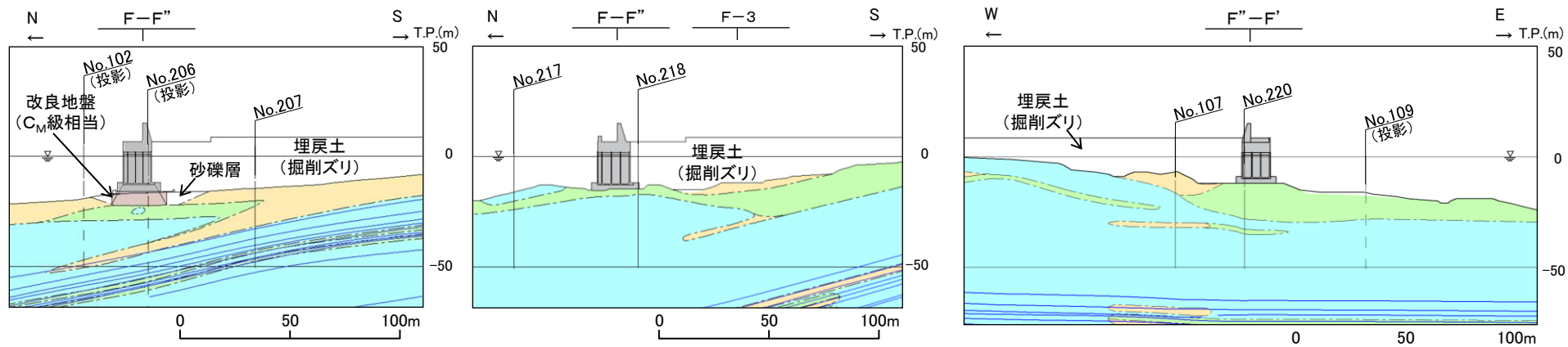
防波壁(波返重力擁壁)
