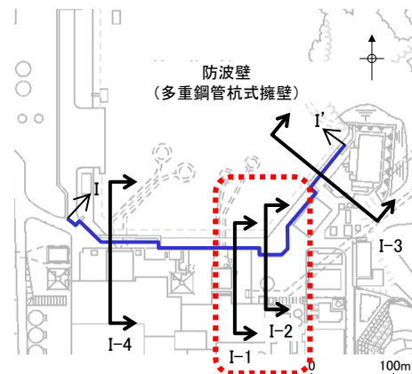
断面位置図
