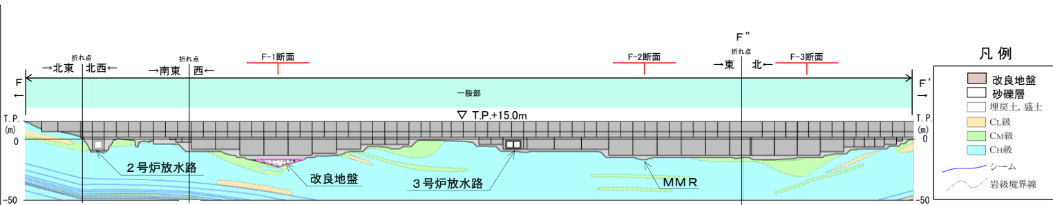
防波壁縦断面図(波返重力擁壁)
