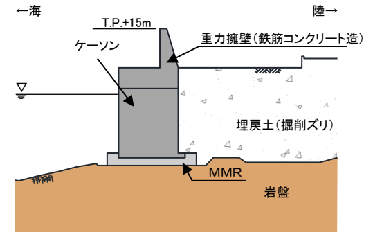
防波壁(波返重力擁壁(岩盤部))標準断面図
