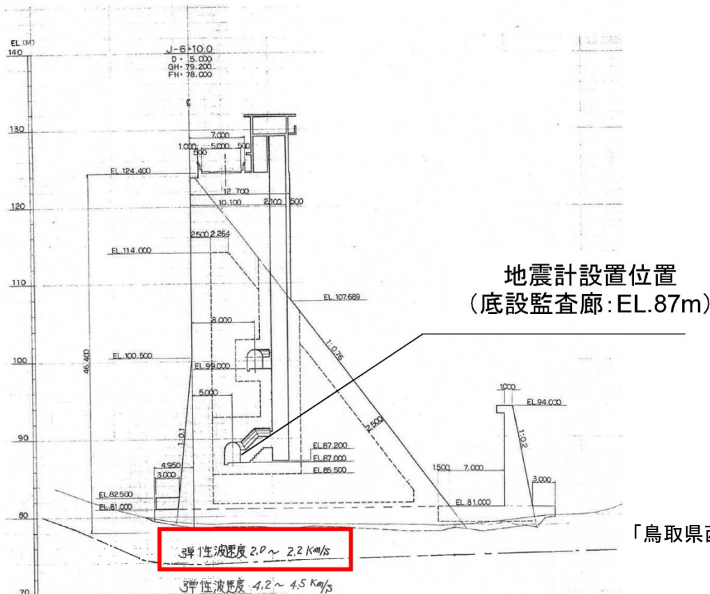
ダム断面図
