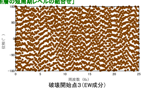
基準地震動S s -D及び選定した断層モデル手法による地震動評価結果のフーリエ位相スペクトルの比較【水平方向】
