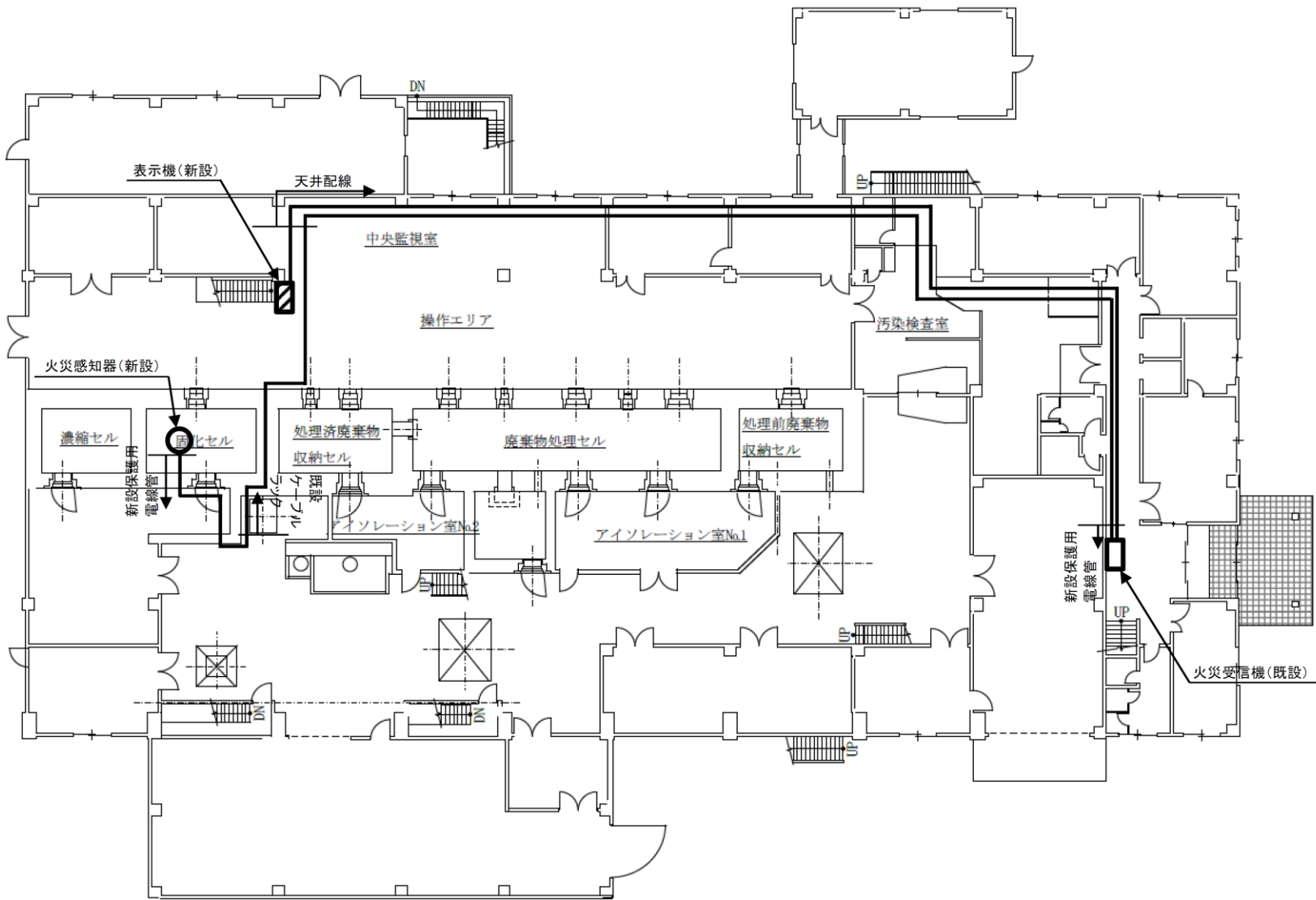
配線敷設図(概略)
