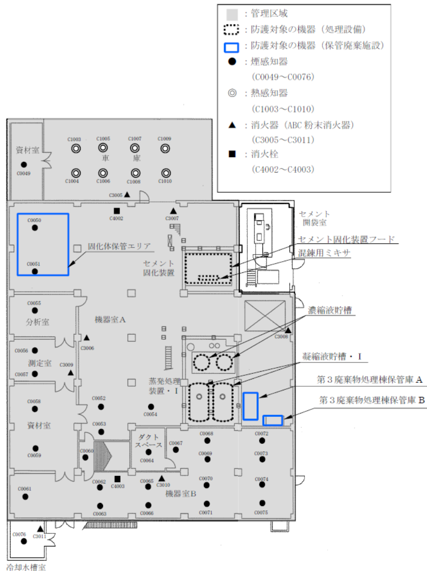
第3廃棄物処理棟における火災感知設備及び消火設備の設置場所(1階)
