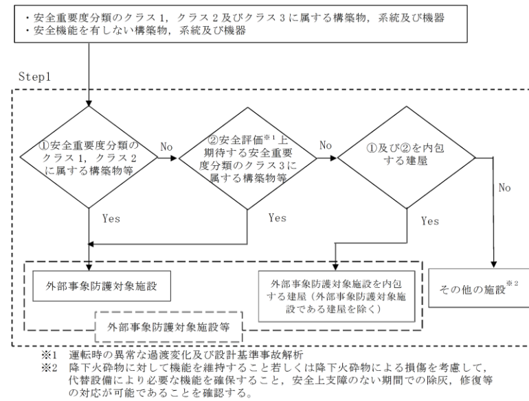
第 3.3-1 図 外部事象防護対象施設等の抽出フロー
