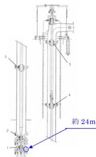
第4図 残留熱除去系海水系ポンプ 断面図
