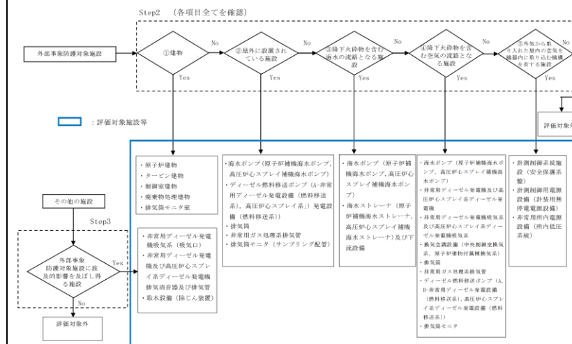
第 1.3-1 図 外部事象防護対象施設評価フロー
