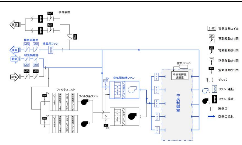
第5図 中央制御室換気空調設備(通常運転) 概要図
