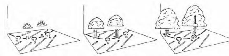
図2.1.4 局地前線に伴う竜巻の発生機構に関する模式図 (上向き黒い⇒が上昇気流を表す)
