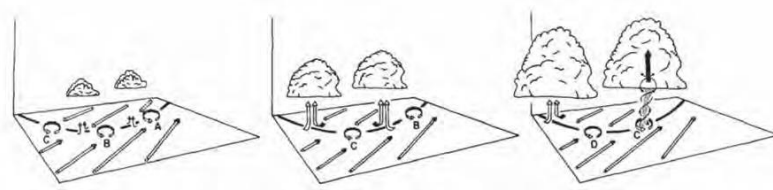
図5 局地前線に伴う竜巻の発生機構に関する模式図 (Wakimoto and Wilson 1989) (上向き黒い⇒が上昇気流を表す)
