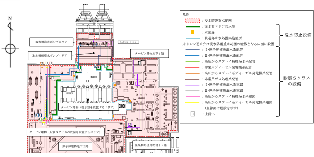
第 2.4-3 図 タービン建物地下1階の復水器エリア防水壁等の浸水防止設備と耐震Sクラスの設備の位置
