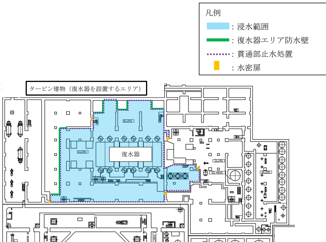
第4.2-9図 復水器エリア水密扉 設置位置
