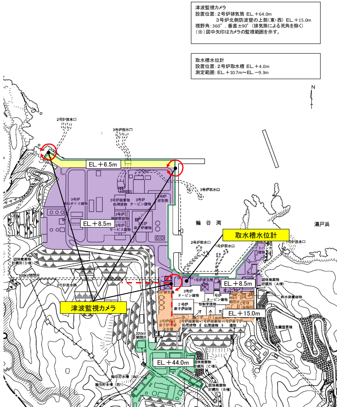
第4.3-1図 津波監視設備の配置
