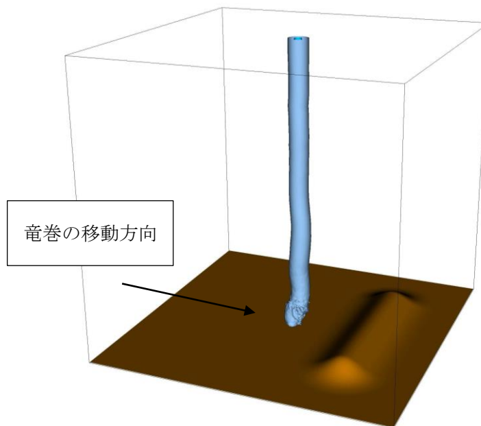
図 2.4.2 数値シミュレーションのセットアップ
