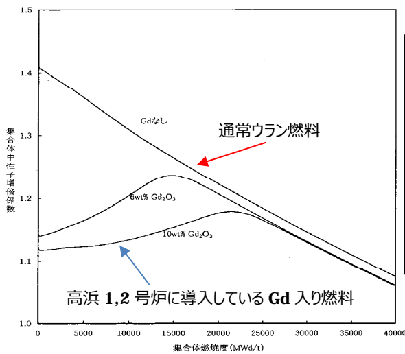
第 1 図 ※1 通常ウラン燃料と Gd 入り燃料の反応度（中性子増倍率） （15×15 型 20 本 Gd ウラン燃料棒 4.6wt% 235 U）
