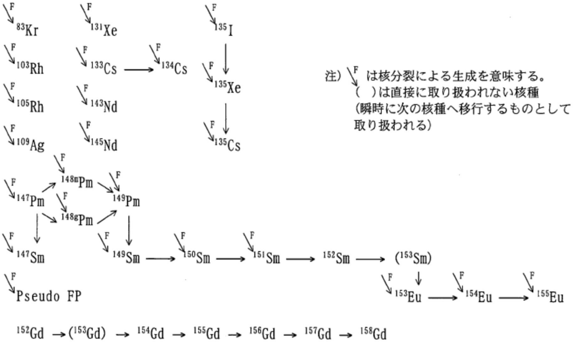
第 2 図 PHOENIX-P 燃焼計算で取り扱われる AC/FP 核種燃焼チェーン
