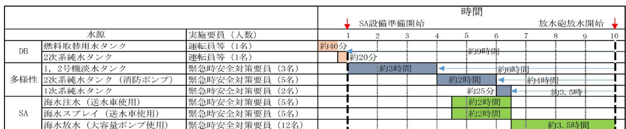
第14図 全手順同時実施を想定したタイムチャート
