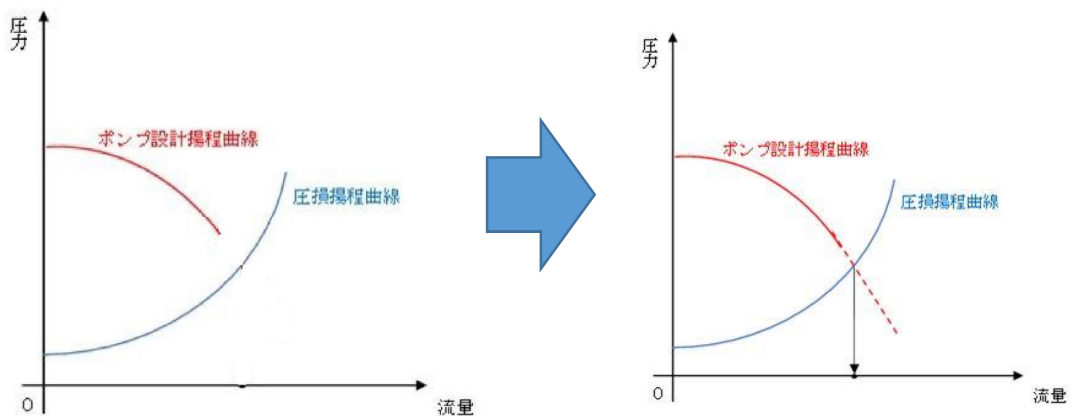
第2図 ポンプ揚程曲線および圧損揚程曲線を用いた流量設定の概要
