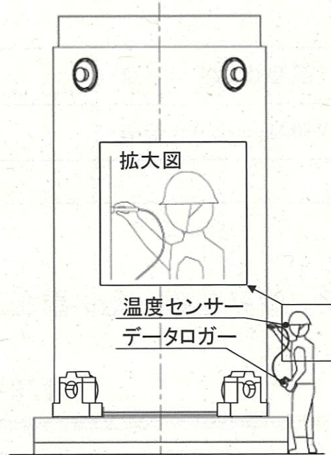
使用済燃料乾式貯蔵容器表面温度計
