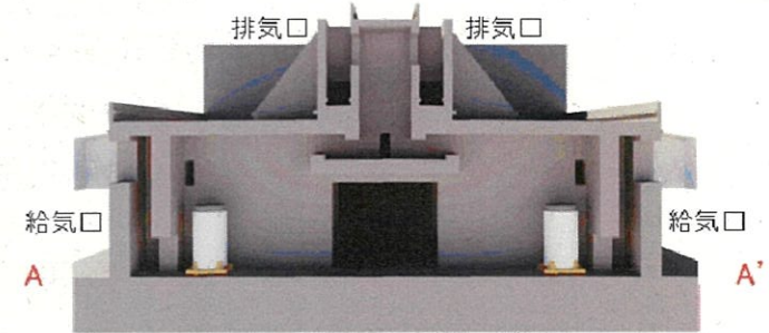
断面図(A-A')
