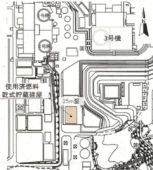
配置図
