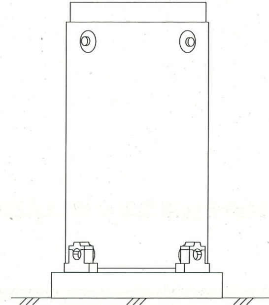
乾式キャスク概要図
