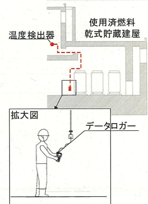
使用済燃料乾式貯蔵建屋内雰囲気温度計
