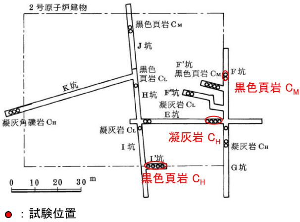
平板載荷試験位置図(2号試掘坑平面図)
