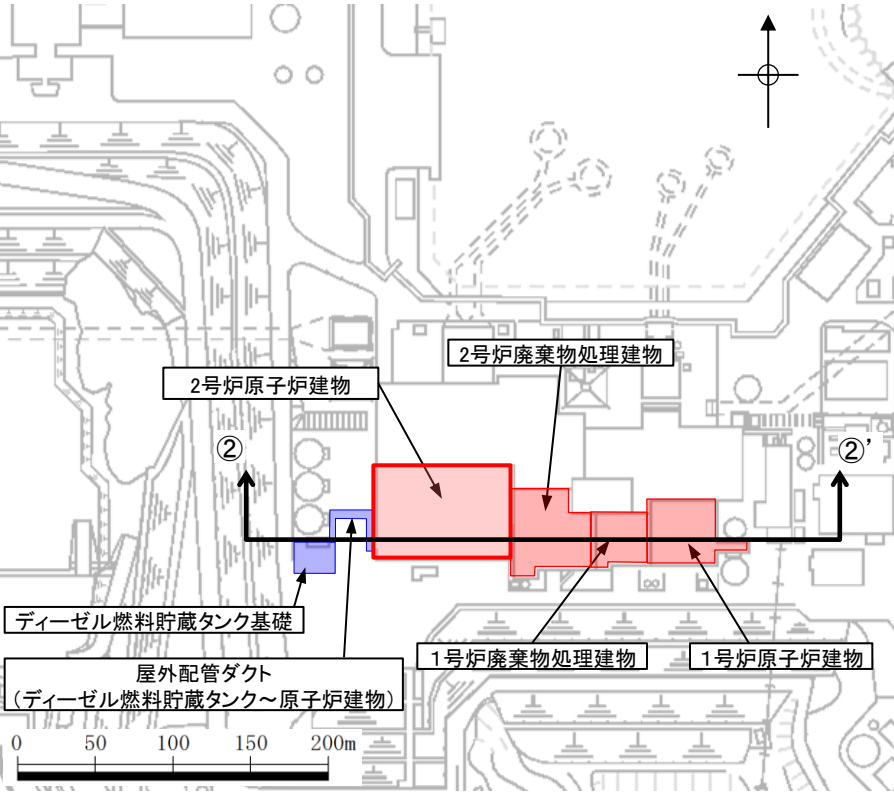
断面位置図
