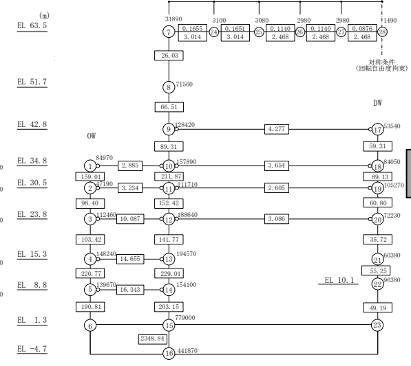
鉛直モデル
