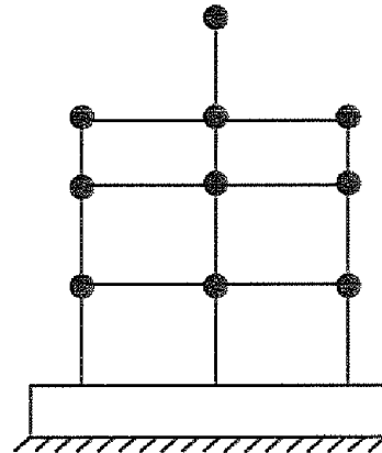
多質点系モデル(地盤バネ無) フロア毎に重量集約 層毎に剛性を集約 ・水平剛性 K_H ・鉛直剛性 K_V ・曲げ剛性 K_\phi
