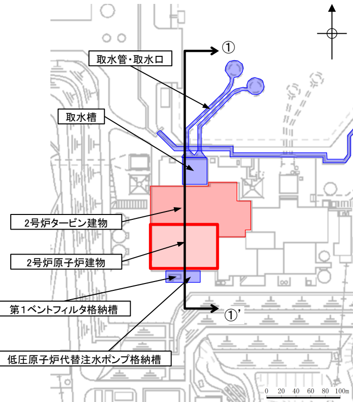
断面位置図
