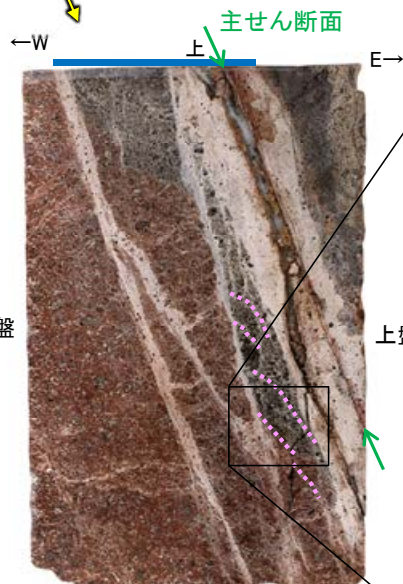
固結した破碎部 変形構造 研磨片写真(変形構造を加筆)
