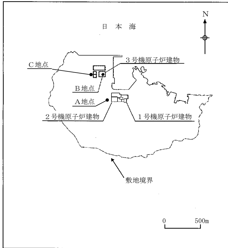
(a) 配置図
