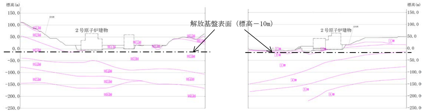
東西断面
