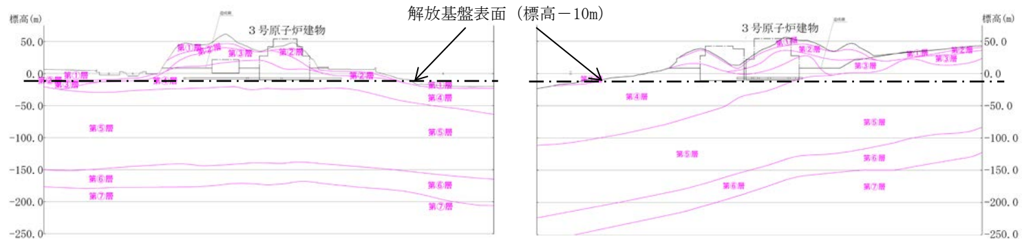
東西断面
