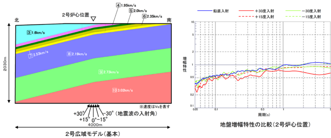
(a) 2号炉
