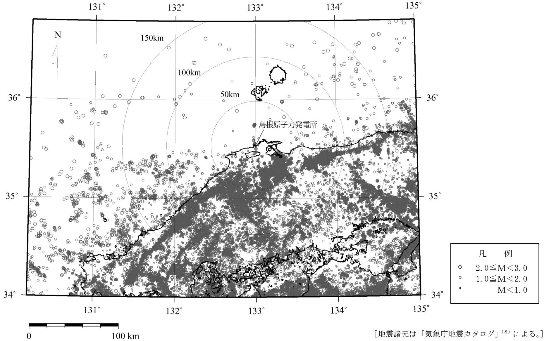
第 5.2-5 図 敷地周辺における地震 (M < 3) の震央分布 (1997 年 10 月 ~ 2016 年 10 月)
