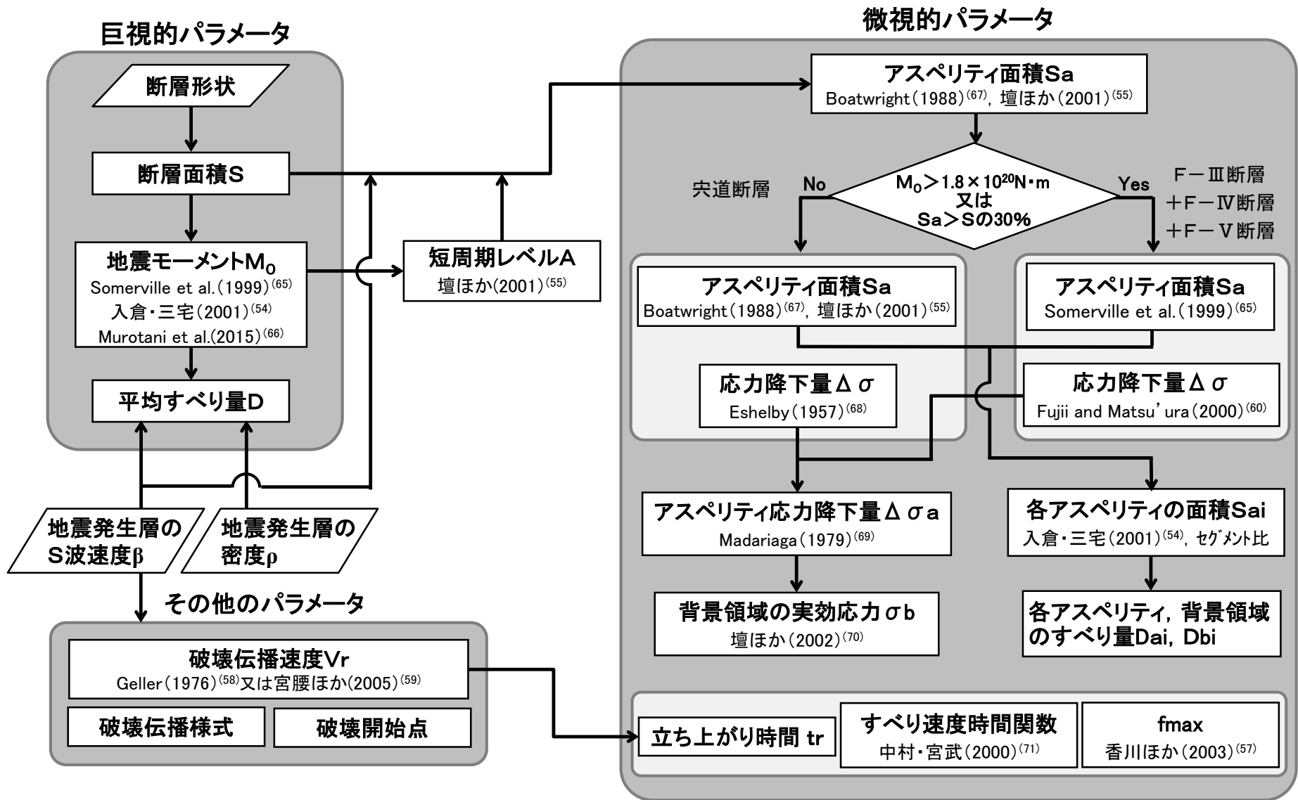
第 5.6-3 図 断層パラメータの設定フロー
