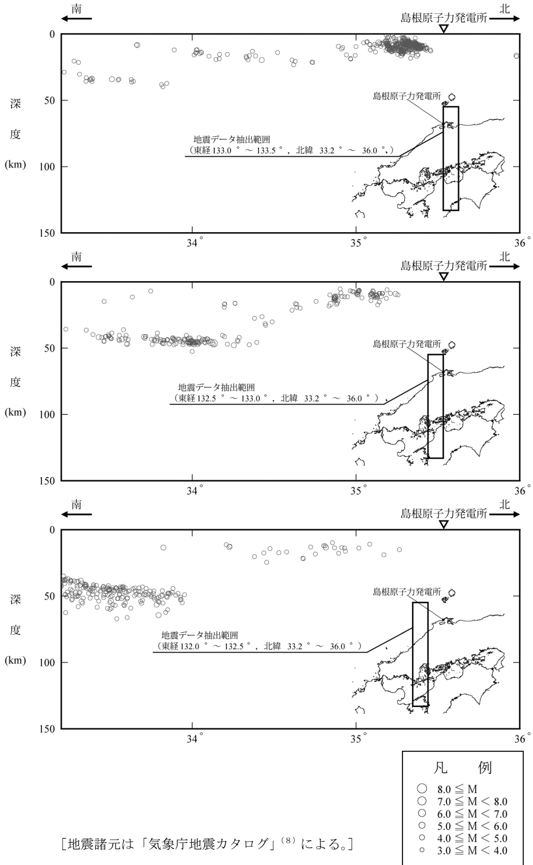
第 5.2-4 図 (1) 敷地周辺における地震 ( M \geq 3 ) の震源鉛直分布 (南北方向) (1997 年 10 月 ~ 2016 年 10 月)
