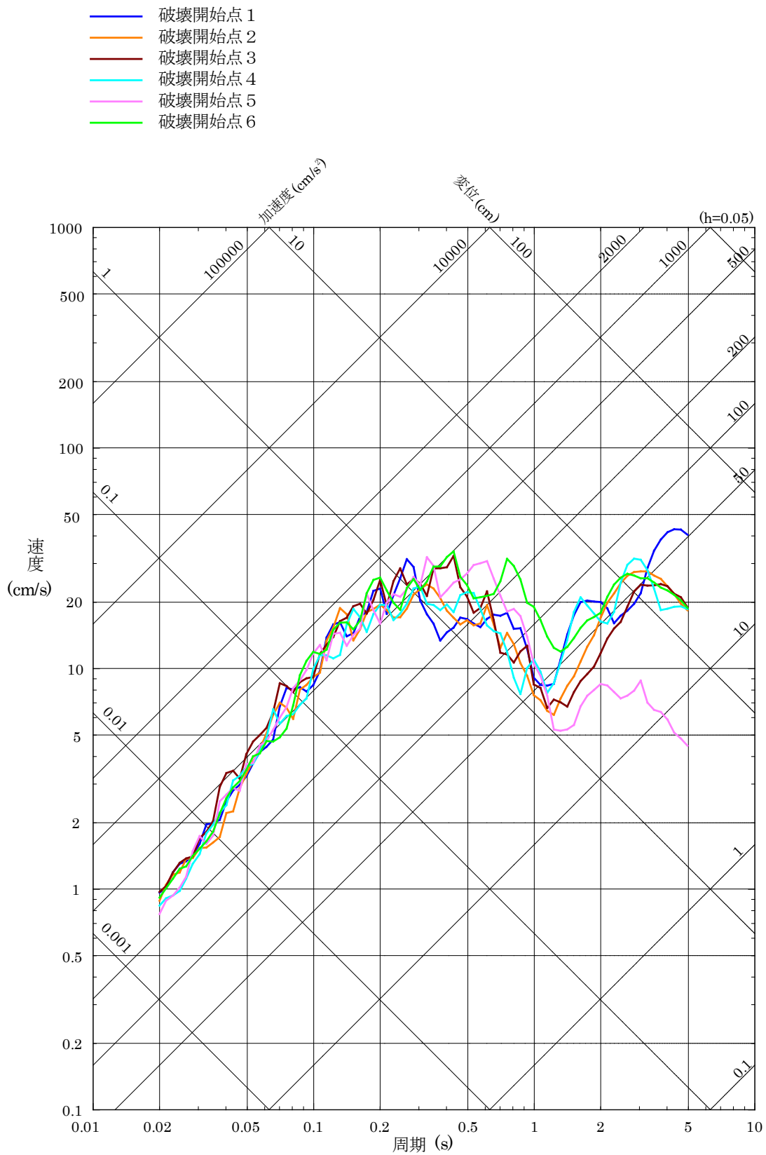
第 5.6-11 図 (16) 「F-III断層 + F-IV断層 + F-V断層による地震」の断層モデルを用いた手法による地震動評価結果 (鉛直方向) (断層位置の不確かさを考慮したケース)
