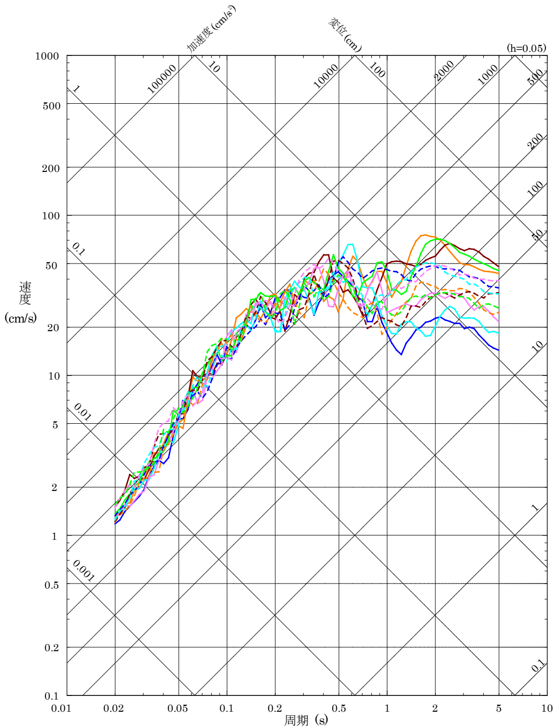
第 5.6-10 図(7) 「宍道断層による地震」の断層モデルを用いた手法による地震動評価結果（水平方向） （すべり角の不確かさを考慮したケース）
