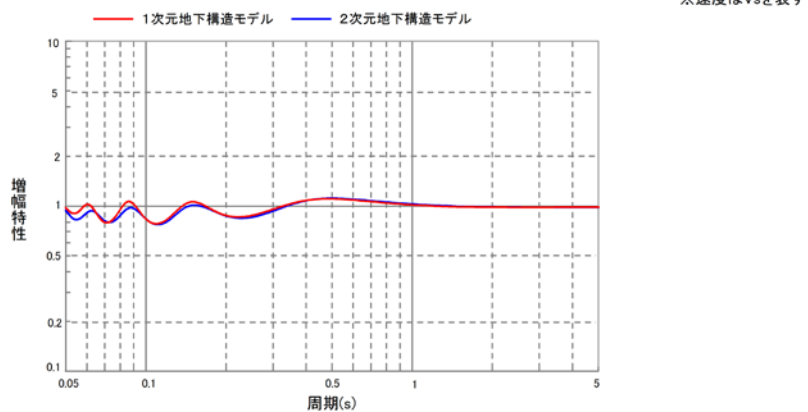
地盤増幅特性の比較
