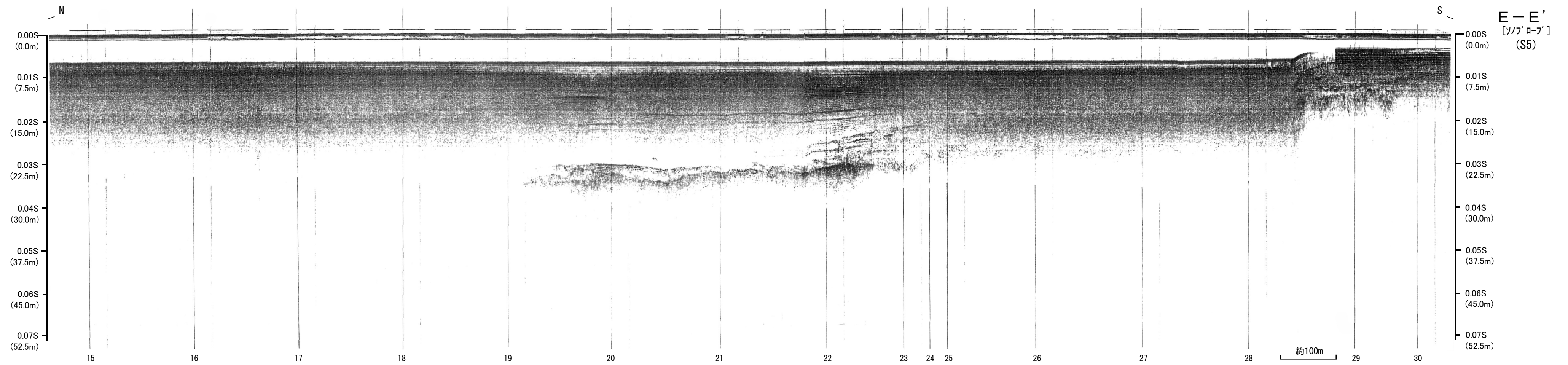
第3.2-9図(3) 宍道湖の音波探査記録(ソノプロブ・E-E')
