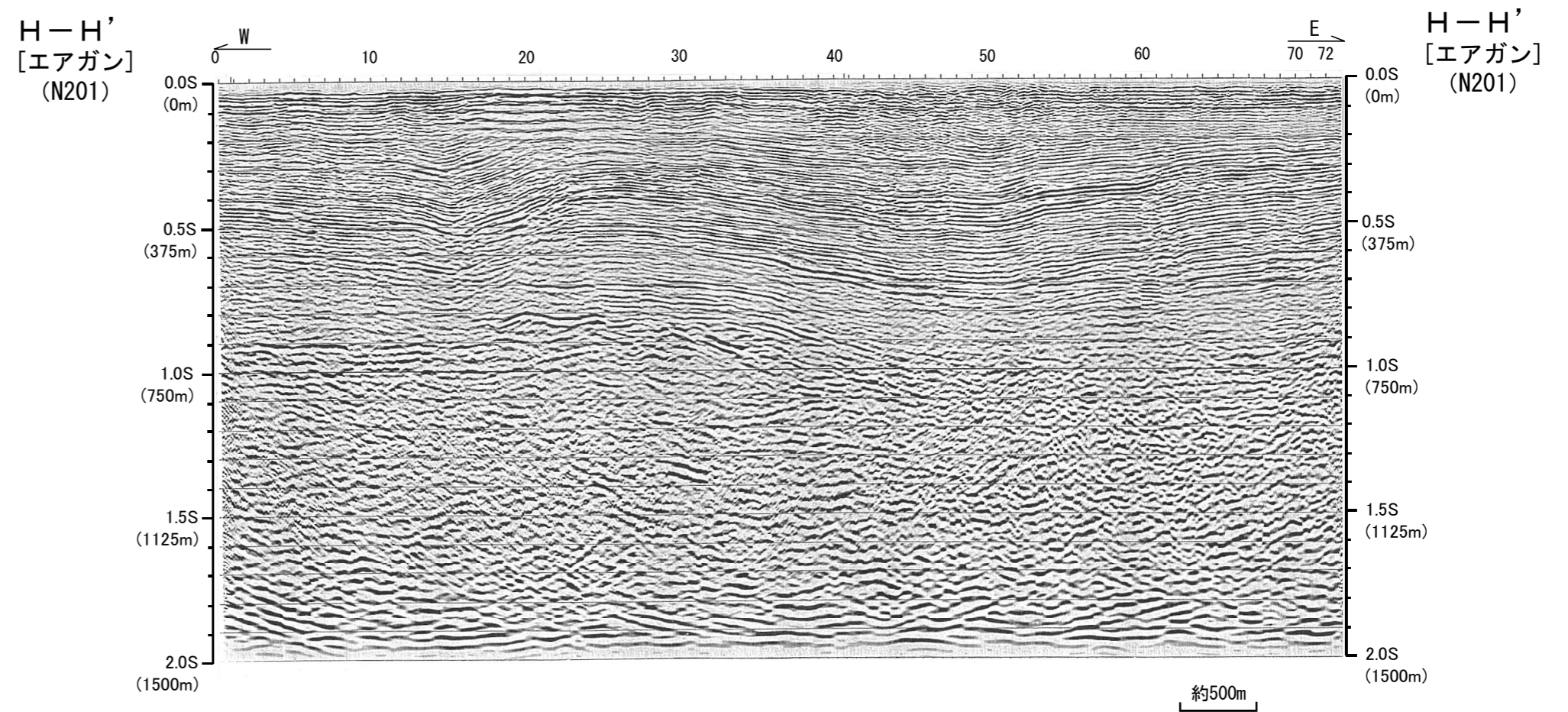
第3.2-10図(1) 中海の音波探査記録(エアガン・マルチチャンネル)
