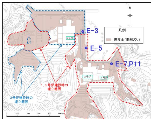
敷地平面図
