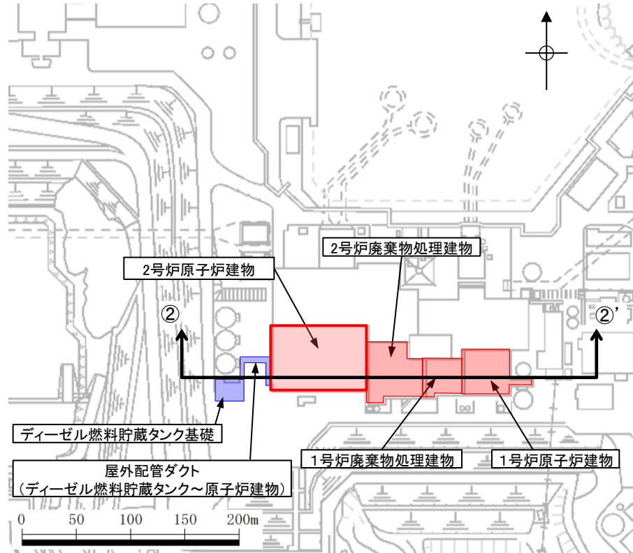
断面位置図
