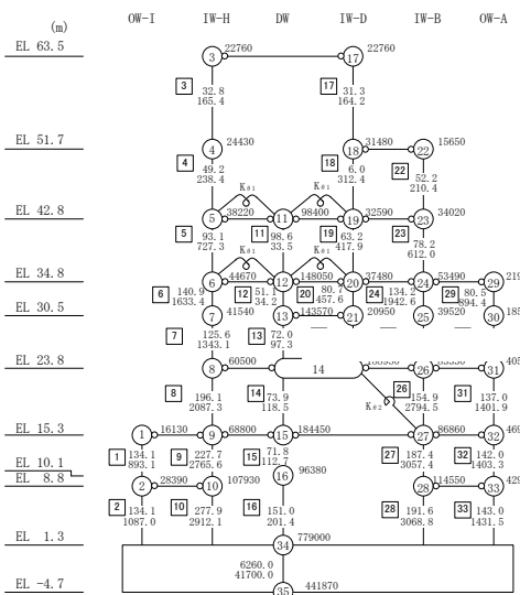
水平モデル(EW方向)
