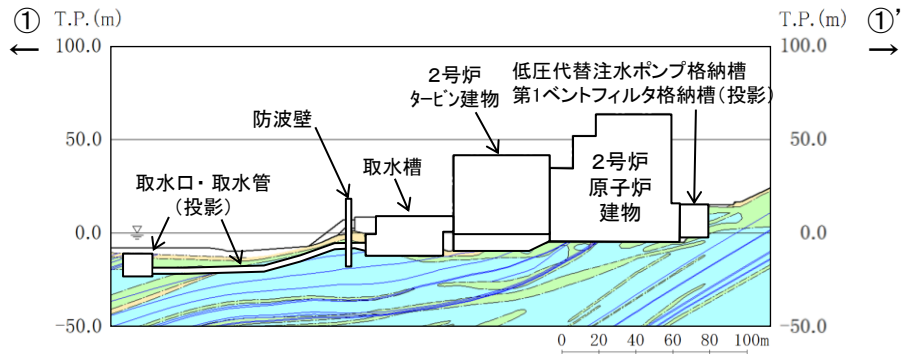
①-①' 断面図
