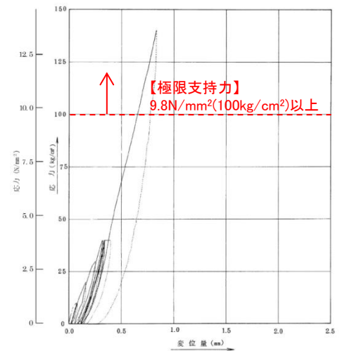
(b) 黑色頁岩 ( C_H 級)
