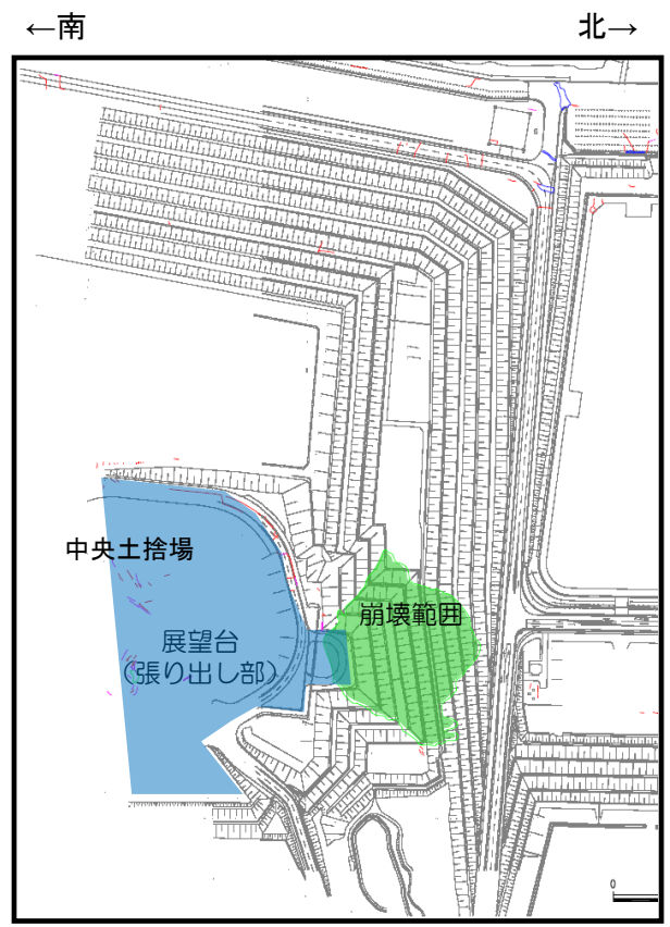
平面図
