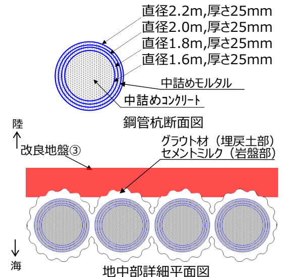
地中部詳細平面図
