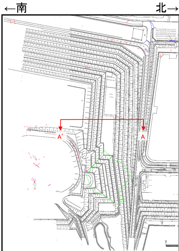
平面図
