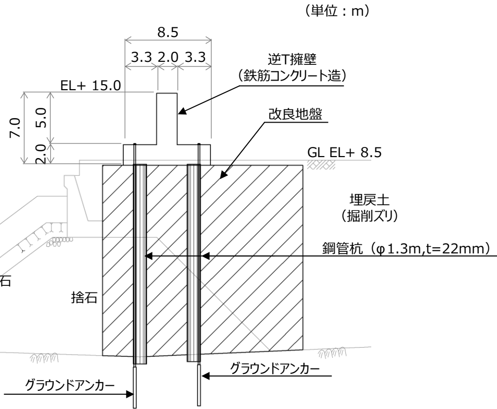
防波壁(鋼管杭式逆T擁壁)防波扉北側部(⑤-⑤断面) 断面図
