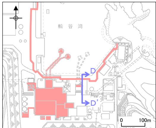
断面位置図 ■ : 評価対象施設
