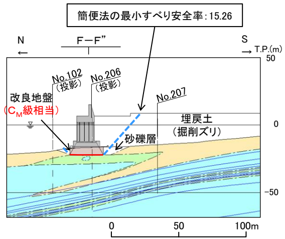
防波壁(波返重力擁壁) F-1断面横断面図(岩級・シーム)
