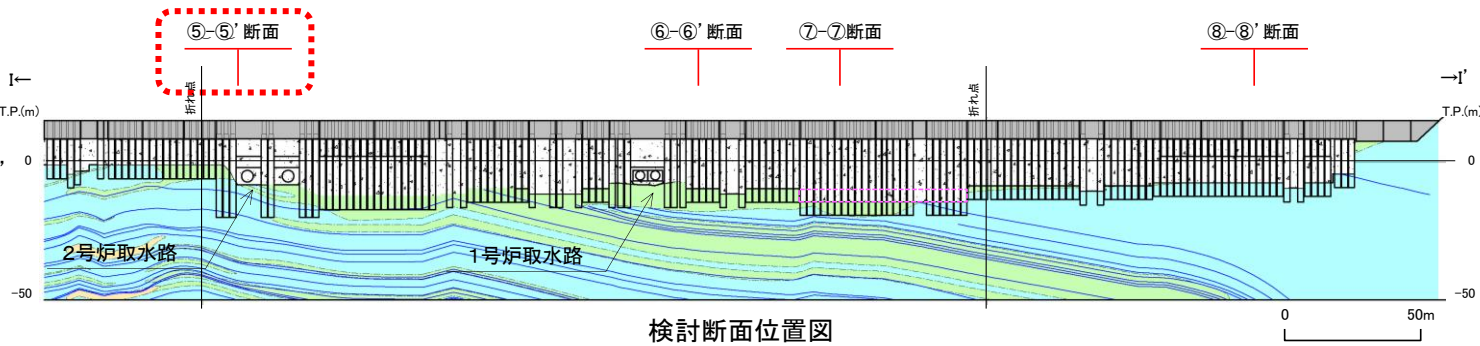
検討断面位置図
