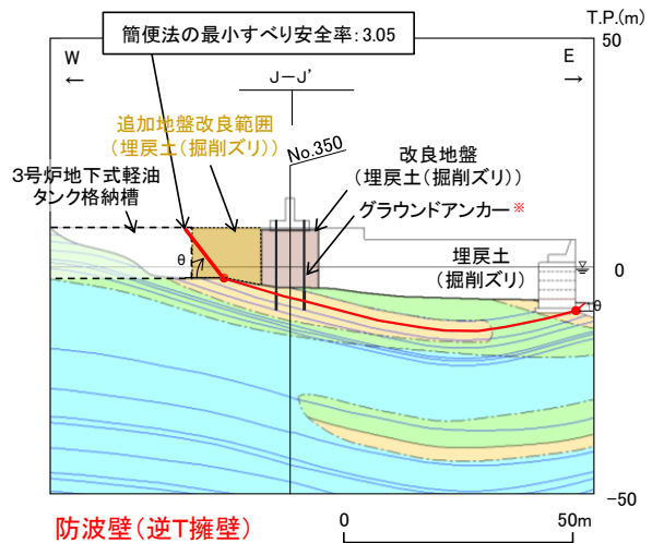
J-3断面 横断面図(岩級・シーム)
