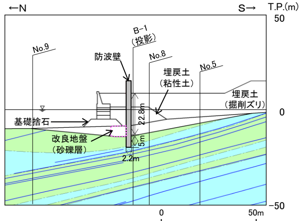
防波壁(多重鋼管杭式擁壁) I-2断面横断面図(岩級・シーム)
