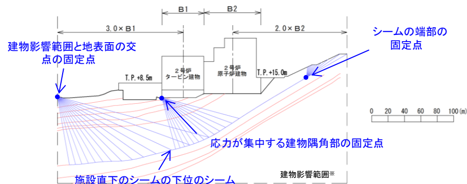
施設直下のシームの下位のシーム
