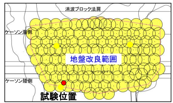
一軸圧縮試験実施箇所
