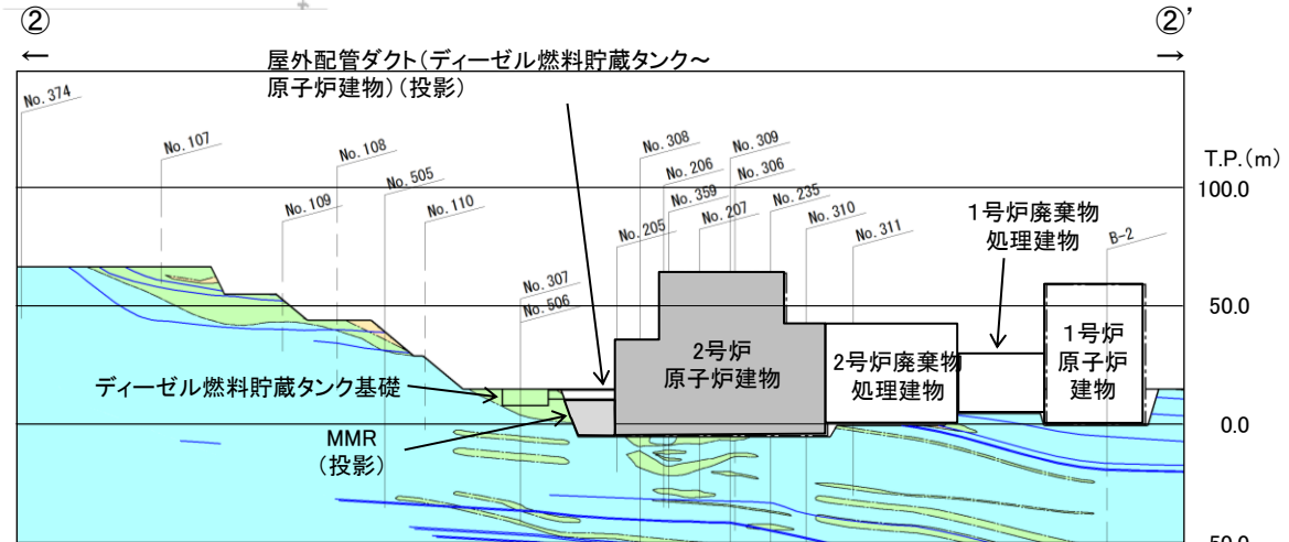
地質断面図(②-②'断面, 岩級・シーム)
