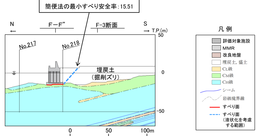
防波壁(波返重力擁壁) F-2断面横断面図(岩級・シーム)
