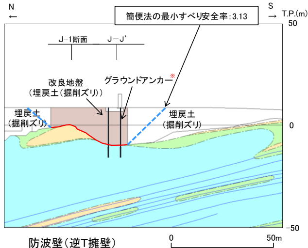
J-2断面 横断面図(岩級・シーム)
