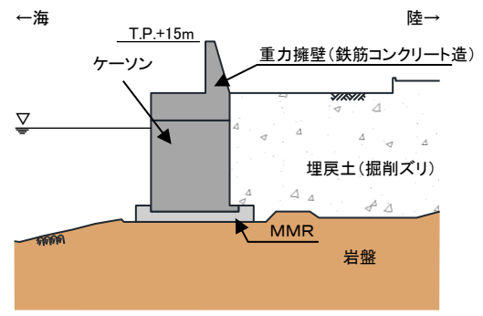
防波壁(波返重力擁壁(岩盤部))標準断面図
