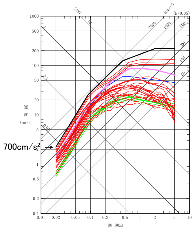
水平成分
