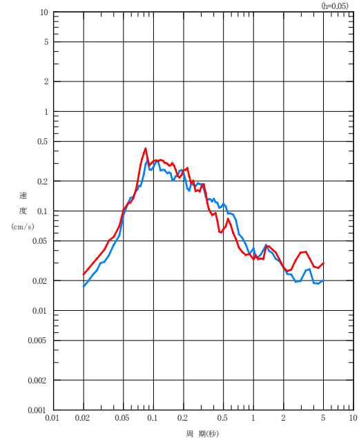
UD成分
