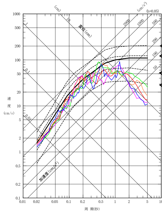
鉛直成分
