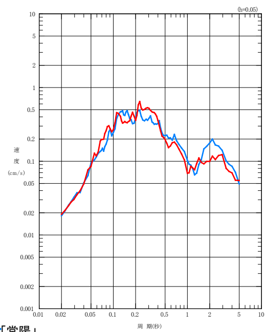
NS成分
