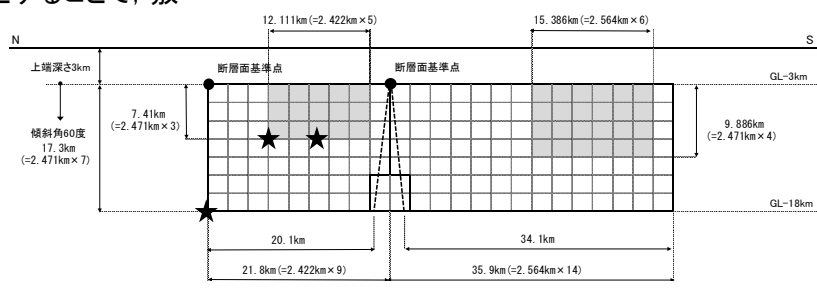
基本震源モデル
