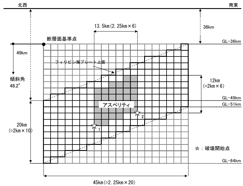
震源モデル
