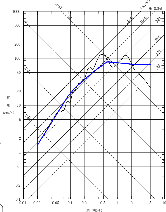
水平成分
