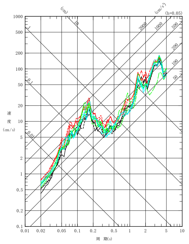
EW成分
