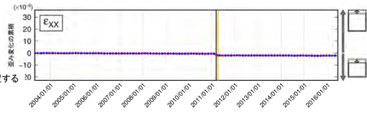
ひずみ変化の累積(大洗研敷地周辺)
