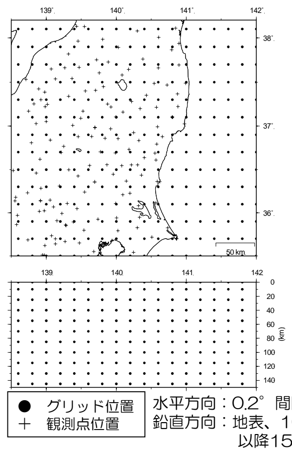
解析の範囲
