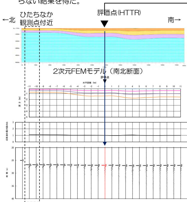
2次元FEMモデルへの模擬入力波(リッカー波)鉛直入射による各地点の時刻歴波形(南北断面)
