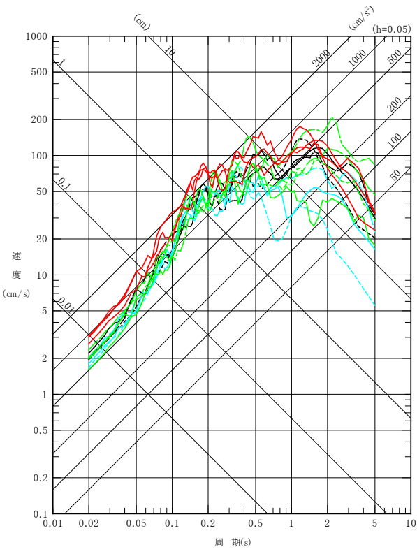
NS成分
