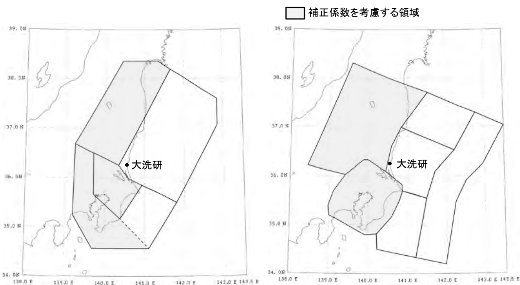
調査モデル
