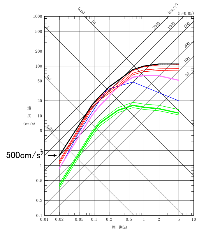
鉛直成分
