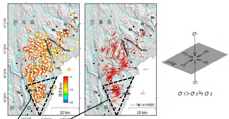
下図の三角形要素11を示す 図11 得られたメカニズム解とT軸の分布 左：下半球投影のメカニズム解。深さで色分けした。井戸沢断層(Ii)と湯ノ岳断層(Yn)の地表地震断層 (Mizoguchi et al., in preparation) を○で示す。中：メカニズム解のT軸方位 (水平投影)。右：推定される応力場の概念図。 青柳・上田(2012)に一部加筆
