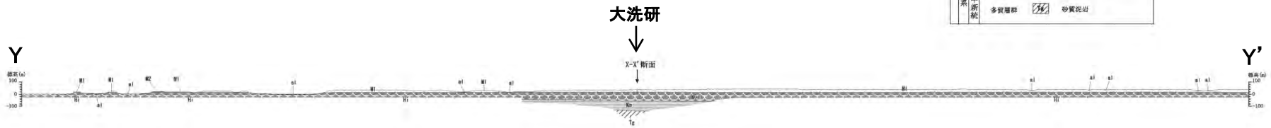
Y-Y' 断面
