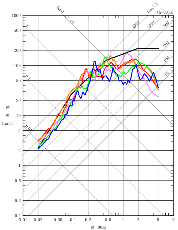
NS成分
