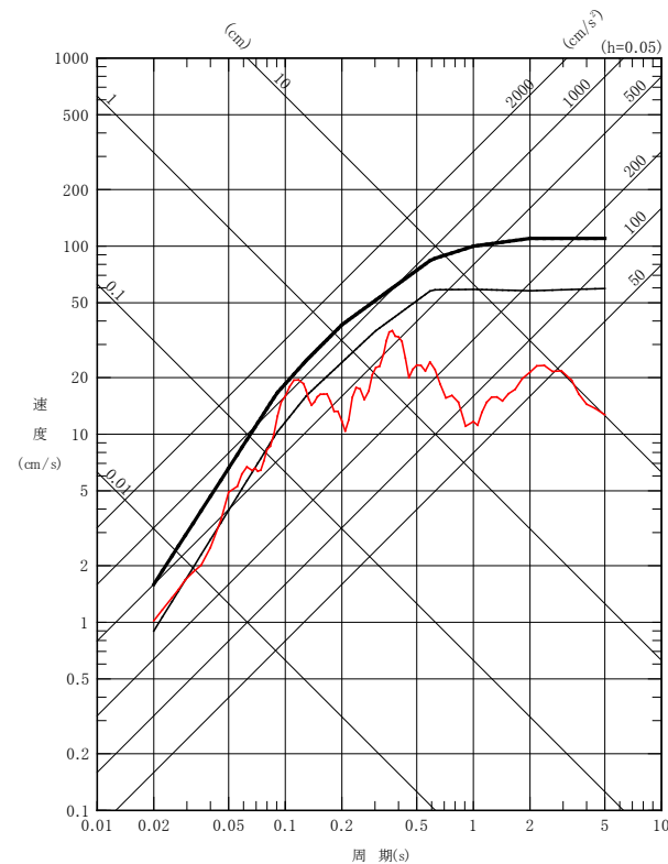
鉛直成分
