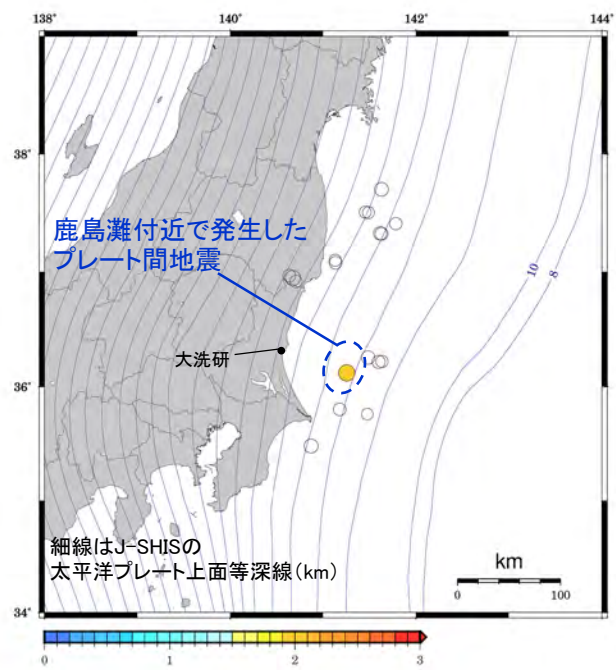
プレート間地震の震央分布図
