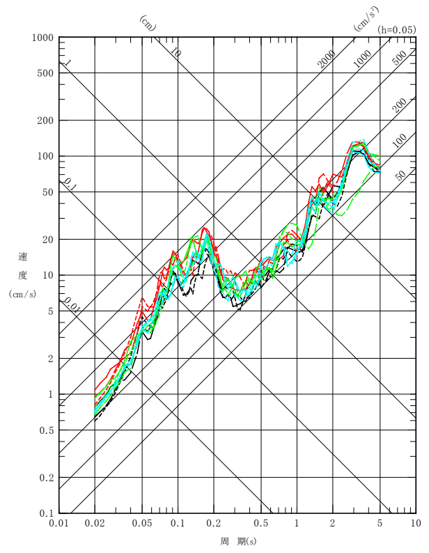
NS成分
