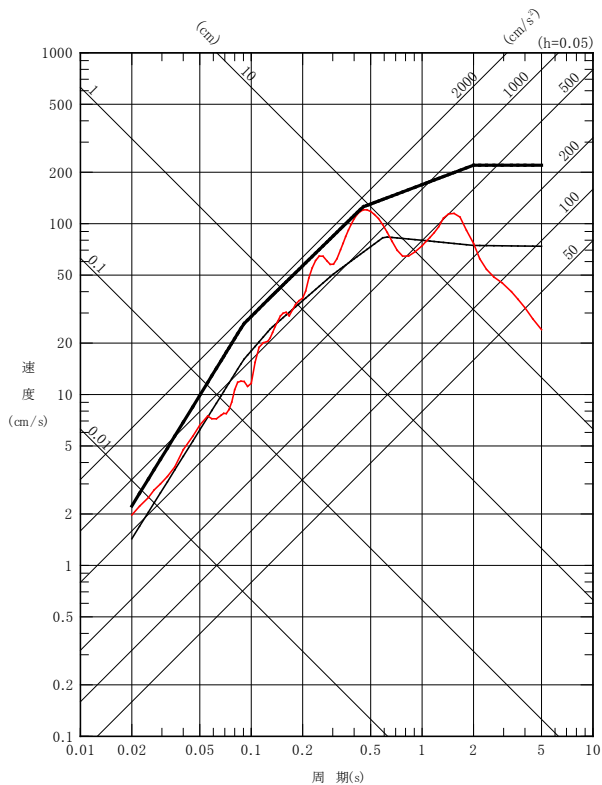
水平成分
