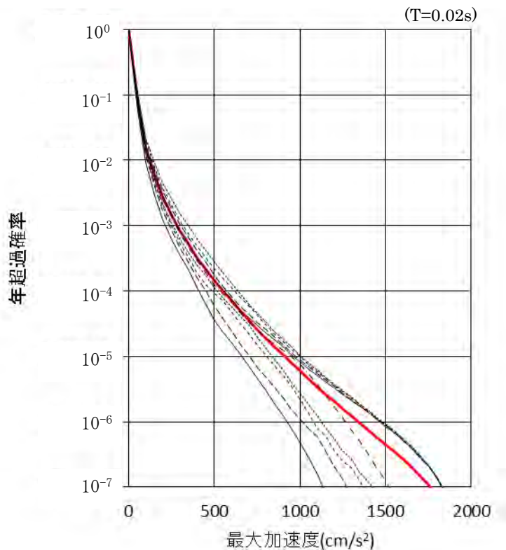
水平成分
