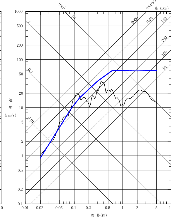
鉛直成分
