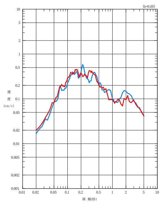
EW成分
