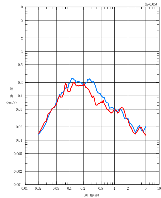
UD成分
