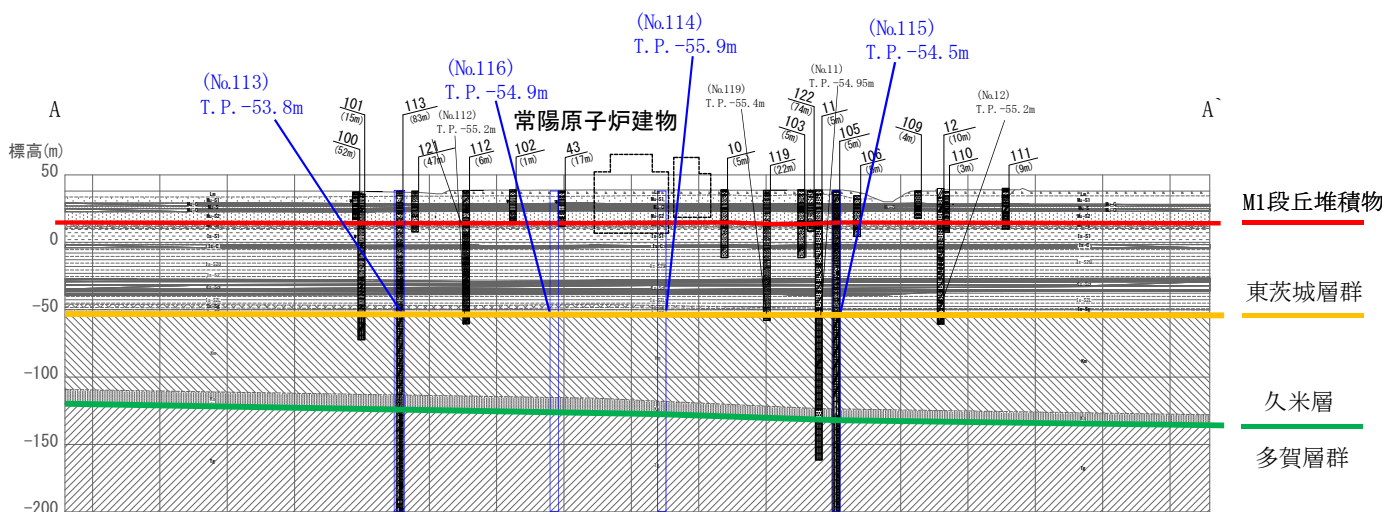
A-A' 測線（南北方向）
