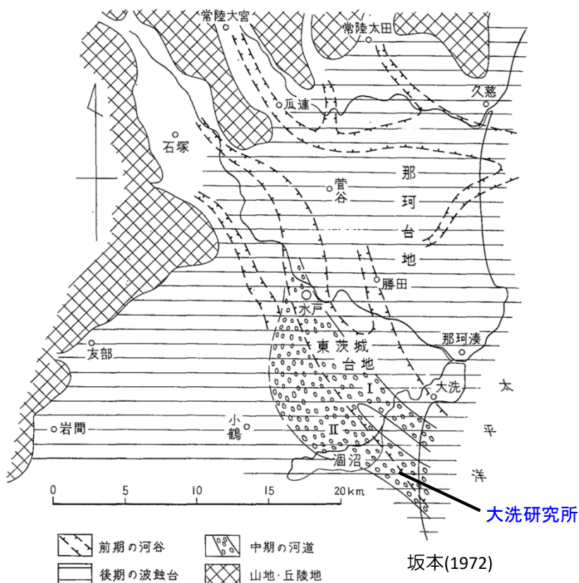
見和層堆積期の古地理
