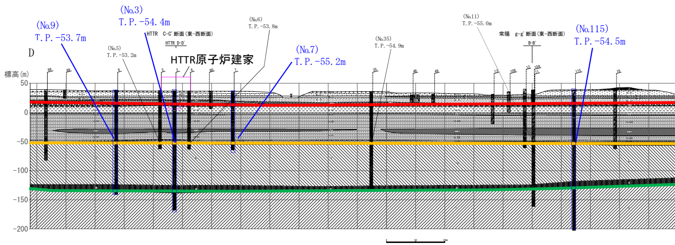
D-D' 測線（東西方向）
