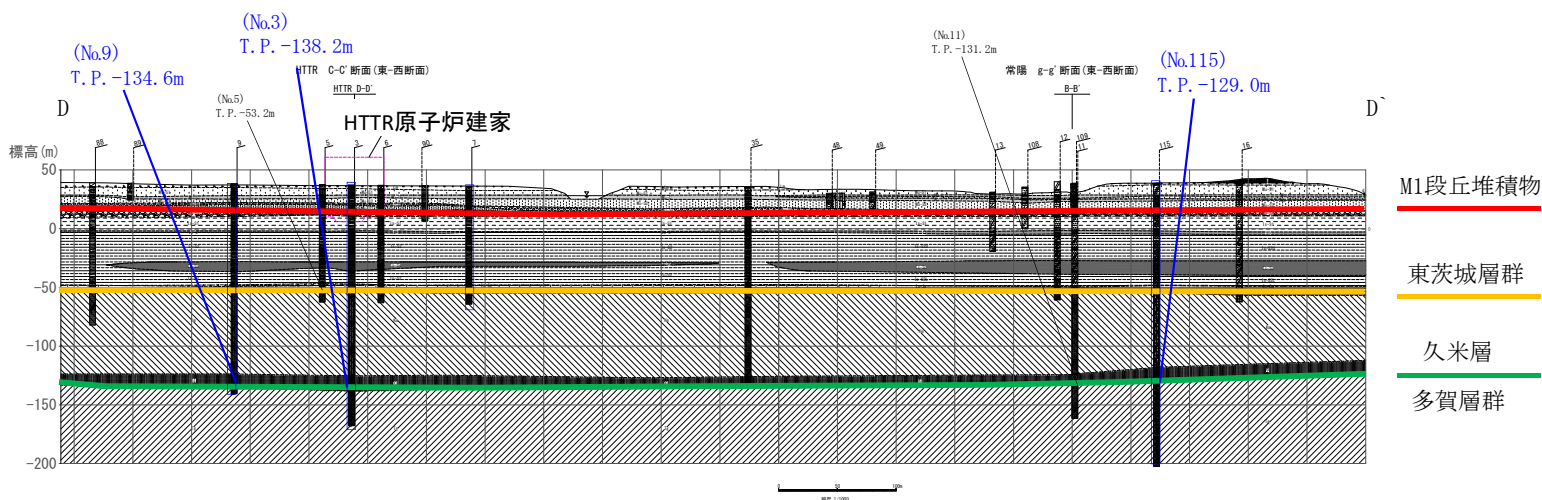
D-D' 測線（東西方向）
