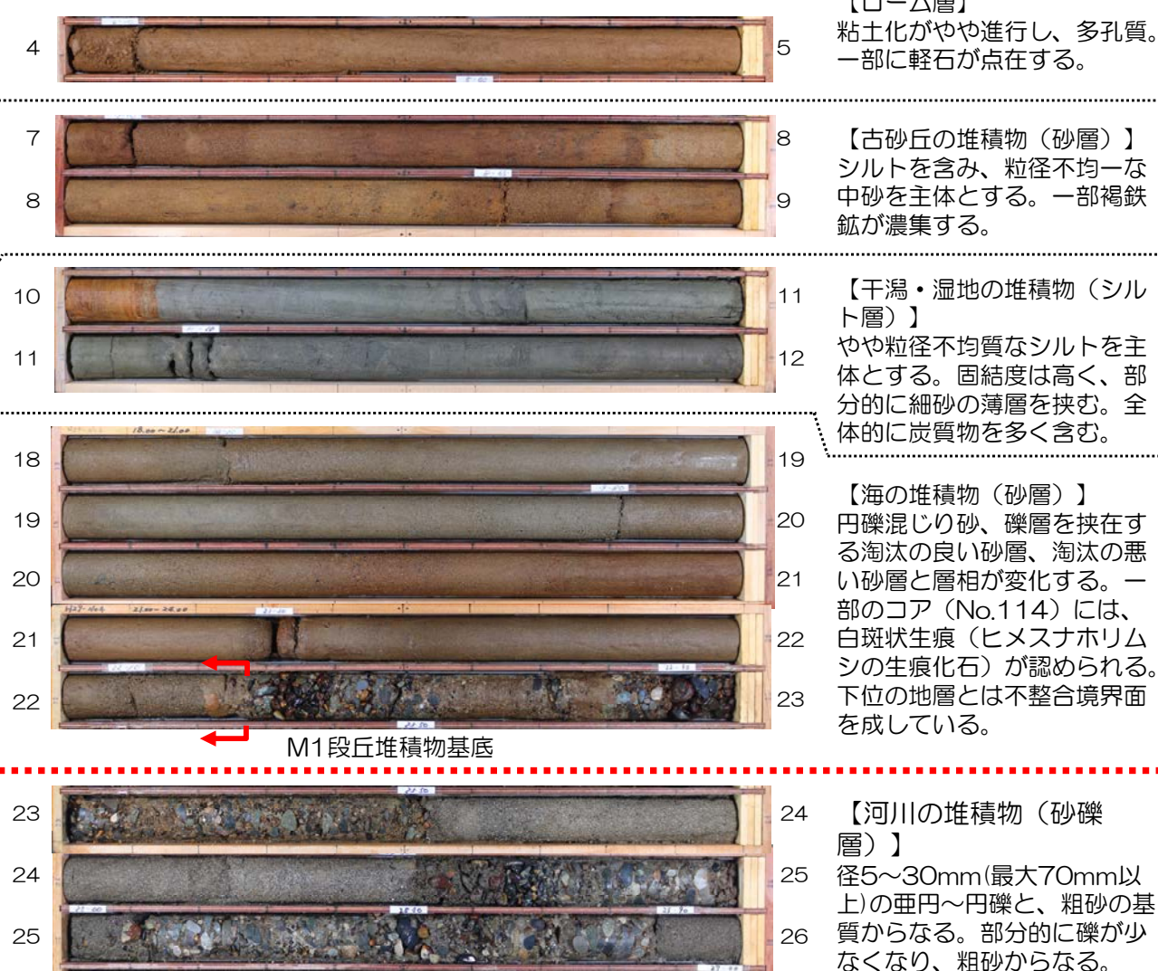
敷地内ボーリングコア写真 (No.116)
