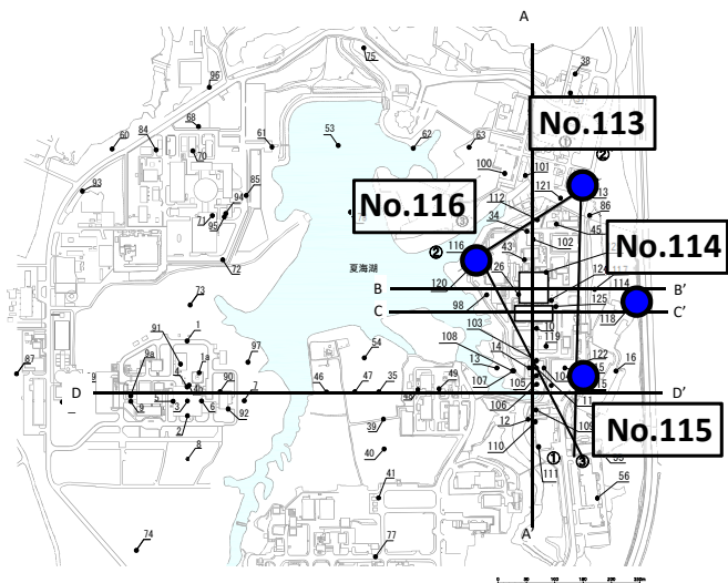
ボーリング位置図
