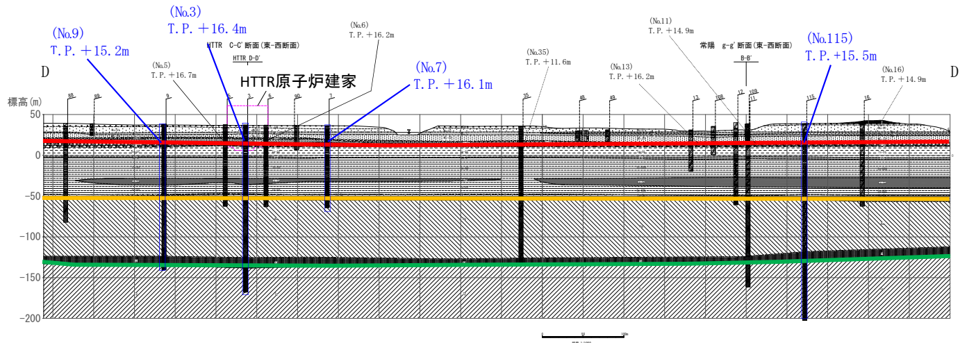
D-D' 測線（東西方向）
