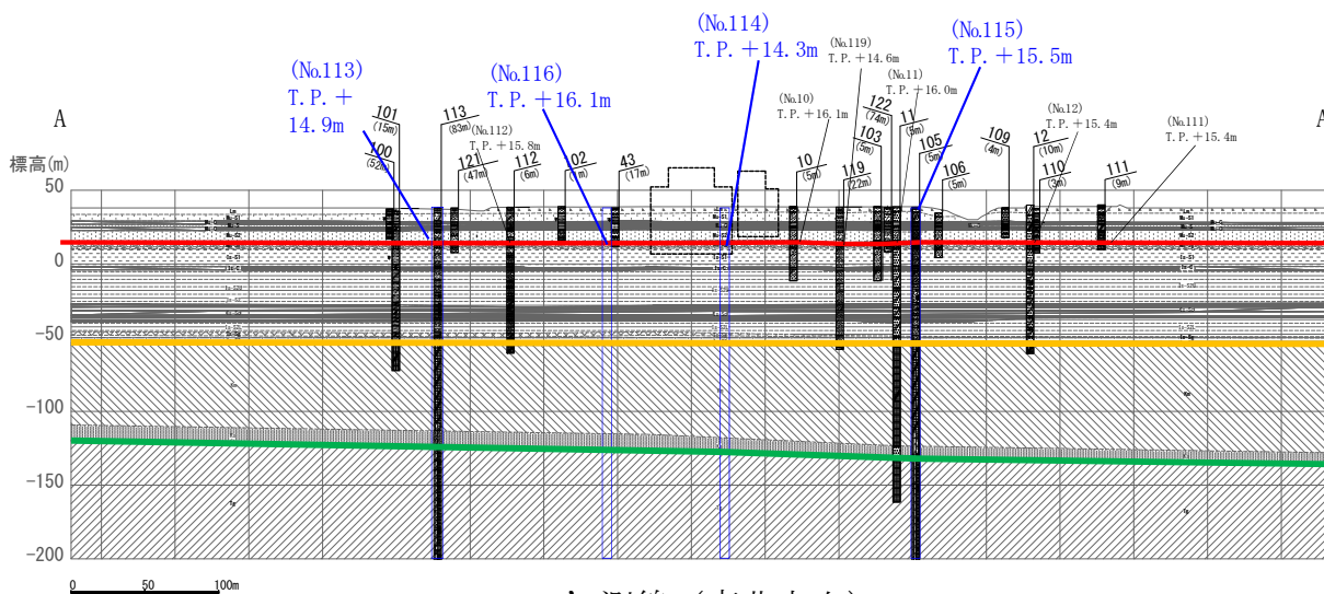
A-A' 測線 (南北方向)
