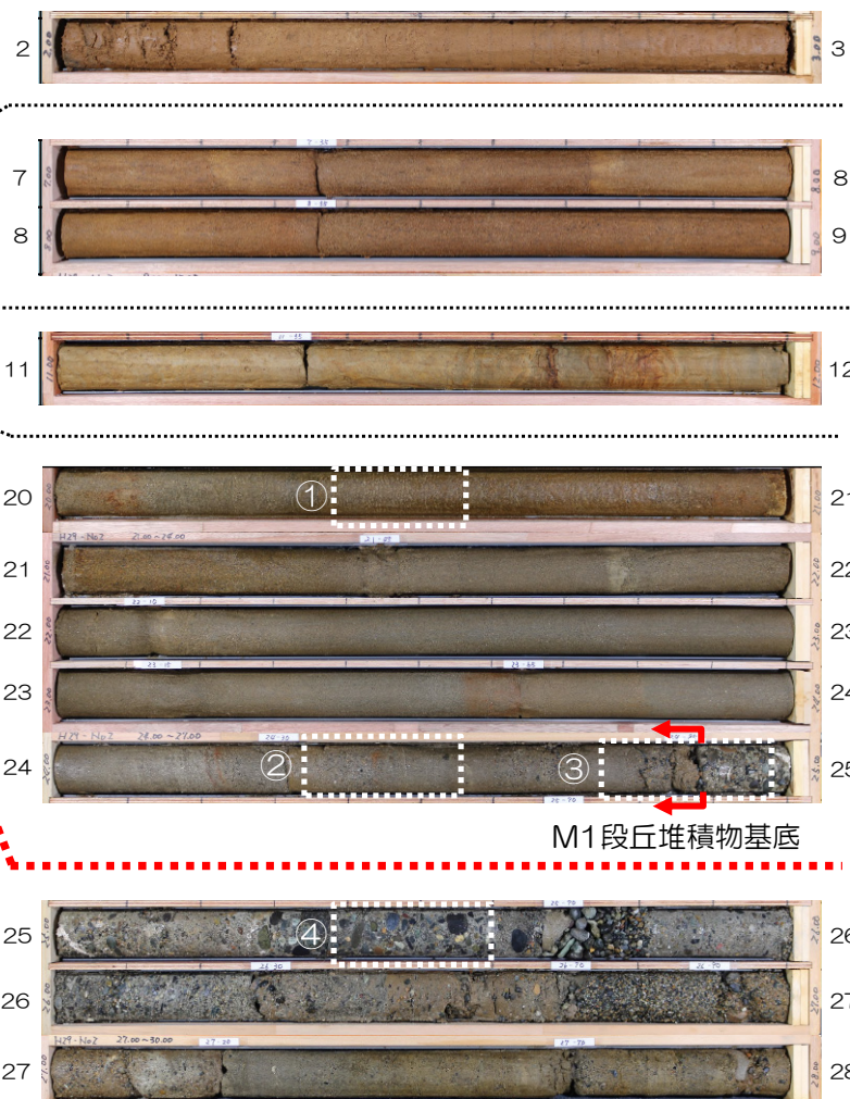
敷地内ボーリングコア写真 (No.114)
