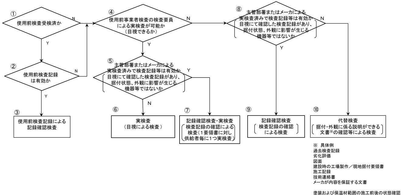
図9 据付・外観検査に対する運用を考慮した検査方法の選定フロー
