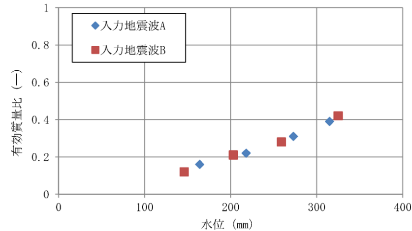
参考 3-2 図 入力地震動の加速度振幅及び周期特性の違いによる有効質量への影響
